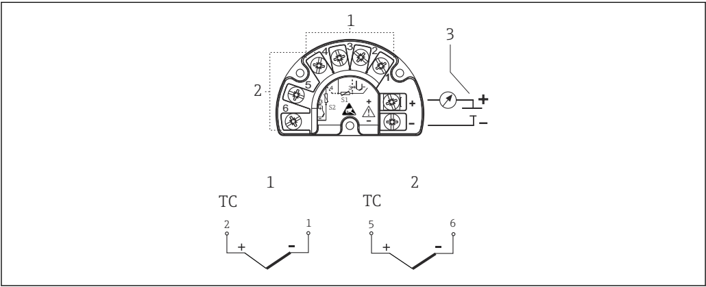
图 12 已安装 iTEMP TMT162 或 iTEMP TMT142B 现场型温度变送器
