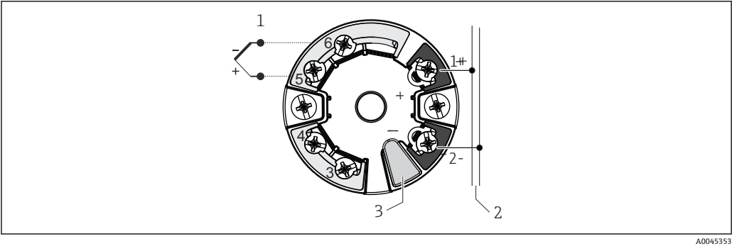
图 11 iTEMP TMT7x 或 iTEMP MT31 模块化温度变送器（单路传感器输入）
