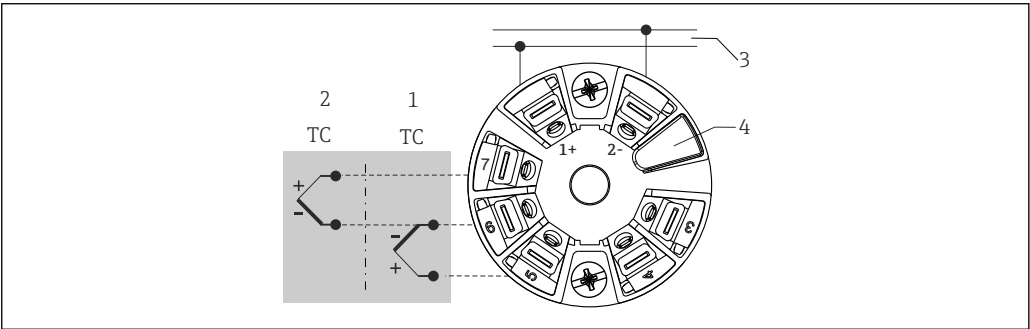
10 iTEMP TMT8x 模块化温度变送器 (两路传感器输入)
