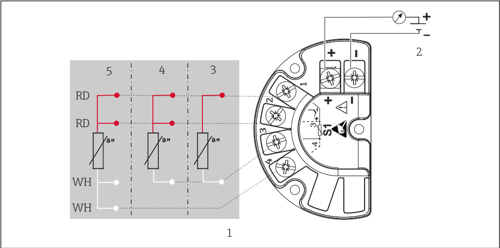
8 iTEMP TMT142B (单输入通道)
