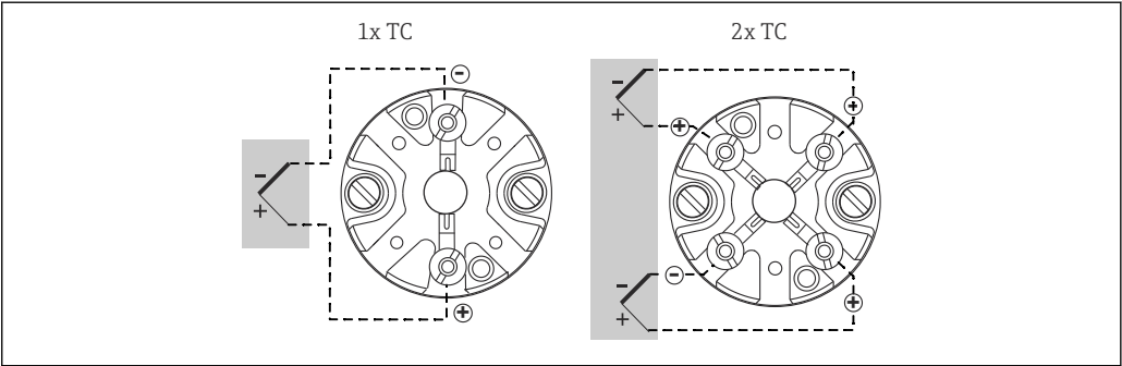
9 已安装的热电偶陶瓷端子接线块。
