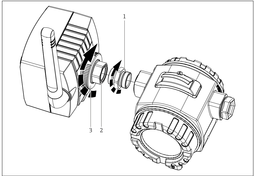
图 12 将 SWA70 安装在现场设备上（箭头尖端指向“闭合”方向。箭头末端指向“打开”方向）
