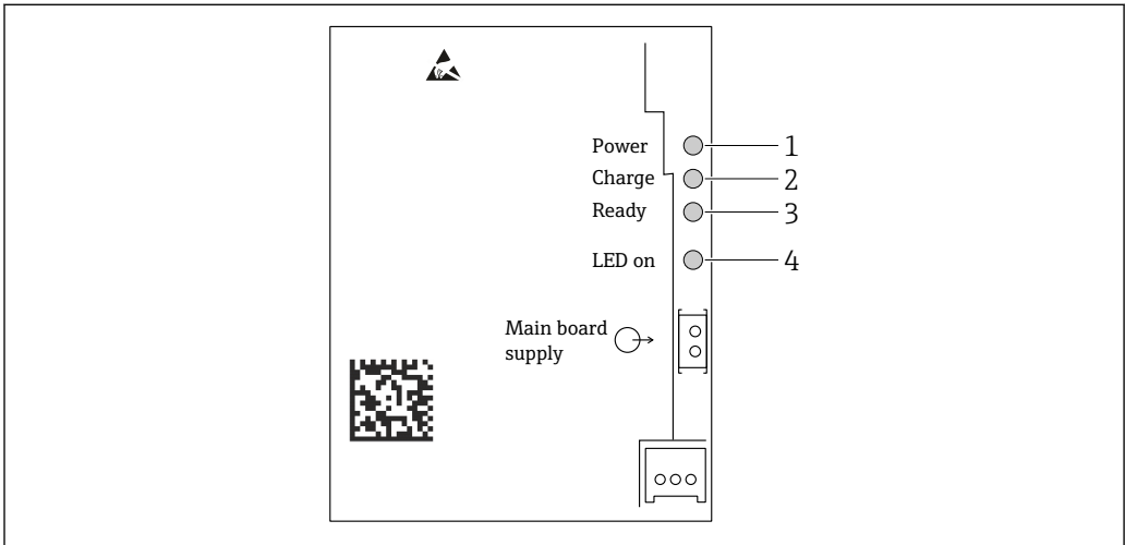
图 38 宽幅单元和直流供电单元上的显示和操作单元
