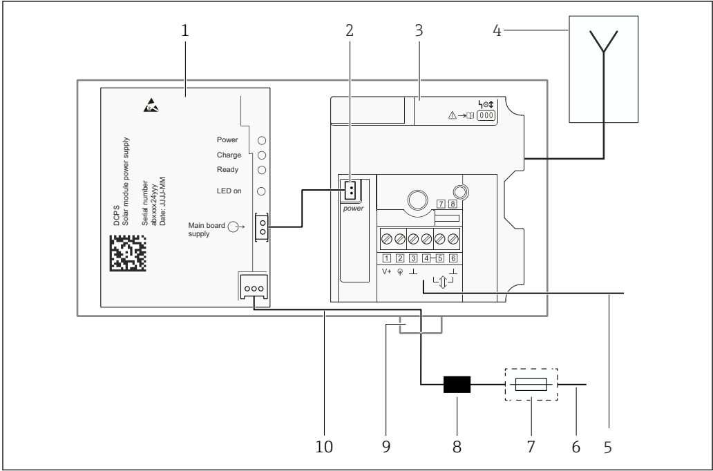
图 28 带直流供电单元的 SWA70 的电路框图
