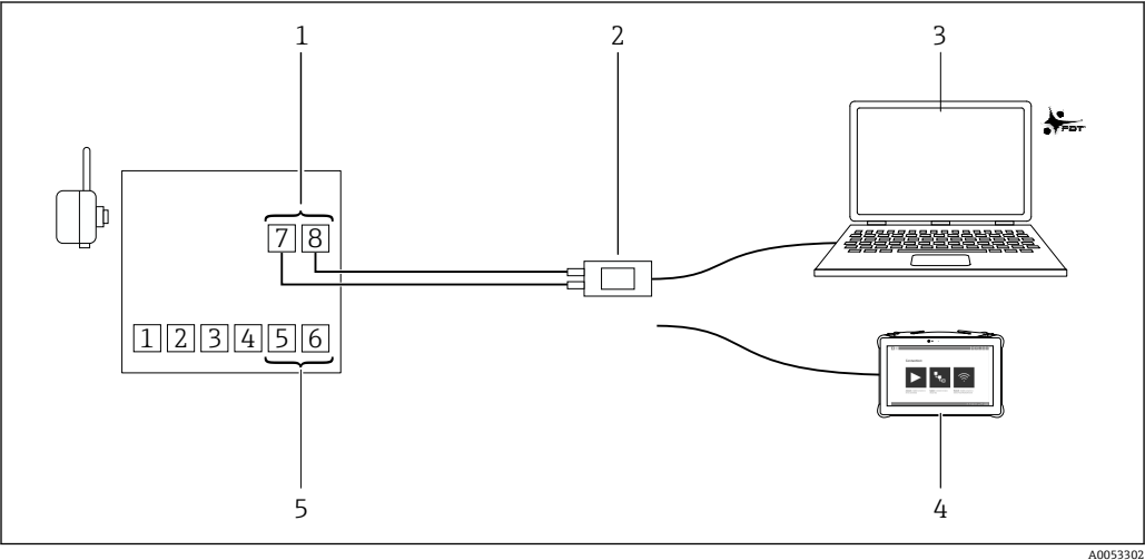
图 36 调制解调器连接示例：通过 Field Xpert SMTxx 或 FieldCare SFE500 进行 SWA70 的现场操作
