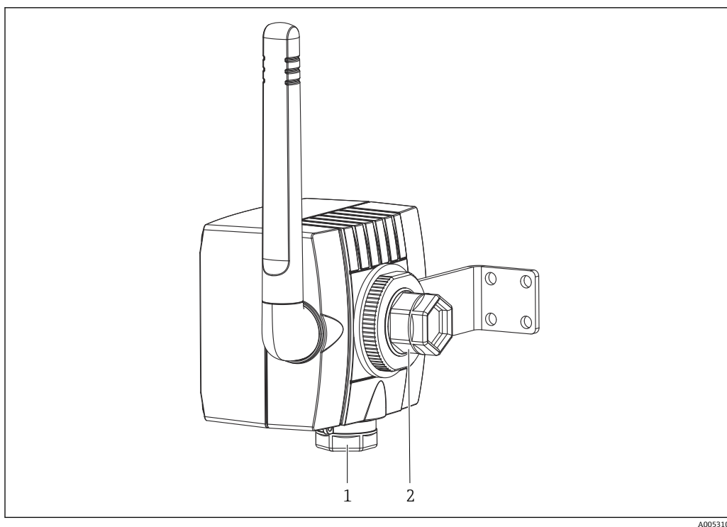
图 31 SWA70 上的电缆入口与“直流供电单元”型号搭配使用
