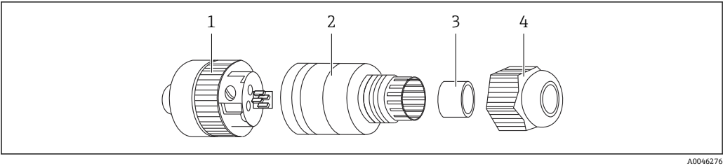
图 20 M12 插座
