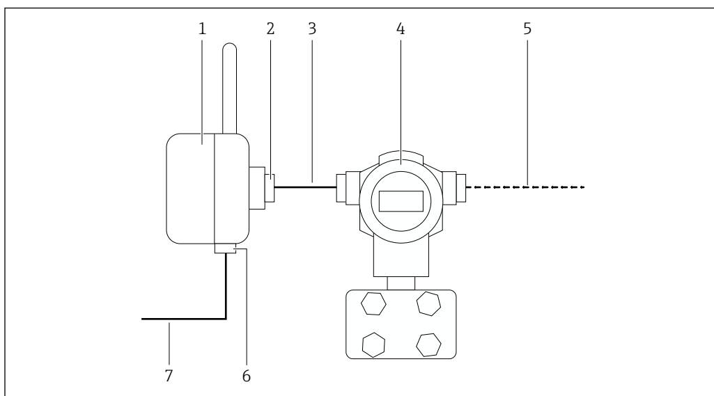
图 7 分体式安装带宽幅供电单元或直流供电单元的型号
