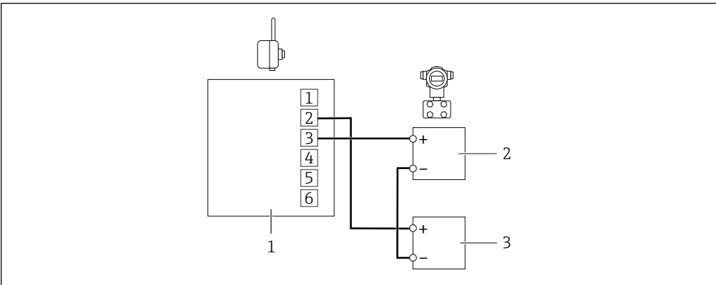
图 18 带电池组的 SWA70 – 不带通信电阻的闭环控制回路中的现场设备的连接
