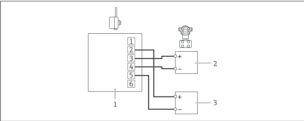
图 17 带电池组的 SWA70 – 不带通信电阻的两线制电缆闭环控制中的现场设备的连接
