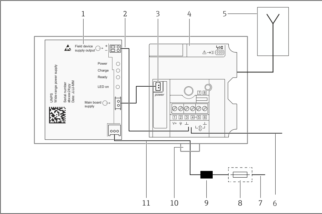
19 带宽幅供电单元的 SWA70 电路框图
