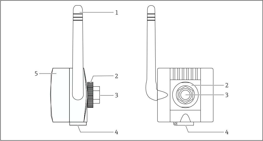
图 2 WirelessHART 适配器 SWA70 的结构设计
