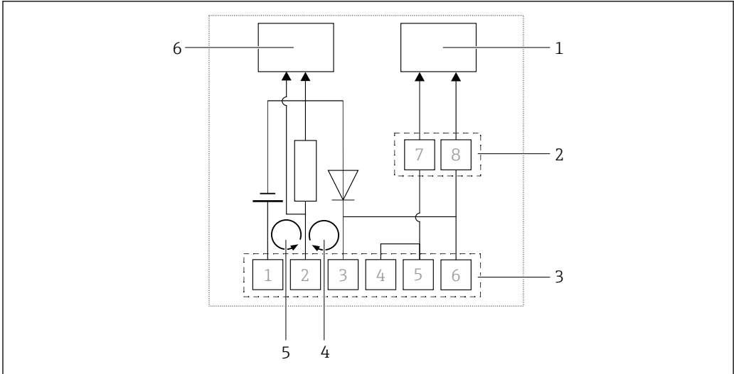
图 42 WirelessHART 适配器接线端子功能
