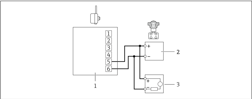
图 16 带电池组的 SWA70 – 带通信电阻的闭环控制中的现场设备的连接
