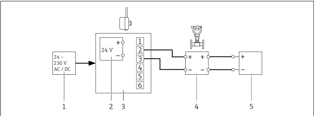
图 24 带宽幅供电单元的 SWA70 - 4/四线制现场设备的连接
