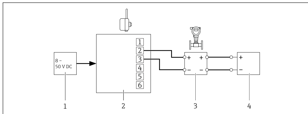
图 33 带直流供电单元的 SWA70 - 四线制现场设备的连接
