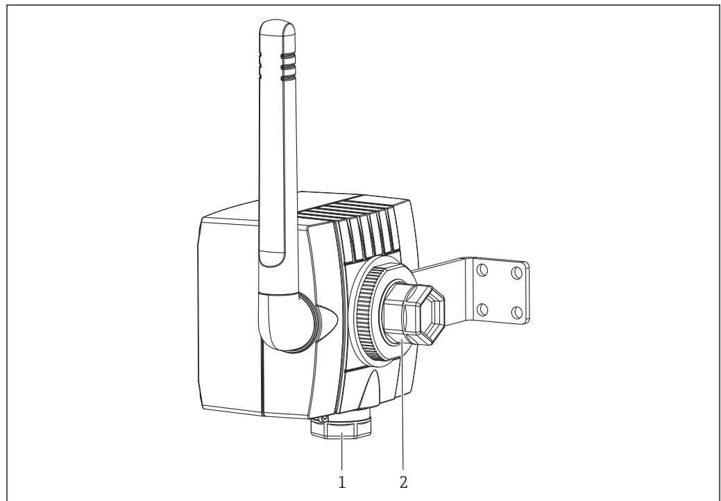
图 13 SWA70 上的电缆入口
