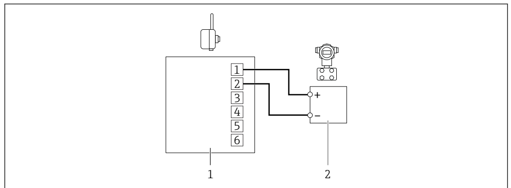
图 14 带电池组的 SWA70 - 连接由 SWA70 电池组供电的两线制现场设备
