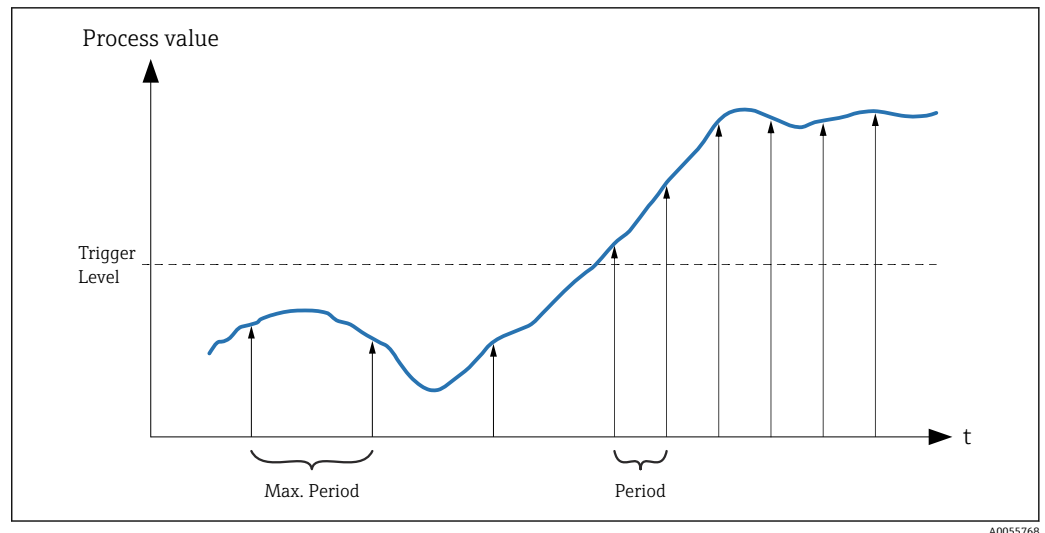
图 40 Trigger Mode 的示例: Raising
