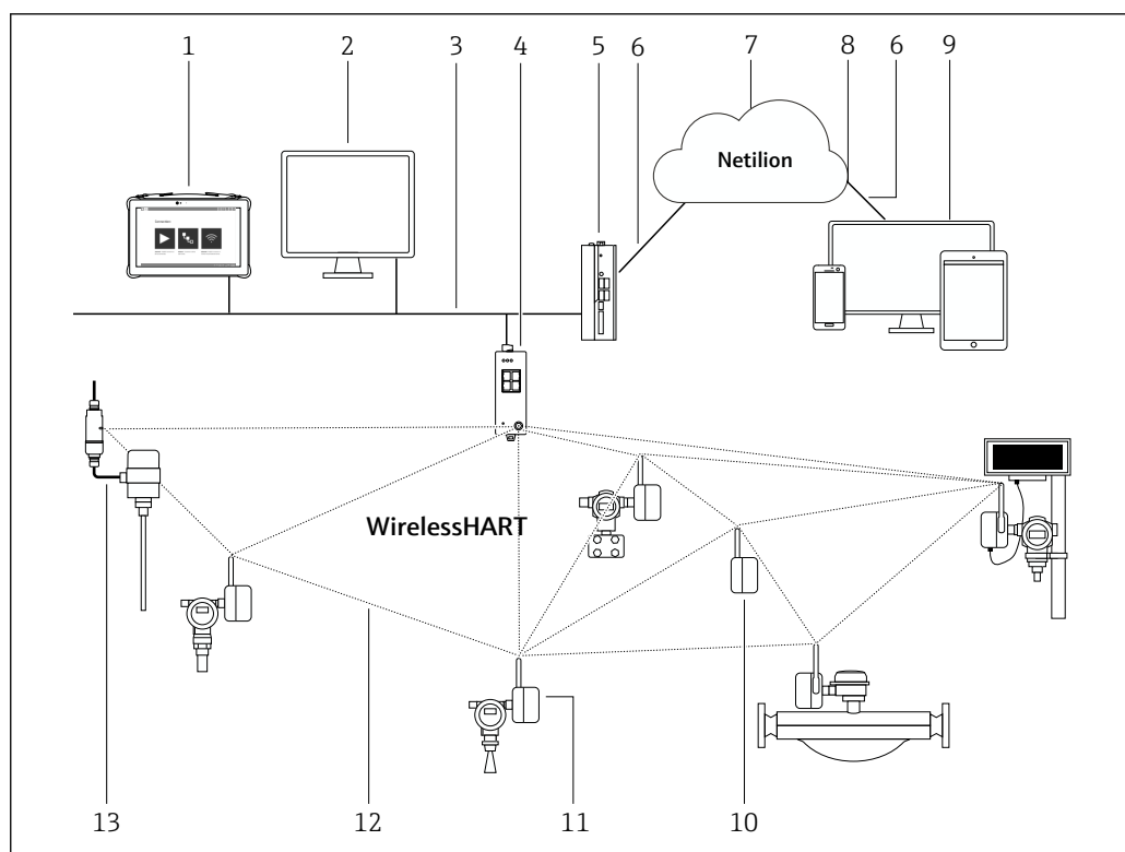
图 1 带 WirelessHART 适配器 SWA70 的 WirelessHART 网络架构示例
