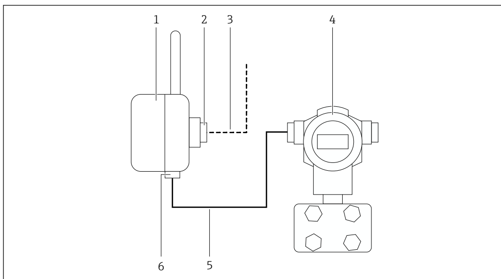
图 6 分体式安装带电池组的型号
