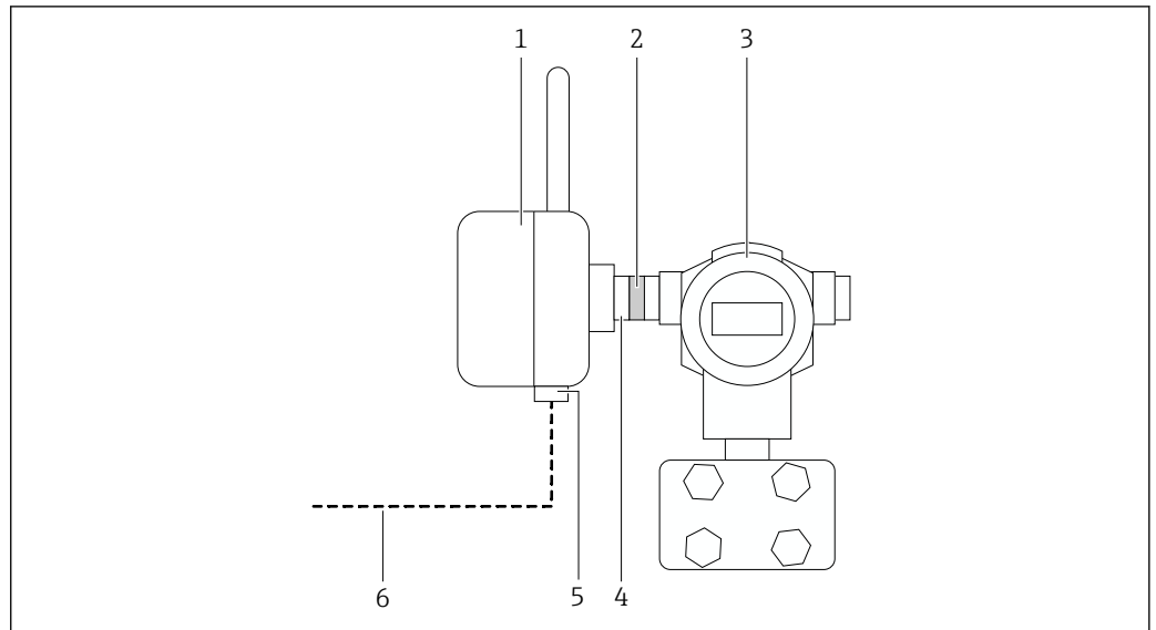
图 4 直接安装带电池组的型号
