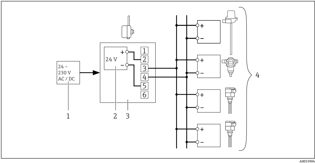
图 27 带宽幅供电单元的 SWA70 - Multidrop 模式下两线制现场设备的连接
