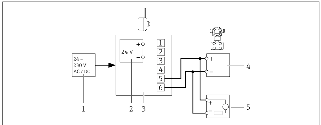
图 25 带宽幅供电单元的 SWA70 – 带通信电阻的闭环控制中的现场设备的连接
