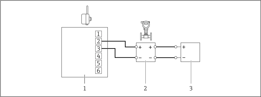
图 15 带电池组的 SWA70 – 连接一个四线制现场设备
