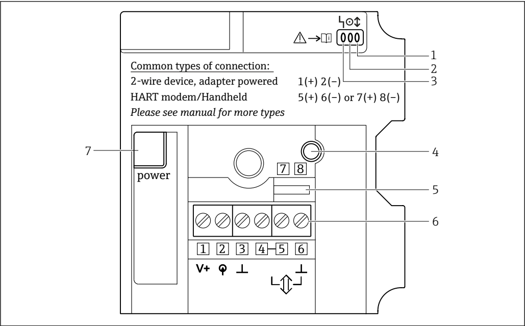
图 37 主电路板上的显示和操作部件
