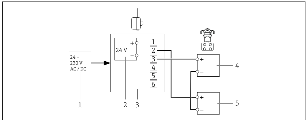
图 26 带宽幅供电单元的 SWA70 - 不带通信电阻的闭环控制中的现场设备的连接
