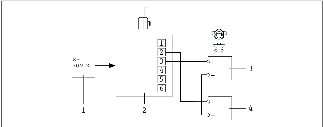
图 35 带直流供电单元的 SWA70 - 不带通信电阻的闭环控制中的现场设备的连接
