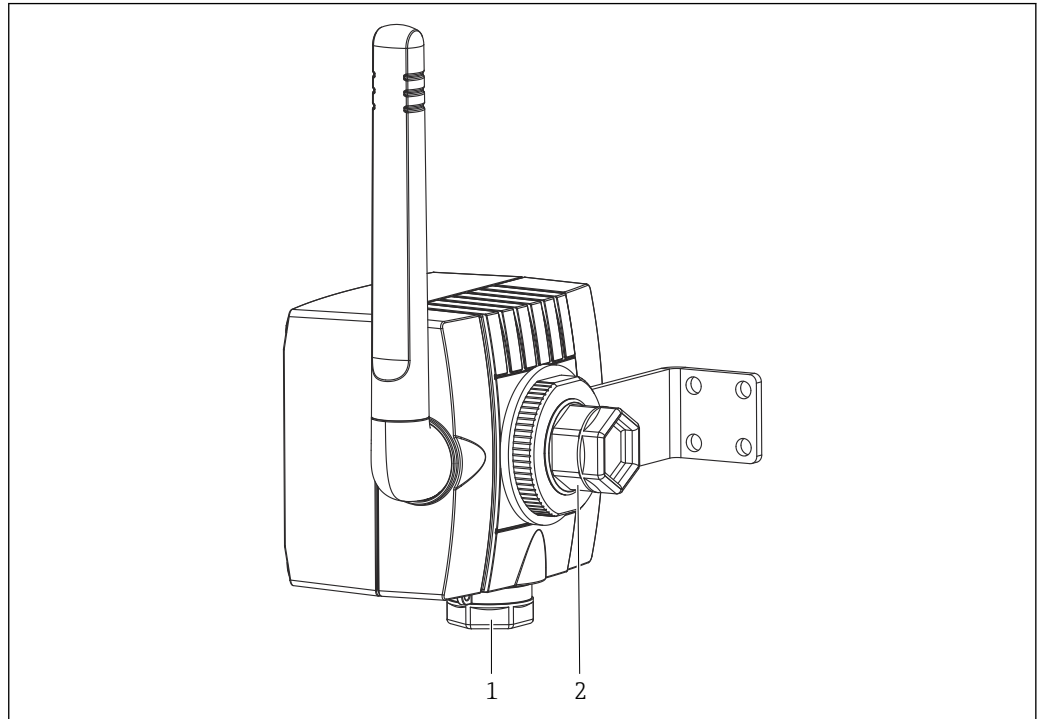
图 22 SWA70 上的电缆入口与“宽幅供电单元”型号搭配使用
