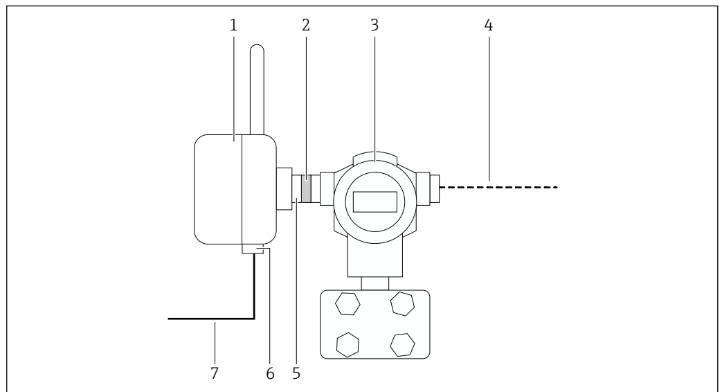
图 5 直接安装带宽幅供电单元或直流供电单元的型号
