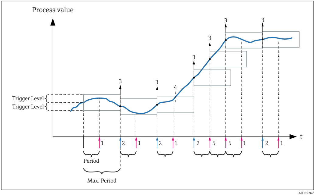
图 39 Trigger Mode 的示例: Window
