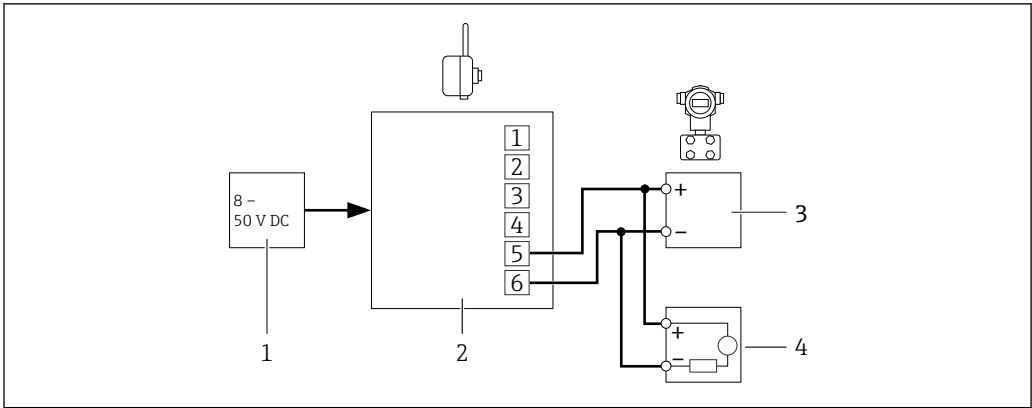
图 34 带直流供电单元的 SWA70 - 不带通信电阻的闭环控制中的现场设备的连接
