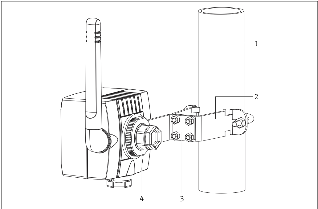
图 10 将 SWA70 安装在管道上，与现场设备分开
