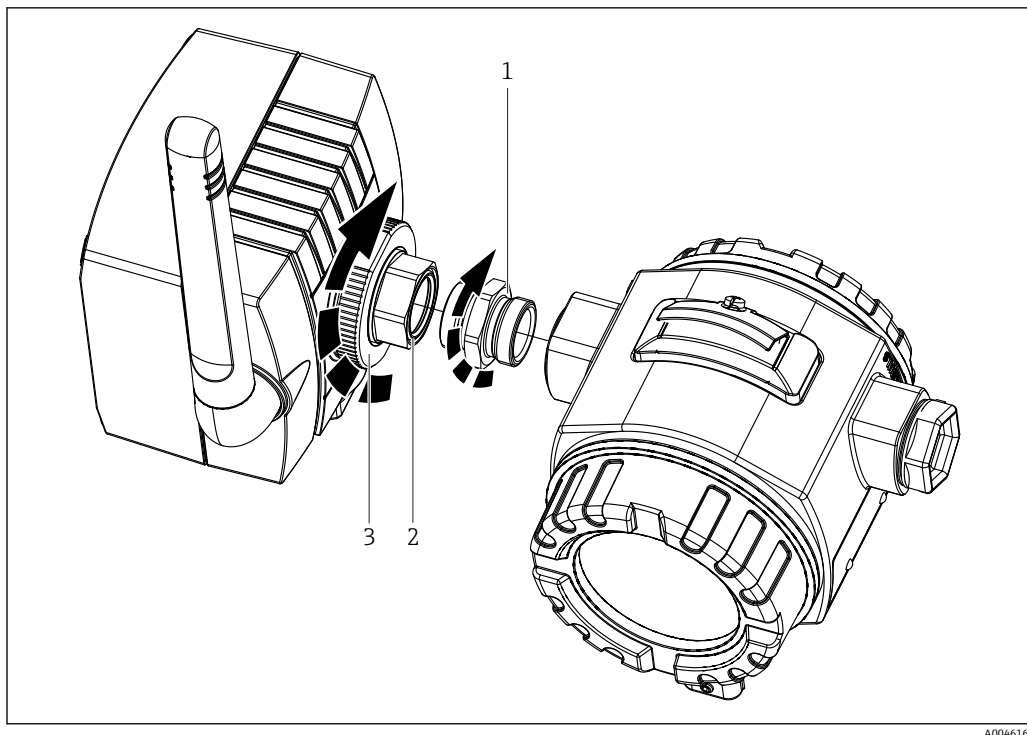
图 8 将 SWA70 安装在现场设备上（箭头尖端指向“闭合”方向。箭头末端指向“打开”方向）
