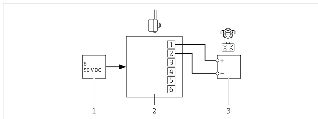
图 32 带直流供电单元的 SWA70 - 连接由 SWA70 直流供电单元供电的两线制现场设备
