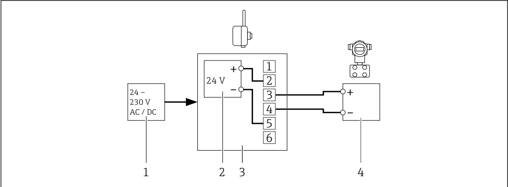
图 23 带宽幅供电单元的 SWA70 - 连接由 SWA70 宽幅供电单元供电的两线制现场设备
