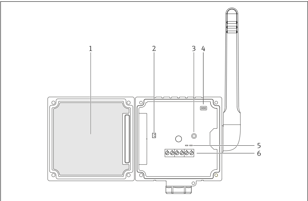
图 3 打开的 WirelessHART 适配器 SWA70
