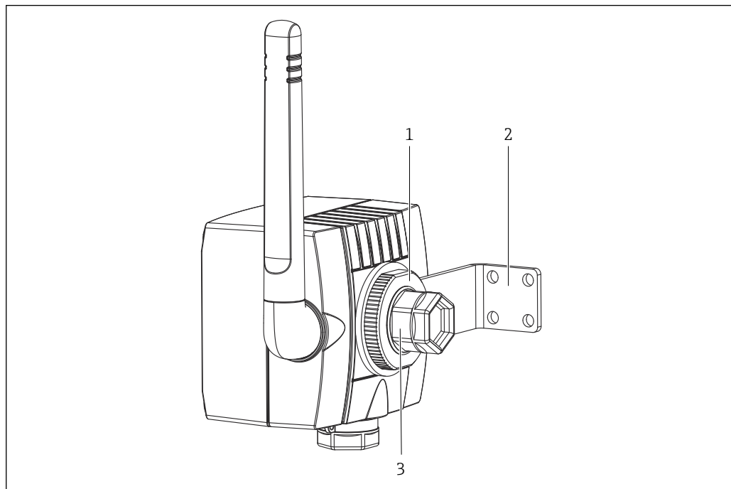
图 9 将 SWA70 安装在墙上，与现场设备分开
