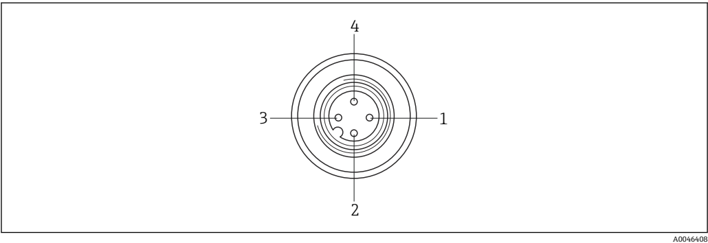
图 21 M12 插座的针脚分配
