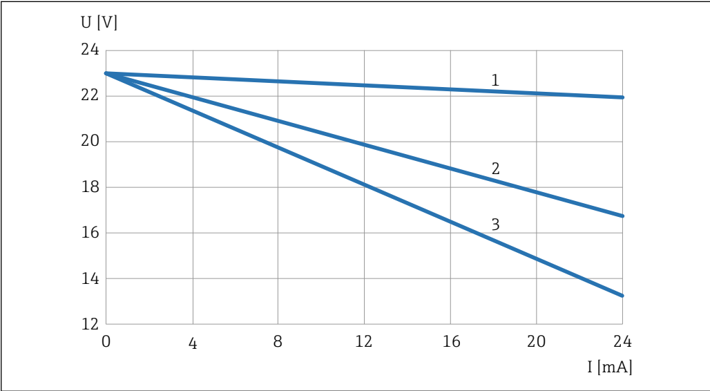
图 43 随回路电流变化的现场设备供电电压
