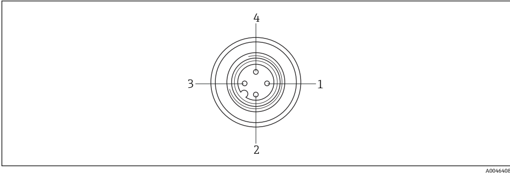
30 M12 插座的针脚分配
