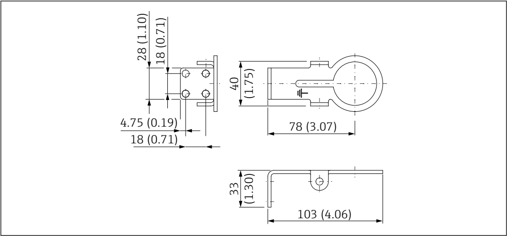
7 固定架的外形尺寸 - 墙装
