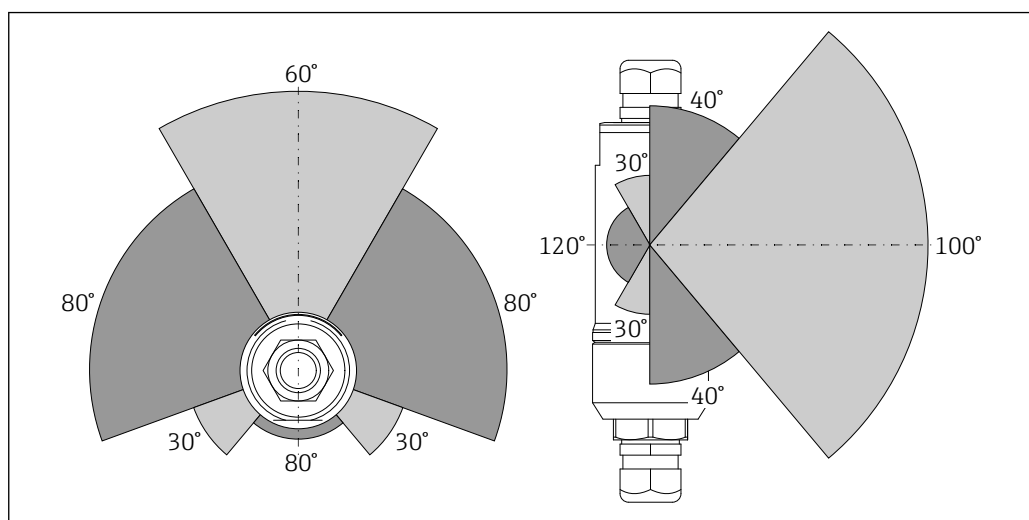
图 2 覆盖范围取决于传输窗口位置
