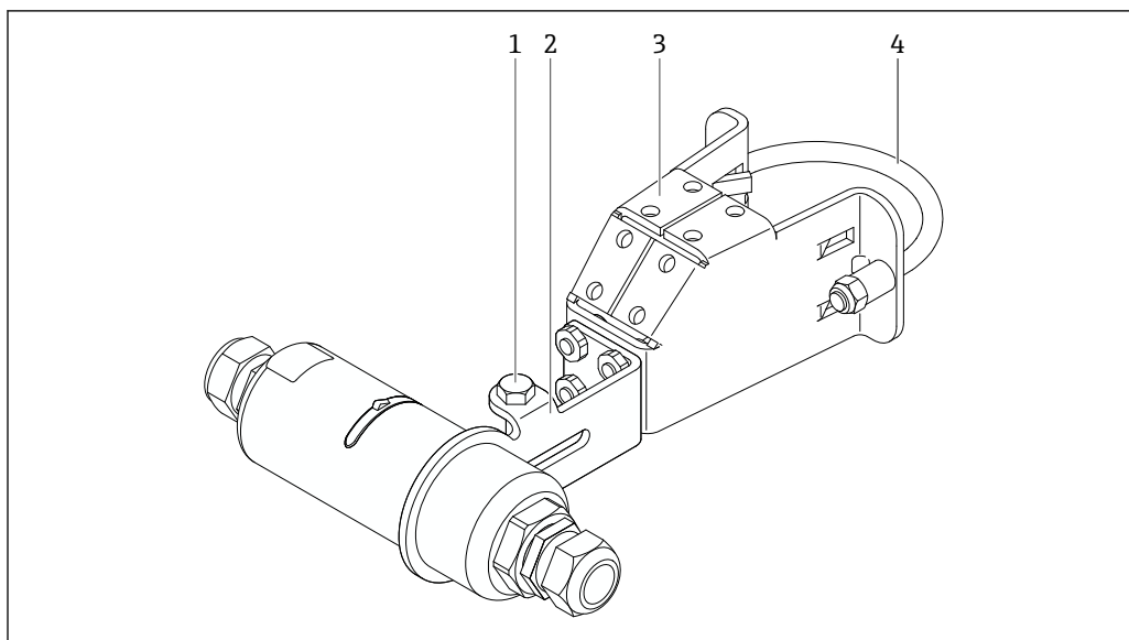
图 8 通过选装安装支架安装的 FieldPort SWA50
