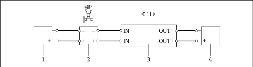
图 13 四线制 HART 现场设备（有源电流输出）的电气接线图（可选接地未显示） - OUT 接线端子连接 PLC 或变送器
