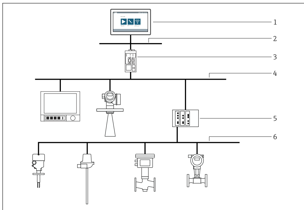
图 6 通过 Fieldgate SFG500 进行 PROFIBUS 点对点连接
