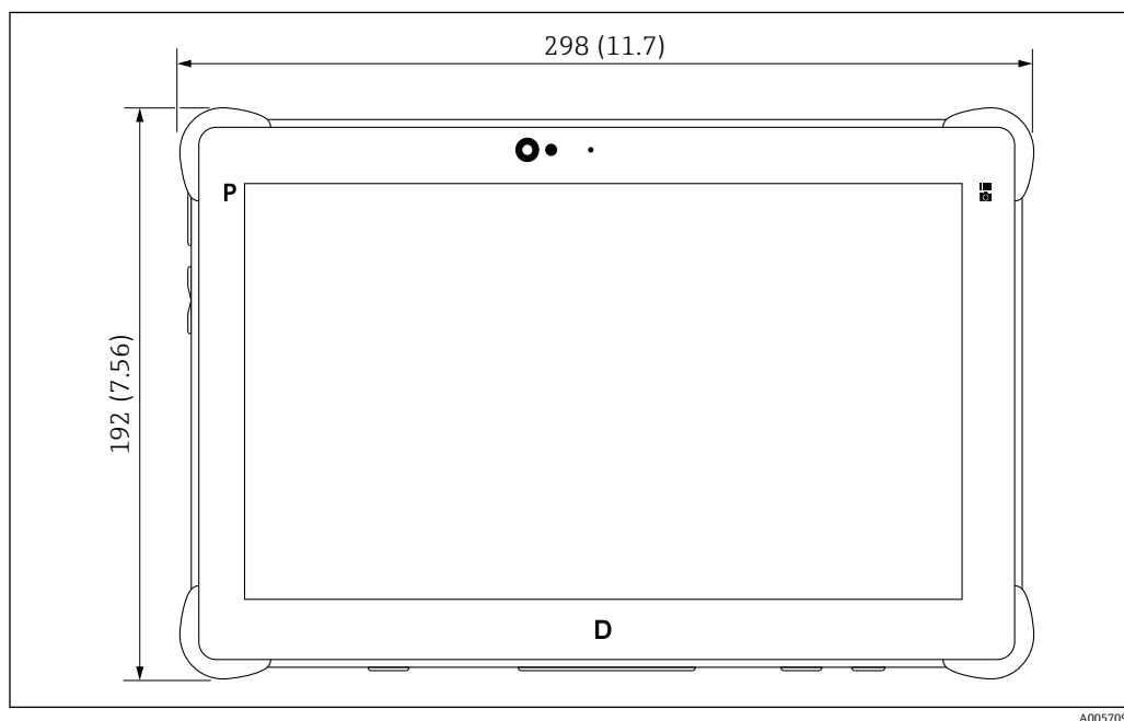
图 10 正视图。测量单位 mm (in)
