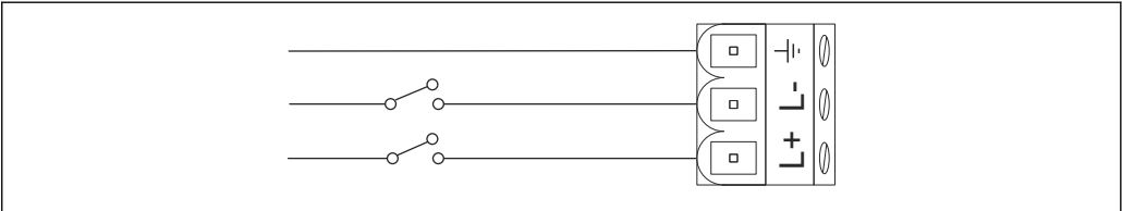
图 11 电流输入接线图
