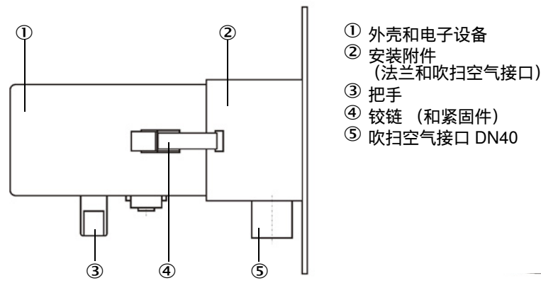
图 5: 发收单元 DUSTHUNTER SB30
