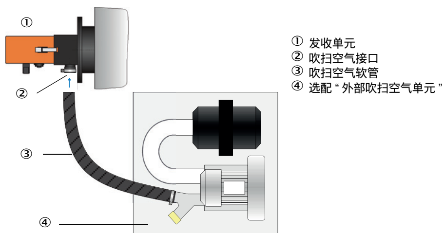
图 18: 把吹扫空气单元连接到收发单元上
