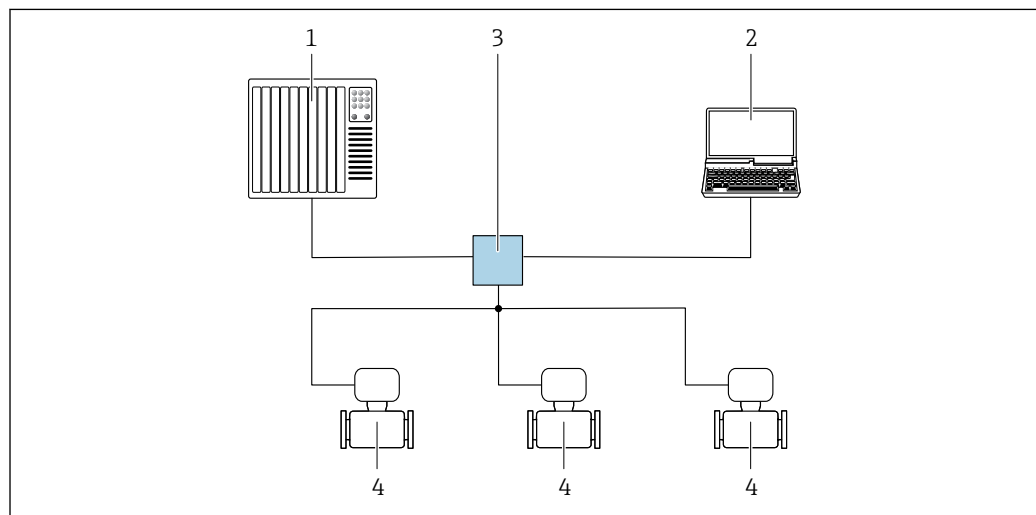
图 58 通过 PROFINET 网络进行远程操作：星形拓扑结构
