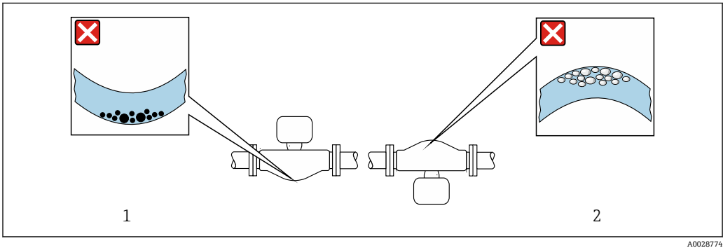
☒ 14 弯测量管传感器的安装方向
