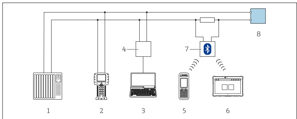
图 50 通过 HART 通信进行远程操作（有源信号）
