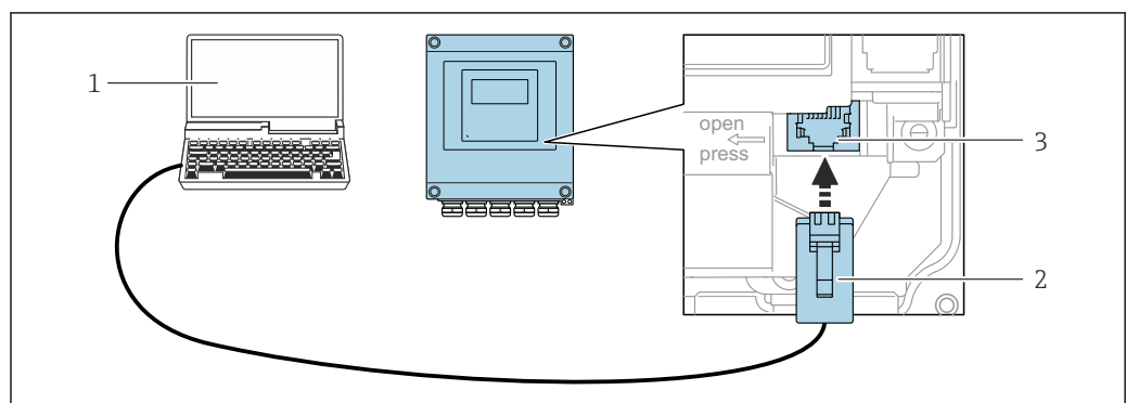
图 62 通过服务接口（CDI-RJ45）连接
