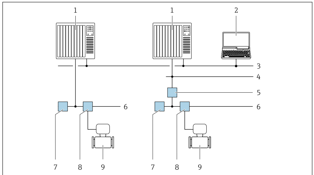
图 52 通过 FOUNDATION Fieldbus 网络进行远程操作
