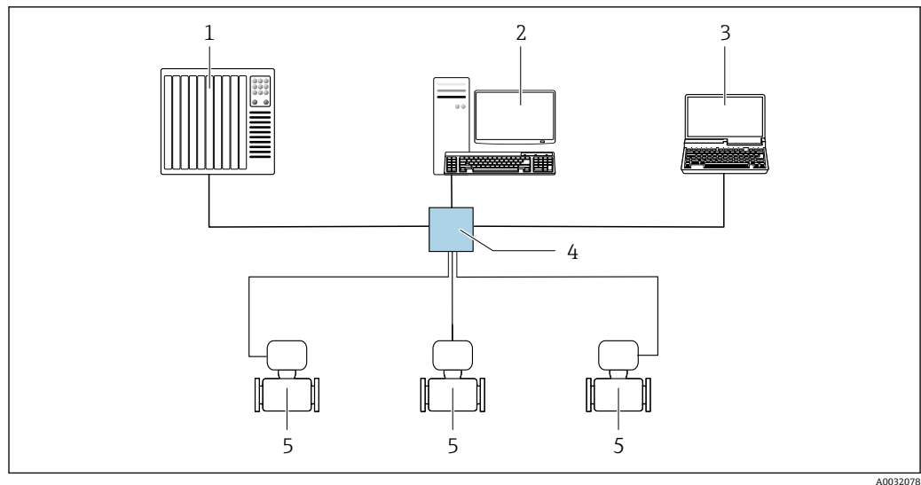
图 61 通过 Modbus TCP + Ethernet 进行远程操作 - 100 Mbit/s: 星形拓扑结构
