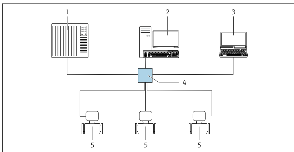
图 56 通过 EtherNet/IP 网络进行远程操作：星形拓扑结构
