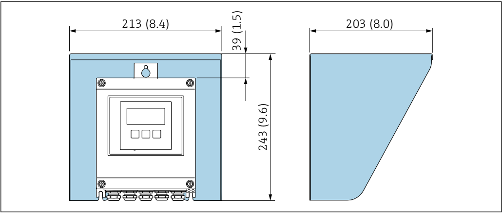
35 Proline 500（数字）变送器的防护罩；单位：mm (in)
