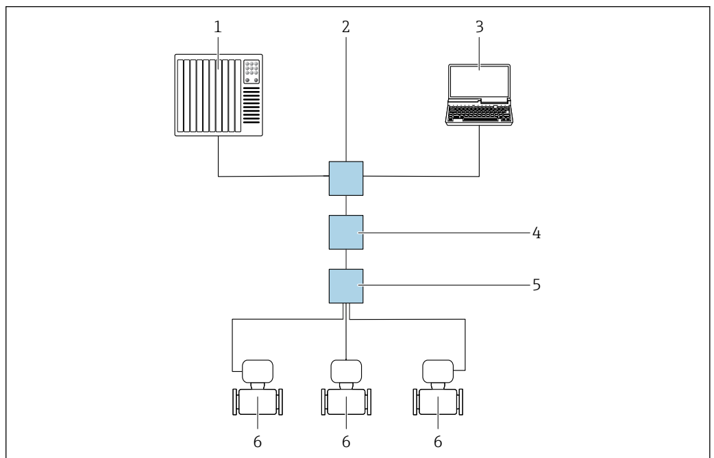
图 60 通过 Modbus TCP + Ethernet-APL 通信进行远程操作（有源信号）
