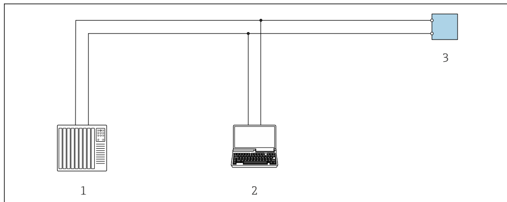
图 55 通过 Modbus RS485 通信进行远程操作（有源信号）
