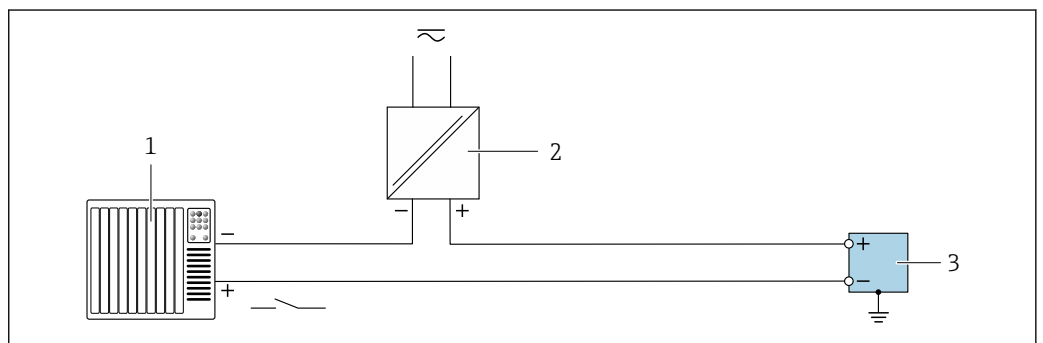
图 8 状态输入
