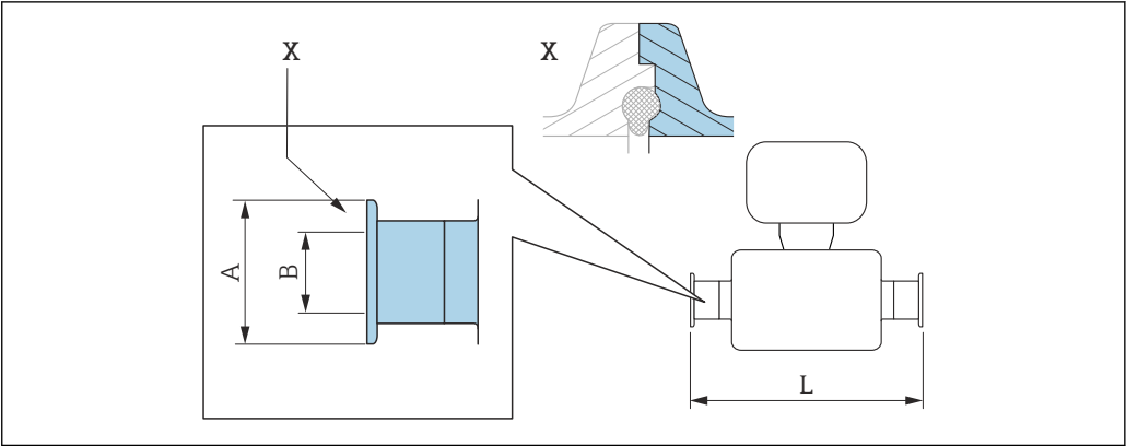
28 部件 X: 非对称过程连接; 蓝色部分由供应商提供。
