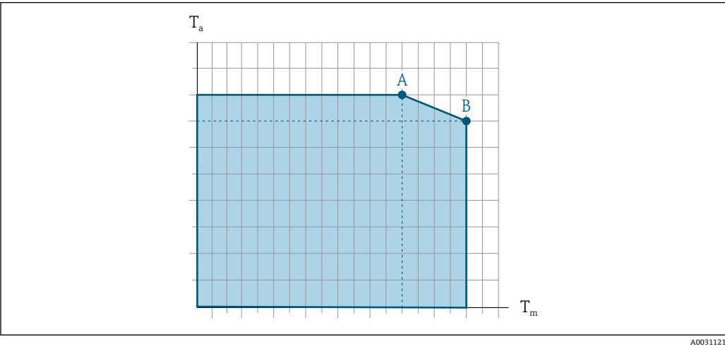
36 示例图，具体数值见下表。 T a 环境温度 T m 介质温度 A 介质温度 T m 越高 (T a max = 60 °C (140 °F)时)，所需的环境温度 T a 越低 B 传感器最高允许介质温度 T m 对应的最高允许环境温度 T a
