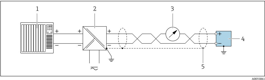
19 接线实例：4 ... 20 mA HART 电流输出（无源） 1 自动化系统，带 4 ... 20 mA HART 电流输入（例如 PLC） 2 电源 3 选配显示单元：注意最大负载 4 变送器，带 4 ... 20 mA HART 电流输出（无源） 5 电缆屏蔽层单端接地。如需确保安装符合 NAMUR NE 89 标准，电缆屏蔽层必须两端接地。
