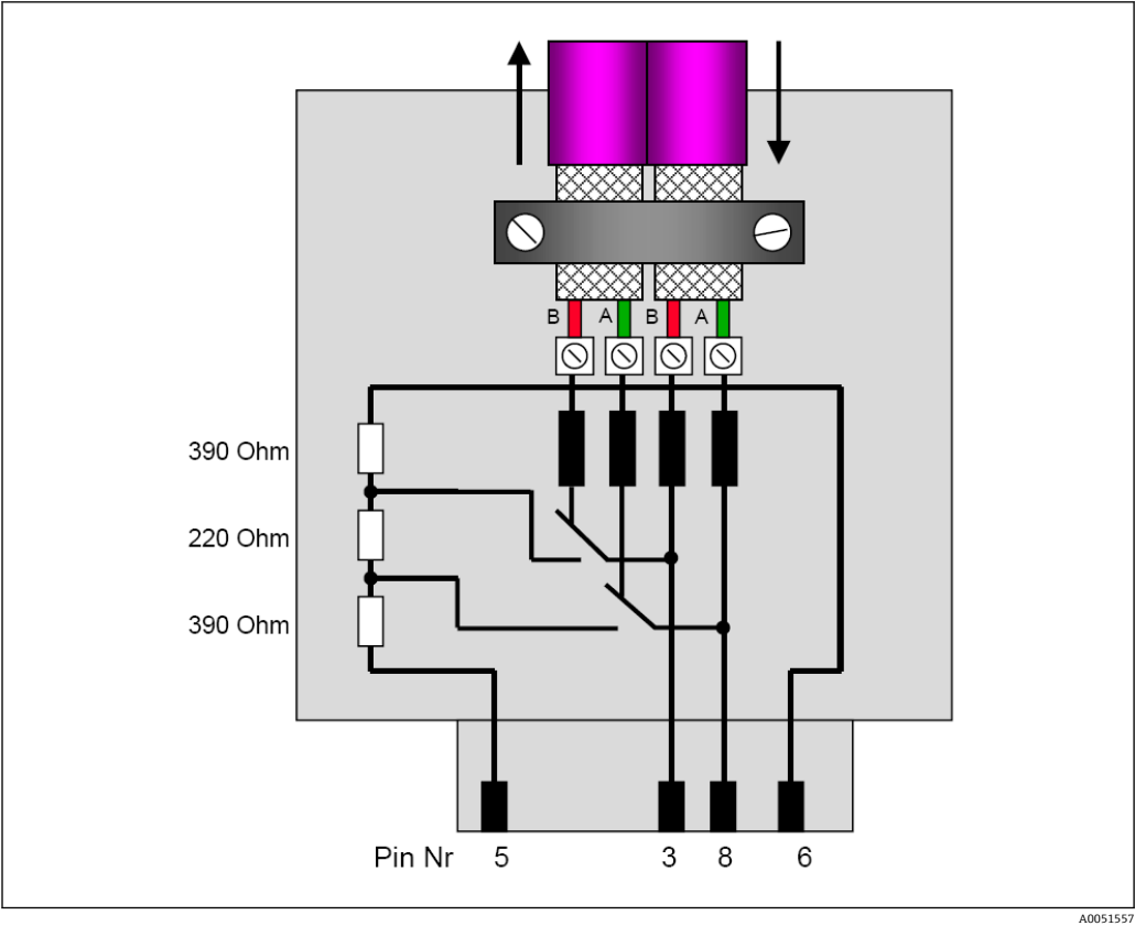
图 2 PROFIBUS 接头中的终端电阻
