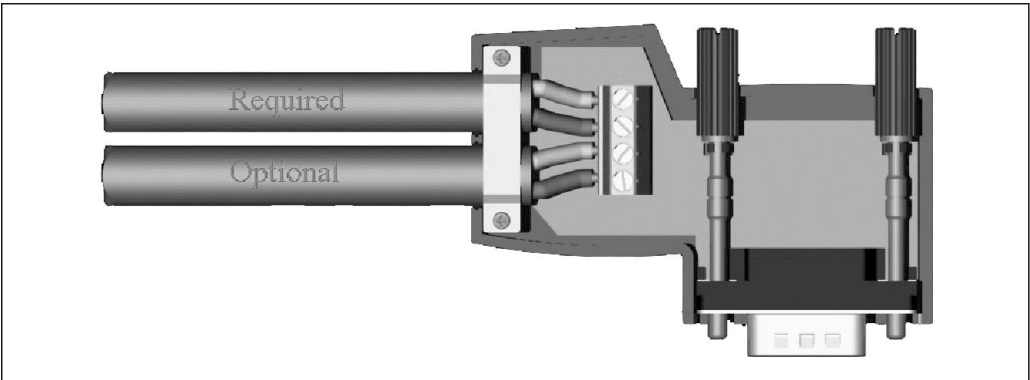
1 符合 IEC 61158/EN 50170 标准的 PROFIBUS 连接头
