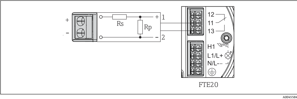
21 电阻回路，用于监测线路状态（短路和断路）
