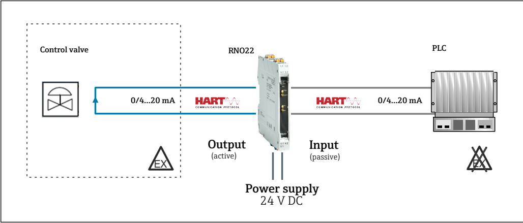
22 在防爆危险区使用 RNO22 输出隔离信号放大器促动控制阀
