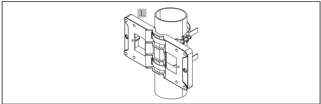
图 13: 管装准备
