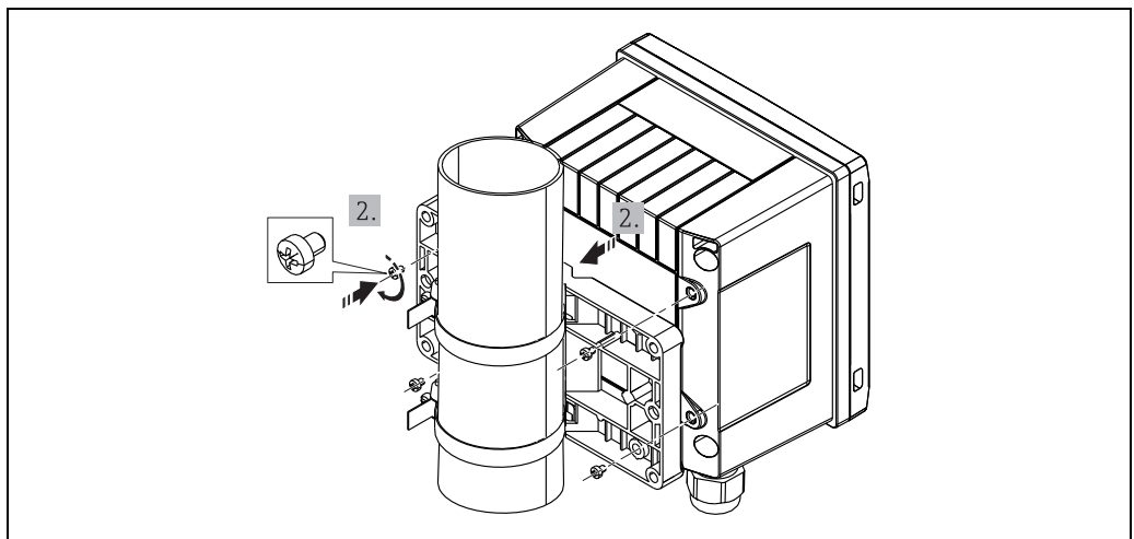
图 14: 管装
