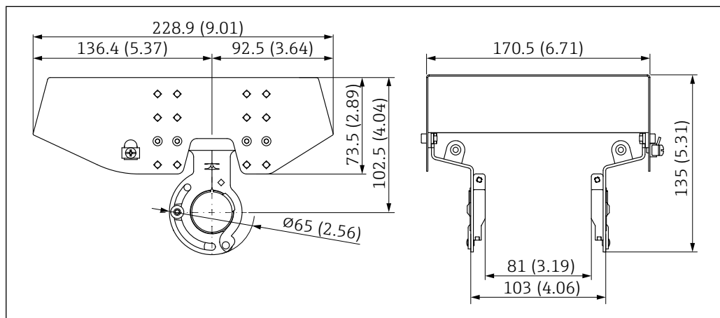
图 22 316L 防护罩 XW112 的外形尺寸示意图。测量单位 mm (in)
