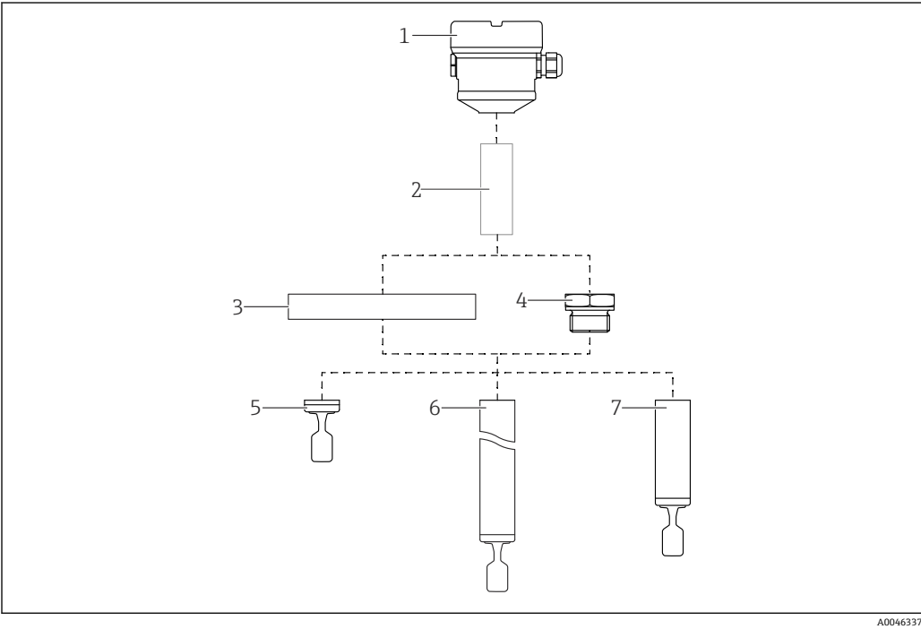
图 2 产品设计: Liquiphant FTL51B 1 外壳，安装有电子插件 FEL60D 和外壳盖 2 选配隔热管，气密馈通（第二道防护） 3 法兰过程连接（选配） 4 螺纹过程连接（选配） 5 一体型探头，带音叉 6 延长管型探头，带音叉 7 短管型探头，带音叉
