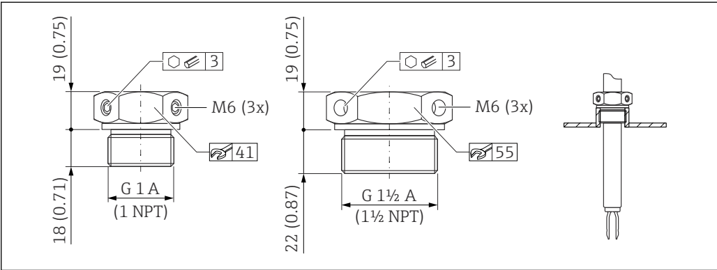
25 常压滑动套管 p_e = 0 \text{ bar} (0 psi)。测量单位 mm (in)
