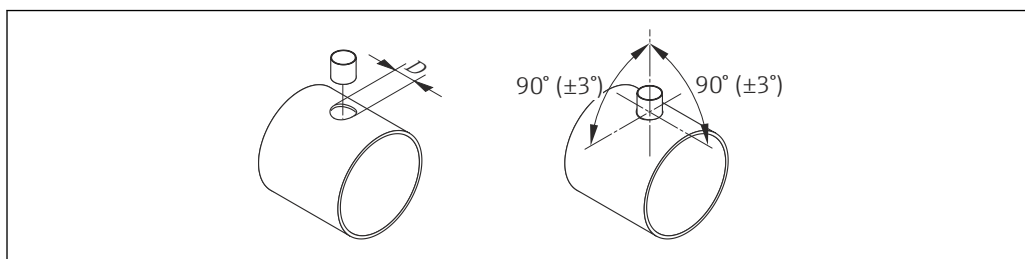
图 4 安装螺母和 threadolets 的安装条件
