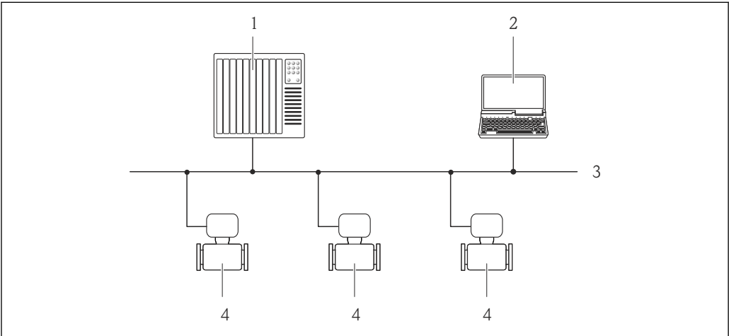
图 19 通过 PROFIBUS DP 网络进行远程操作 1 自动化系统 2 带 PROFIBUS 网卡的计算机 3 PROFIBUS DP 网络 4 测量设备
