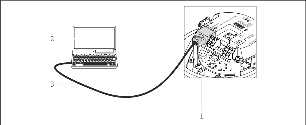
图 20 订购选项“输出”，选型代号 L: PROFIBUS DP 1 测量设备的服务接口 (CDI-RJ45)，内置 Web 服务器访问接口 2 计算机，带 Web 浏览器 (例如：互联网浏览器)，用于访问内置设备 Web 服务器；或安装有“FieldCare”调试工具，带 COM DTM “CDI 通信 TCP/IP” 互联网浏览器)，用于访问内置设备 Web 服务器；或安装有“FieldCare”调试工具，带 COM DTM “CDI 通信 TCP/IP” 3 标准以太网连接电缆，带 RJ45 插头
