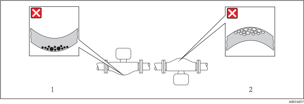
图 4 带弯测量管的传感器安装方向示意图 1 测量含固流体时，请避免此安装方向：存在固体积聚的风险 2 测量除气流体时，请避免此安装方向：存在气体积聚的风险
