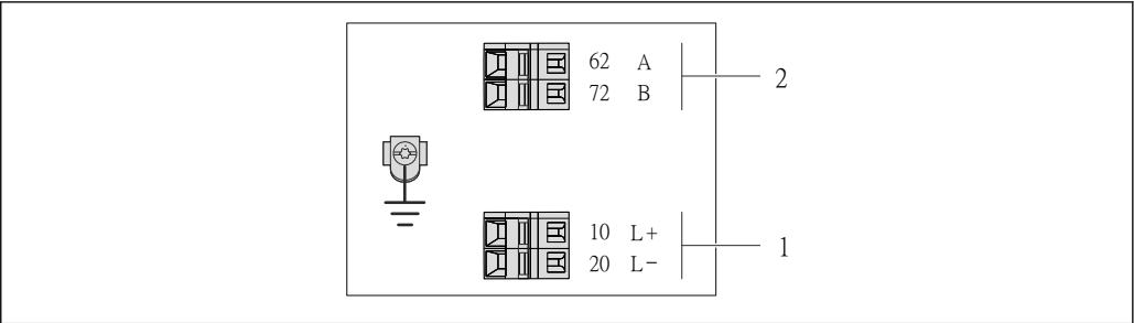
7 Modbus RS485 型仪表的接线端子分配示意图，连接类型适用于在本安防爆场合中使用(通过 Promass 100 安全栅连接)
