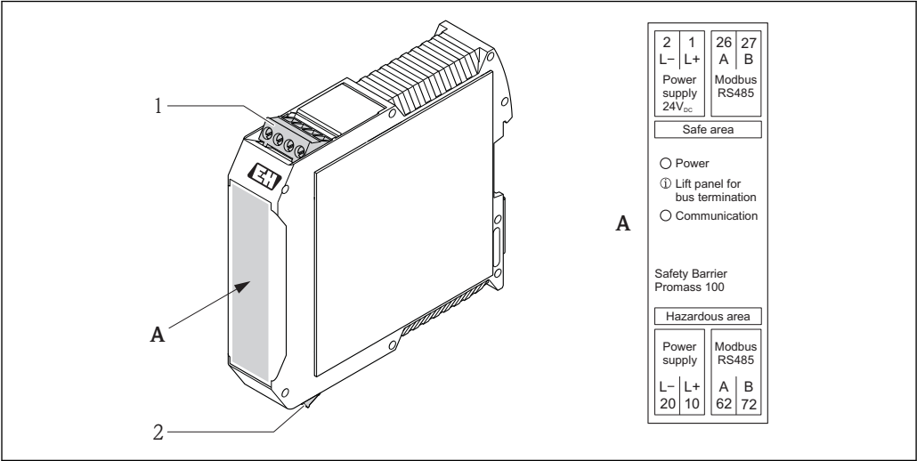
8 Promass 100 安全栅和接线端子示意图
