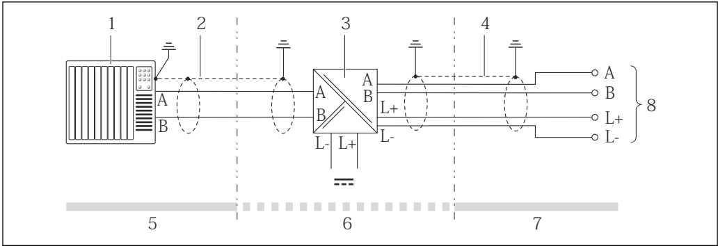
11 变送器和 Promass 100 安全栅间的电气连接
