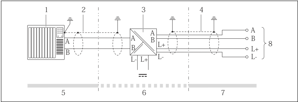
12 本安型 Modbus RS485 的连接示例
