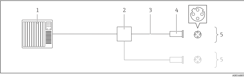
图 8 工业以太网(EtherNet/IP)的连接示例
