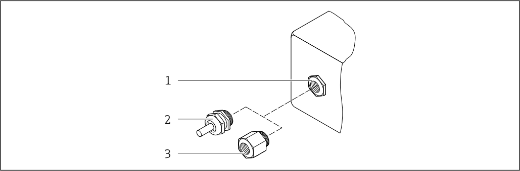
图 22 允许的电缆入口/缆塞 1 M20 × 1.5 内螺纹 2 M20 × 1.5 缆塞 3 转接头，适用 G ½"或 NPT ½"内螺纹电缆入口
