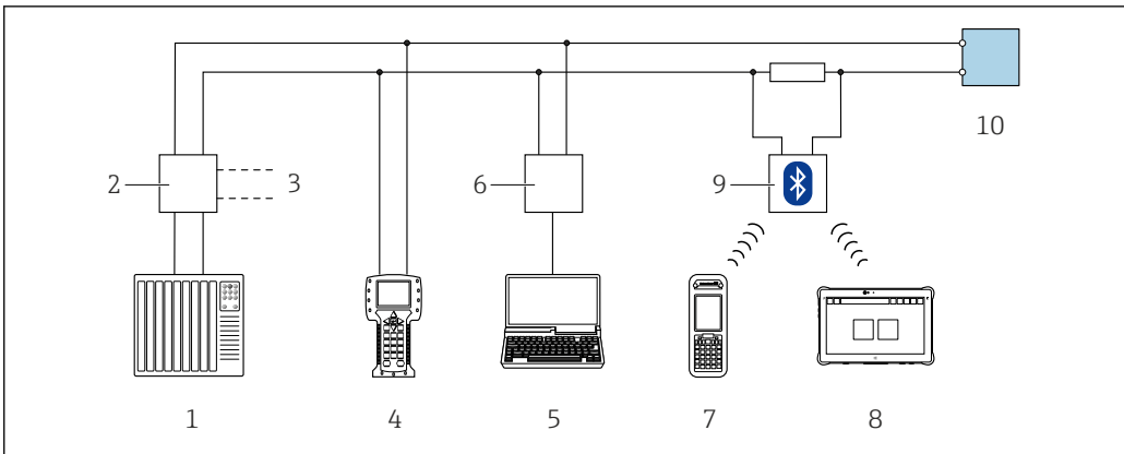
图 12 通过 HART 通信进行远程操作（无源信号）
