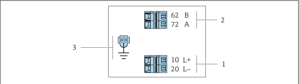
图 9 接线端子分配: Modbus RS485, 在本安防爆区中使用 (通过 Promass 100 安全栅连接) 1 本安型电源 2 Modbus RS485 3 电缆屏蔽层 (IO 信号) 连接端 (如有) 和/或电源保护性接地端 (如有)。不适用选型代号 C “超紧凑一体型, 不锈钢; 卫生型”。
