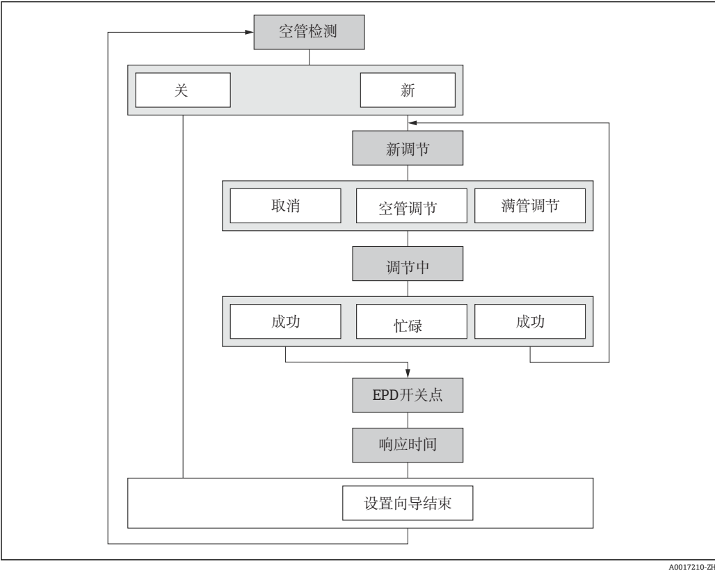
图 27 “空管检测” 向导，“设置” 菜单中
