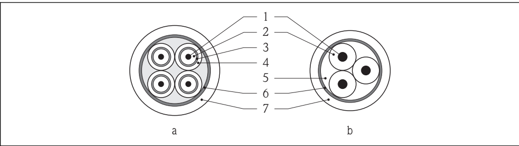
9 电缆横截面示意图
