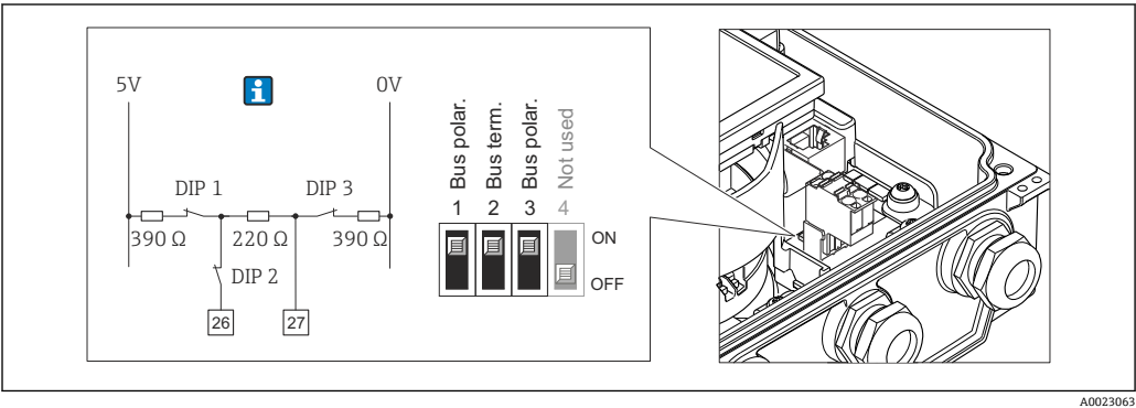
图 19 通过主要电子模块上的 DIP 开关开启终端电阻
