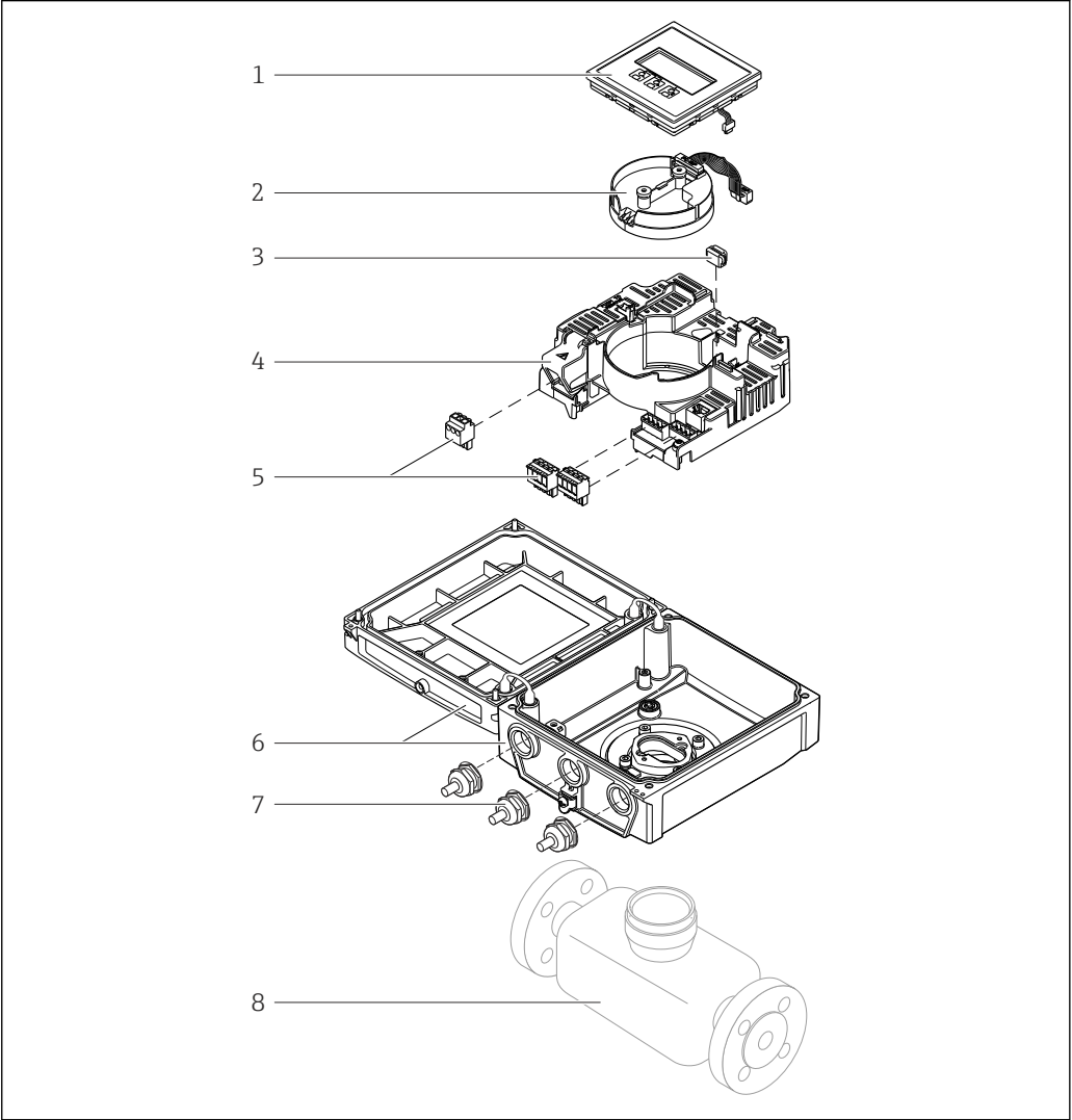
图 1 一体式仪表的重要部件
