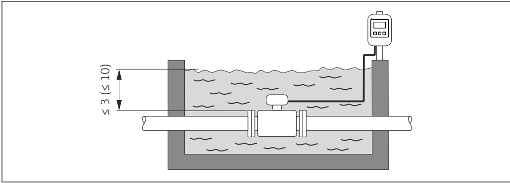
图 6 单位: m (ft)
