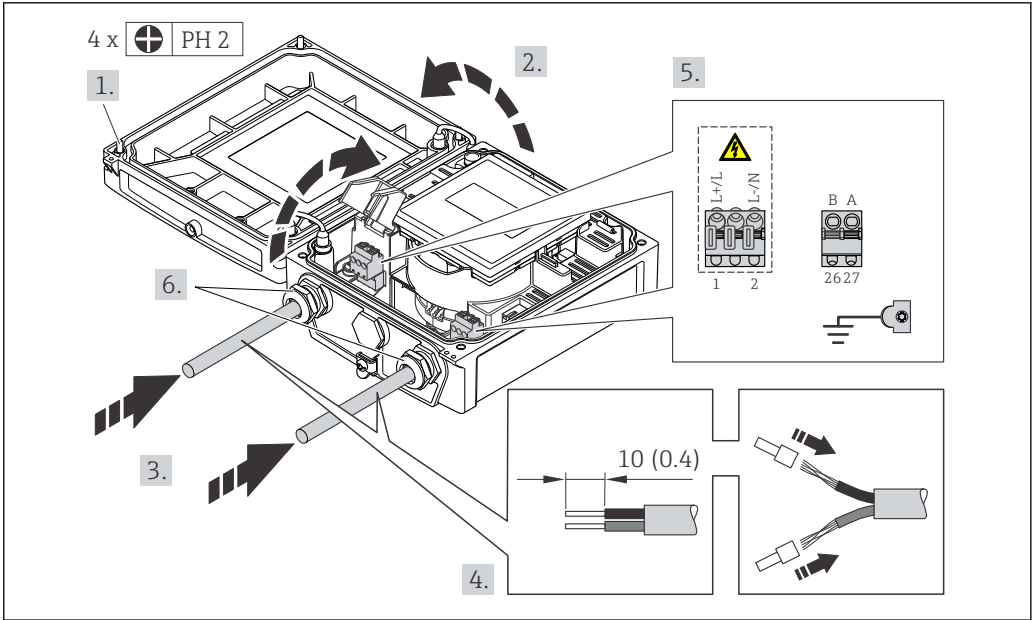
15 连接供电电压和 Modbus RS485
