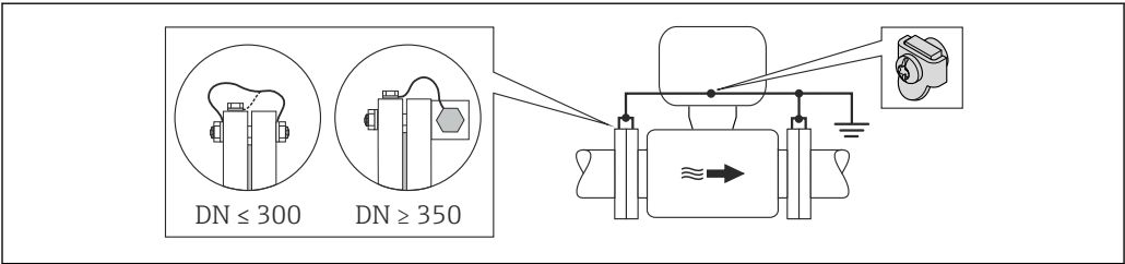
图 17 通过接地端子和管道法兰实现系统电势平衡
