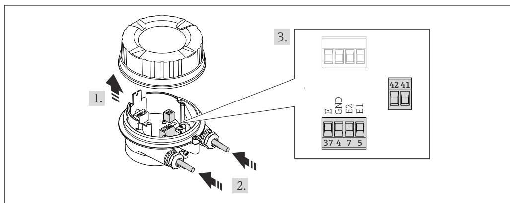
图 14 传感器：连接模块
