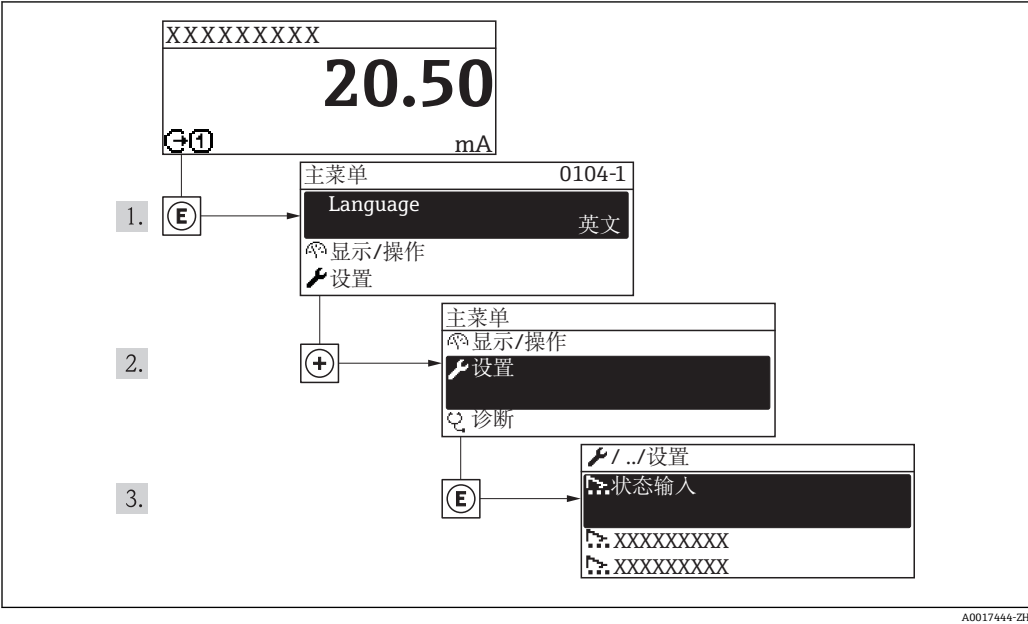
图 23 现场显示示意图
