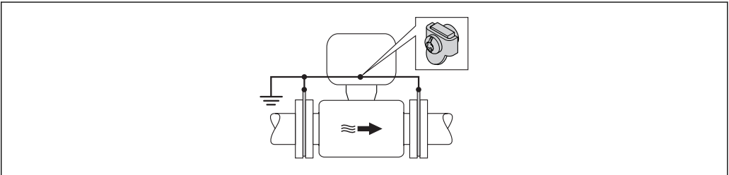
18 通过接地端子和接地环实现系统电势平衡
