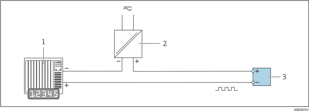
图 14 脉冲/频率输出（无源）的连接实例
