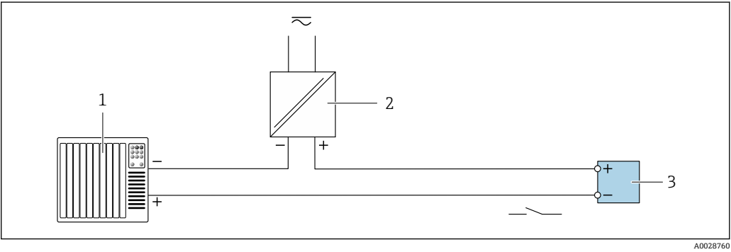
图 16 继电器输出的连接实例(无源)
