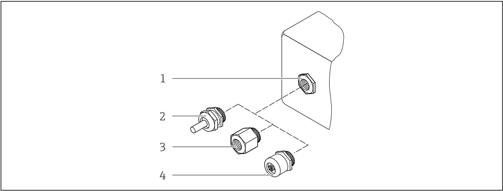
图 36 允许的电缆入口/缆塞 1 内螺纹 M20 × 1.5 2 缆塞 M20 × 1.5 3 电缆入口转接头，带 G ½"或 NPT ½"内螺纹 4 设备插头
