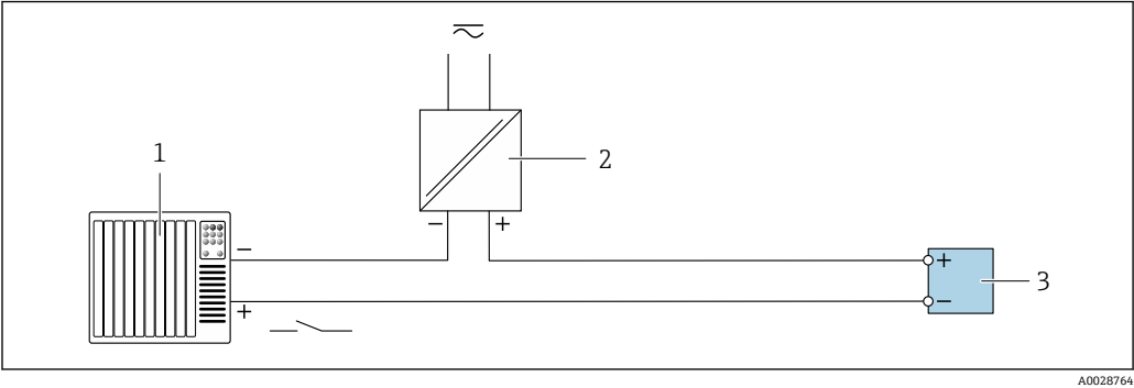
18 状态输入的连接示例 1 带状态输出的自动化系统（例如 PLC） 2 电源 3 变送器
