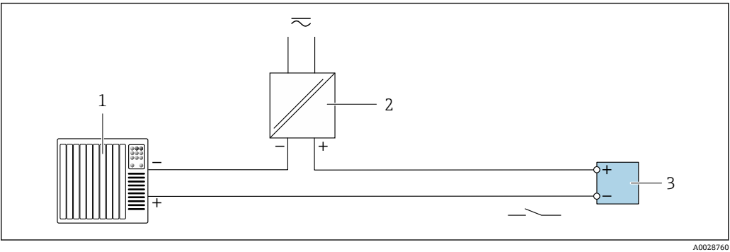
图 15 开关量输出(无源信号)的连接实例
