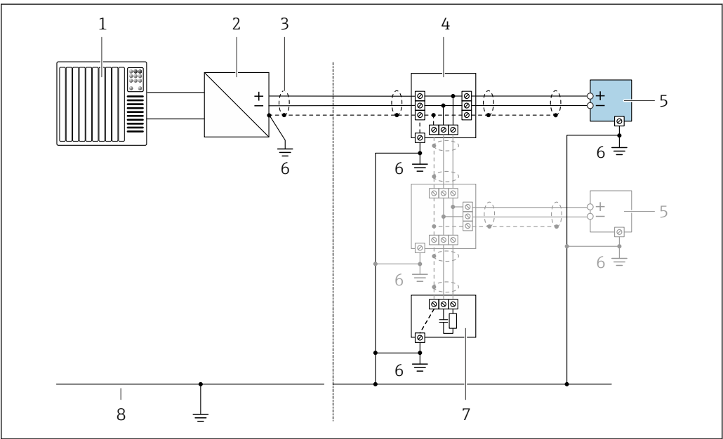
图 11 基金会现场总线(FF)的连接实例
