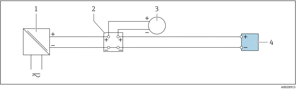
图 17 4...20 mA 电流输入的连接示例
