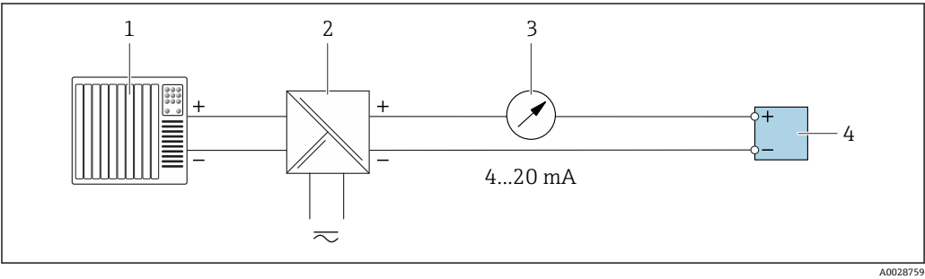
图 13 4...20 mA 电流输出（无源）的连接示例
