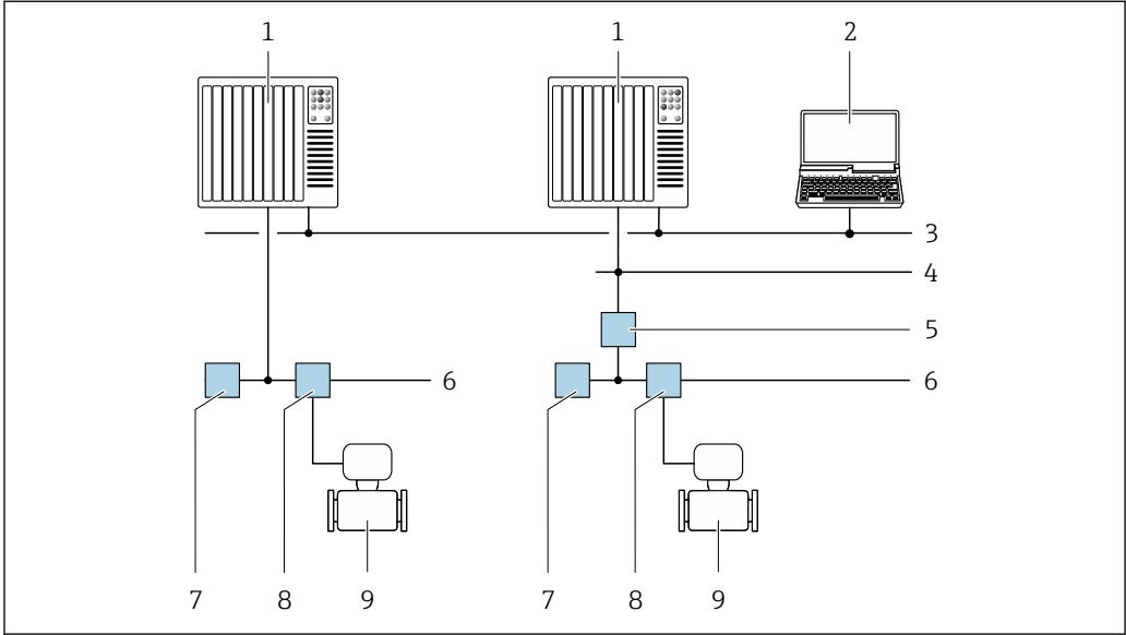
图 23 通过基金会现场总线(FF)网络进行远程操作
