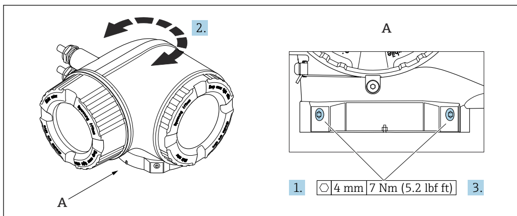
图 6 防爆型外壳
