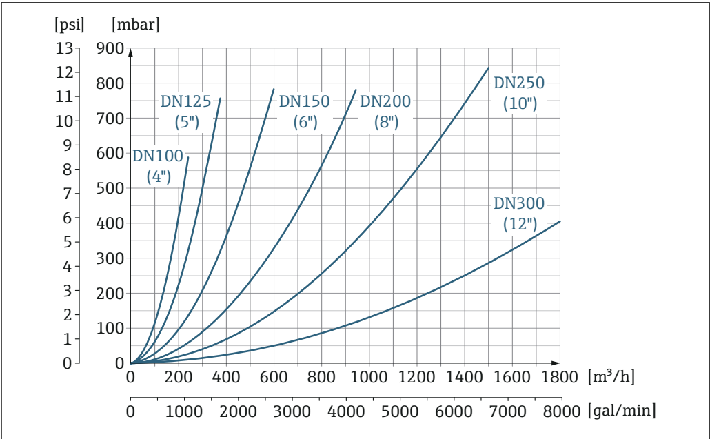
34 压损：适用口径 DN 100...300 (4...12"); 订购选项“设计”，选型代号 C “固定法兰，缩径测量管，无前后直管段长度要求”
