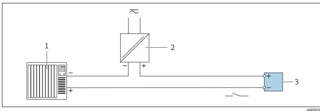
图 25 继电器输出的连接实例(无源)
