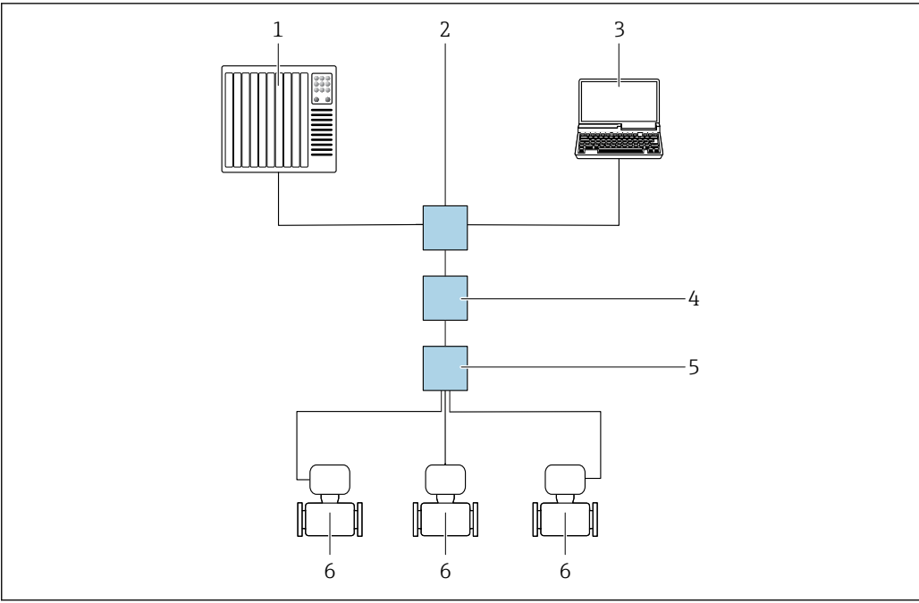
图 26 通过 Modbus TCP + Ethernet-APL 通信进行远程操作（有源信号）
