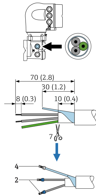
供电电缆
