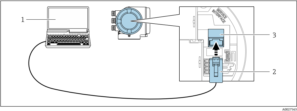
图 29 通过服务接口 (CDI-RJ45) 连接
