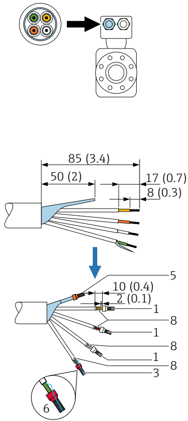
电极电缆
