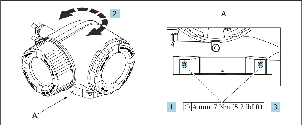
图 6 防爆型外壳
