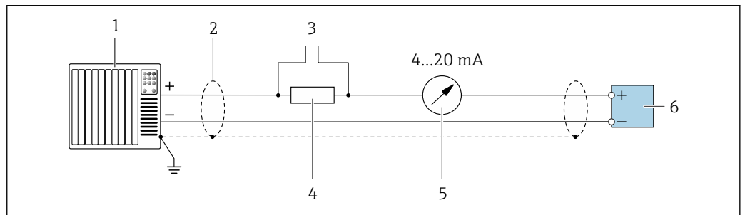
8 接线实例: 4...20 mA HART 电流输出 (有源信号)
