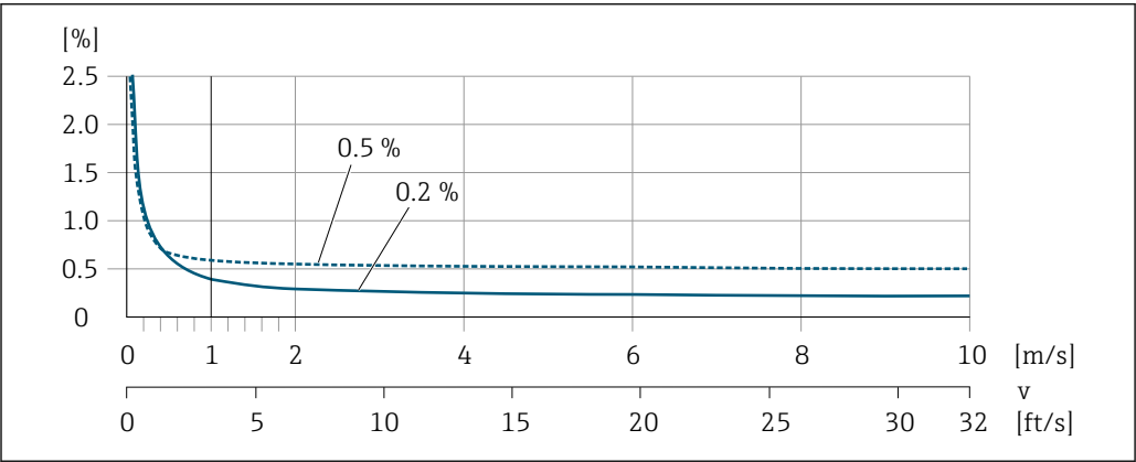
34 最大测量误差 (% o.r.)
