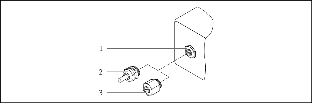
40 允许的电缆入口/缆塞 1 内螺纹 M20 × 1.5 2 缆塞 M20 × 1.5 3 转接头，适用 G ½"或 NPT ½"内螺纹电缆入口
