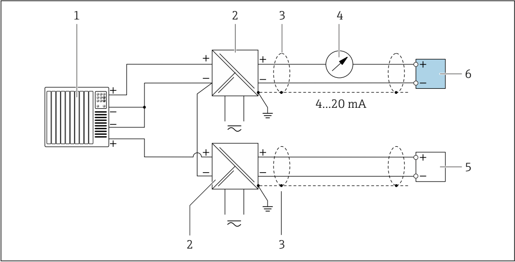
图 10 接线实例：HART 输入，公共端接负极（无源信号）
