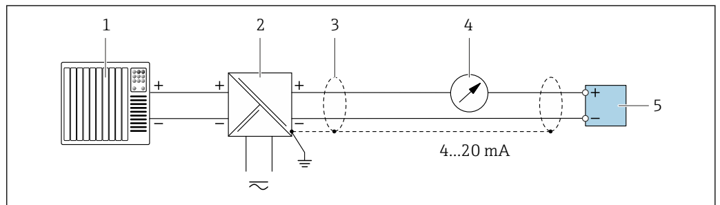
9 接线实例: 4...20 mA HART 电流输出 (无源信号)
