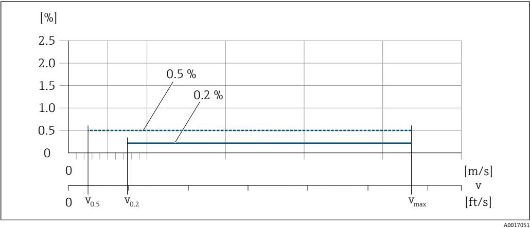
图 35 设计测量精度 (% o.r.)
