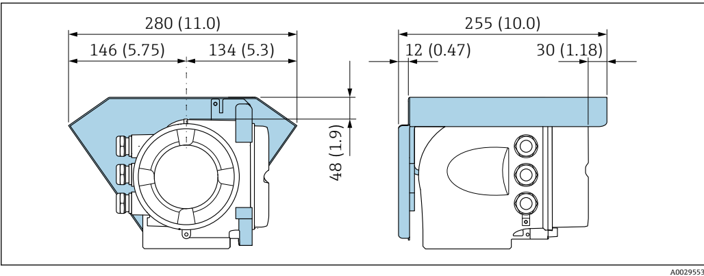
图 4 单位: mm (in)
