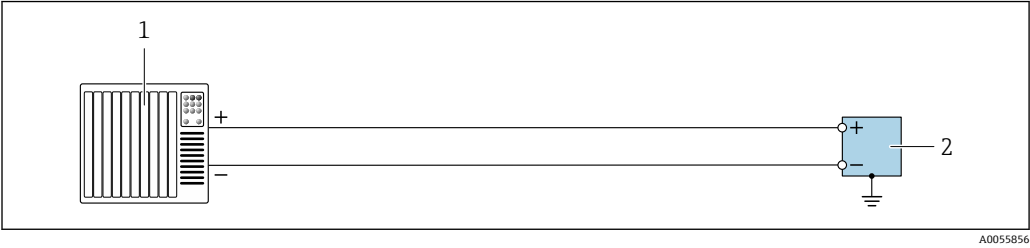
11 接线实例：脉冲输出/频率输出/开关量输出（有源） 1 自动化系统，带脉冲输入/频率输入/开关量输入（例如 PLC） 2 变频器，带脉冲输出/频率输出/开关量输出（有源）
