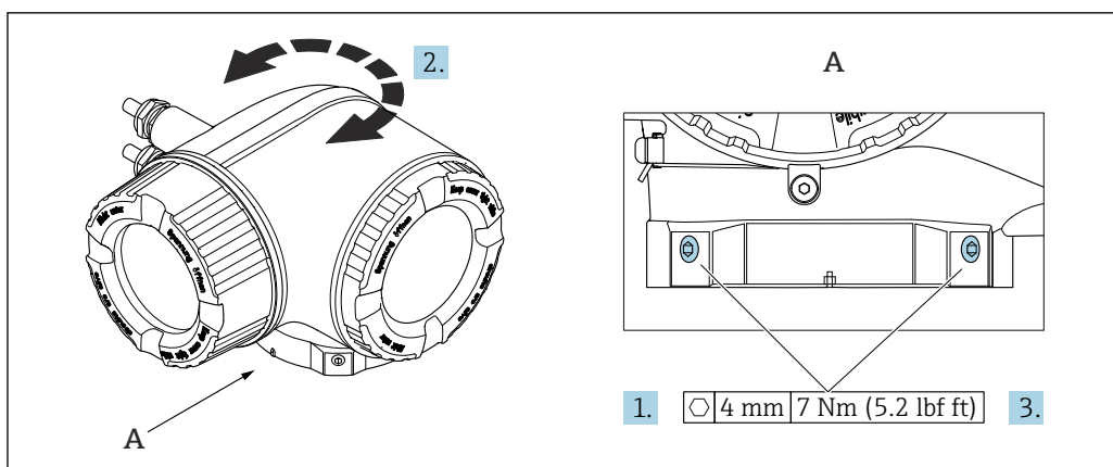
图 6 防爆型外壳
