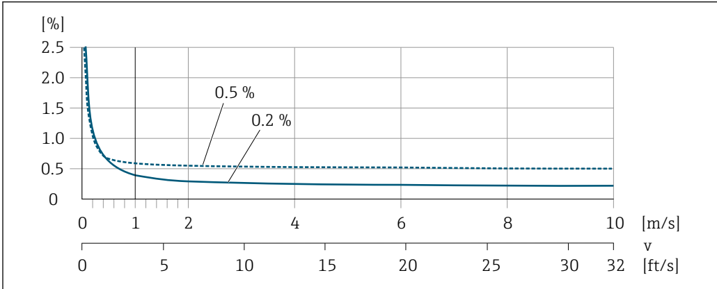
图 28 最大测量误差 (% o.r.)
