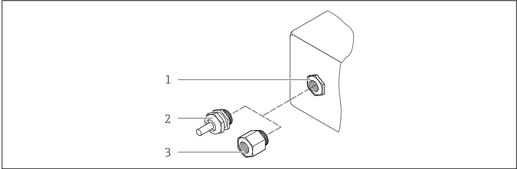
图 18 允许的电缆入口/缆塞 1 电缆入口，在变送器外壳内，带内螺纹 M20 x 1.5 2 M20 x 1.5 缆塞 3 适配接头，适用于带 G ½"和 NPT ½"内螺纹的电缆入口
