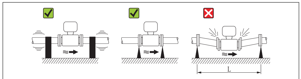
17 避免设备振动的措施( L > 10 \text{ m} (33 ft))
