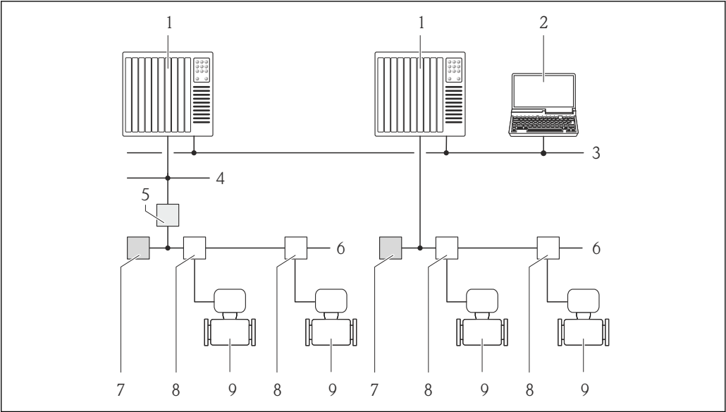
图 22 通过基金会现场总线(FF)网络进行远程操作
