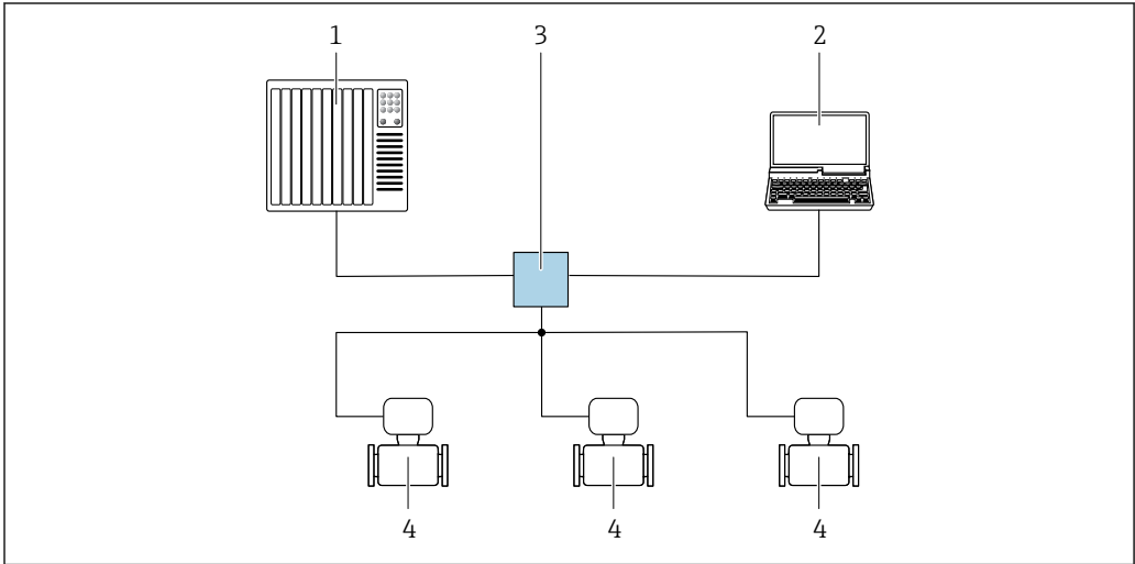
图 14 通过 PROFINET 网络实现远程操作：星形拓扑结构
