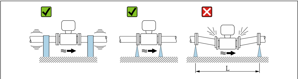
图 7 避免仪表振动的措施 (L > 10 m (33 ft))
