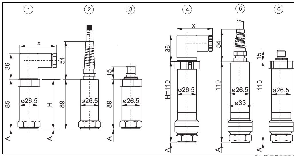
PMP131 和 PMP135 的外壳示意图；材料：AISI 304 (1.4301)
