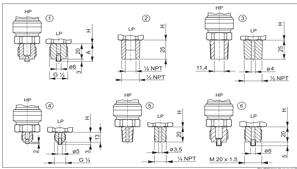
PMP131 的过程连接示意图；材料：AISI 304 (1.4301)
