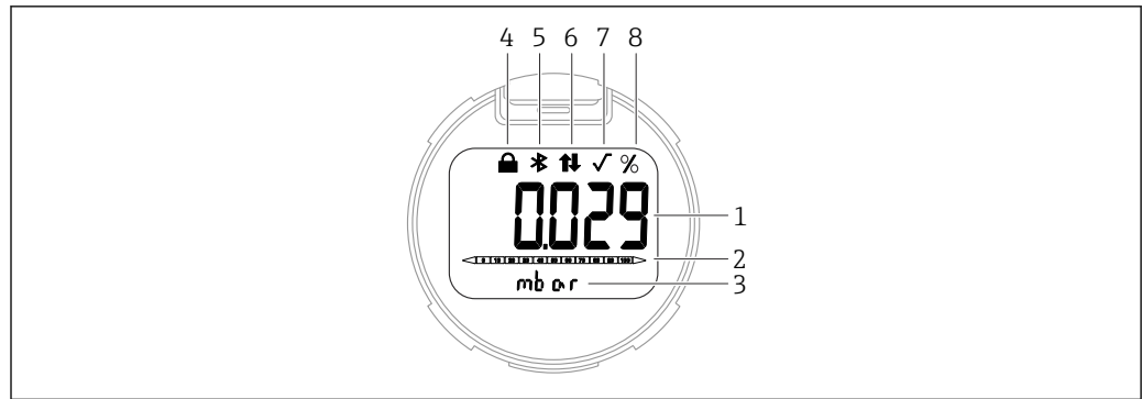
图 7 段码显示屏
