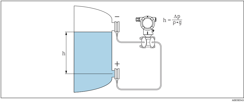
带双侧毛细管隔膜密封系统的仪表
