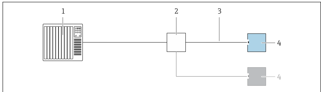
图 4 接线示例: PROFINET + Ethernet-APL
