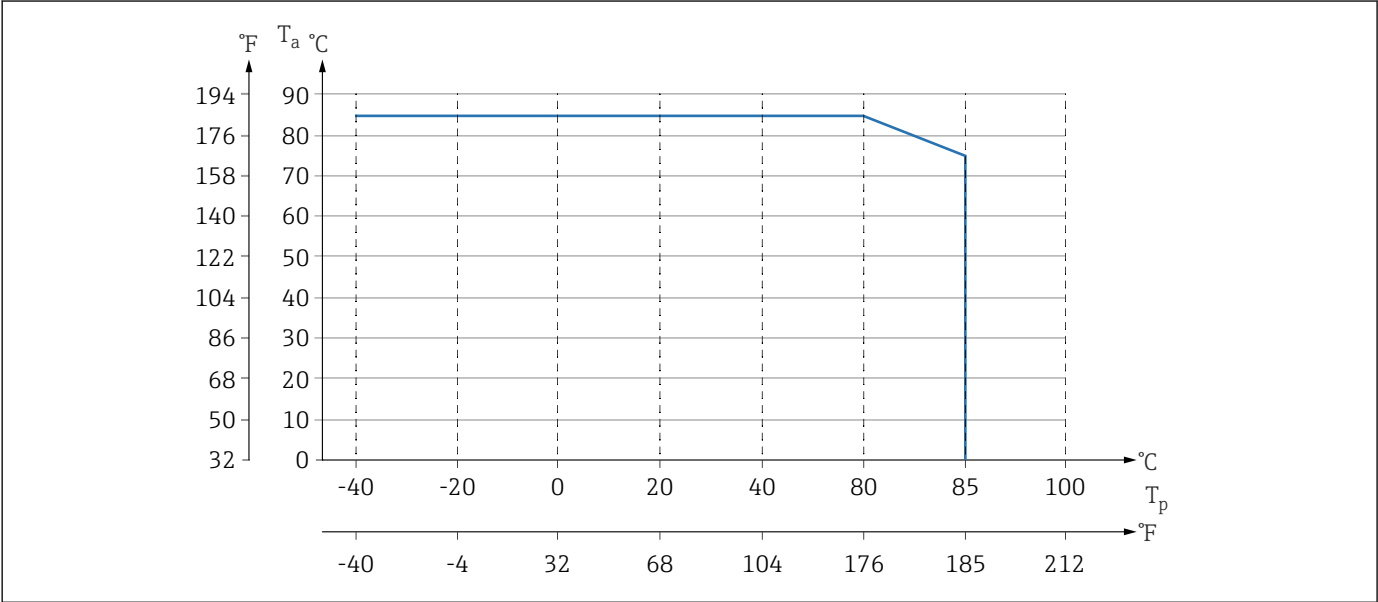
图 13 以上为无保温层垂直安装时的温度范围。 Tp 过程温度 Ta 环境温度
