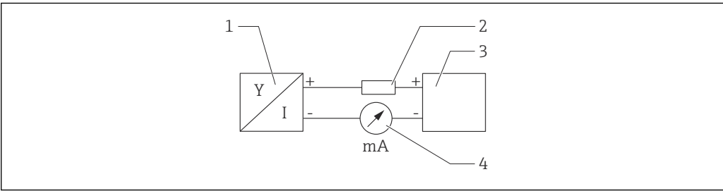
4 HART 接线框图
