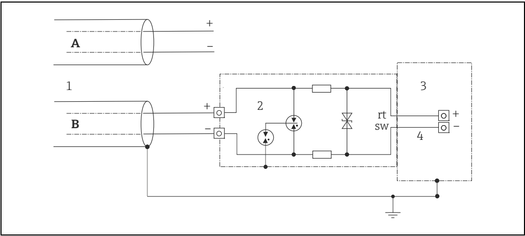
图 14: A 屏蔽层不直接接地 B 屏蔽层直接接地 1 连接进线 2 HAW569-DA2B 3 需要保护的 4 连接电缆
