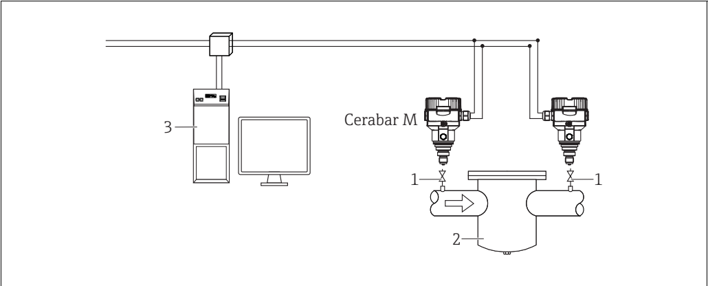
图 37: 1 截止阀 2 例如过滤器 3 FF 主站系统
