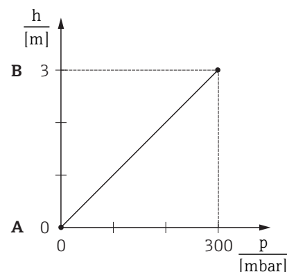
图 21: 带参考压力的标定 - 湿标
