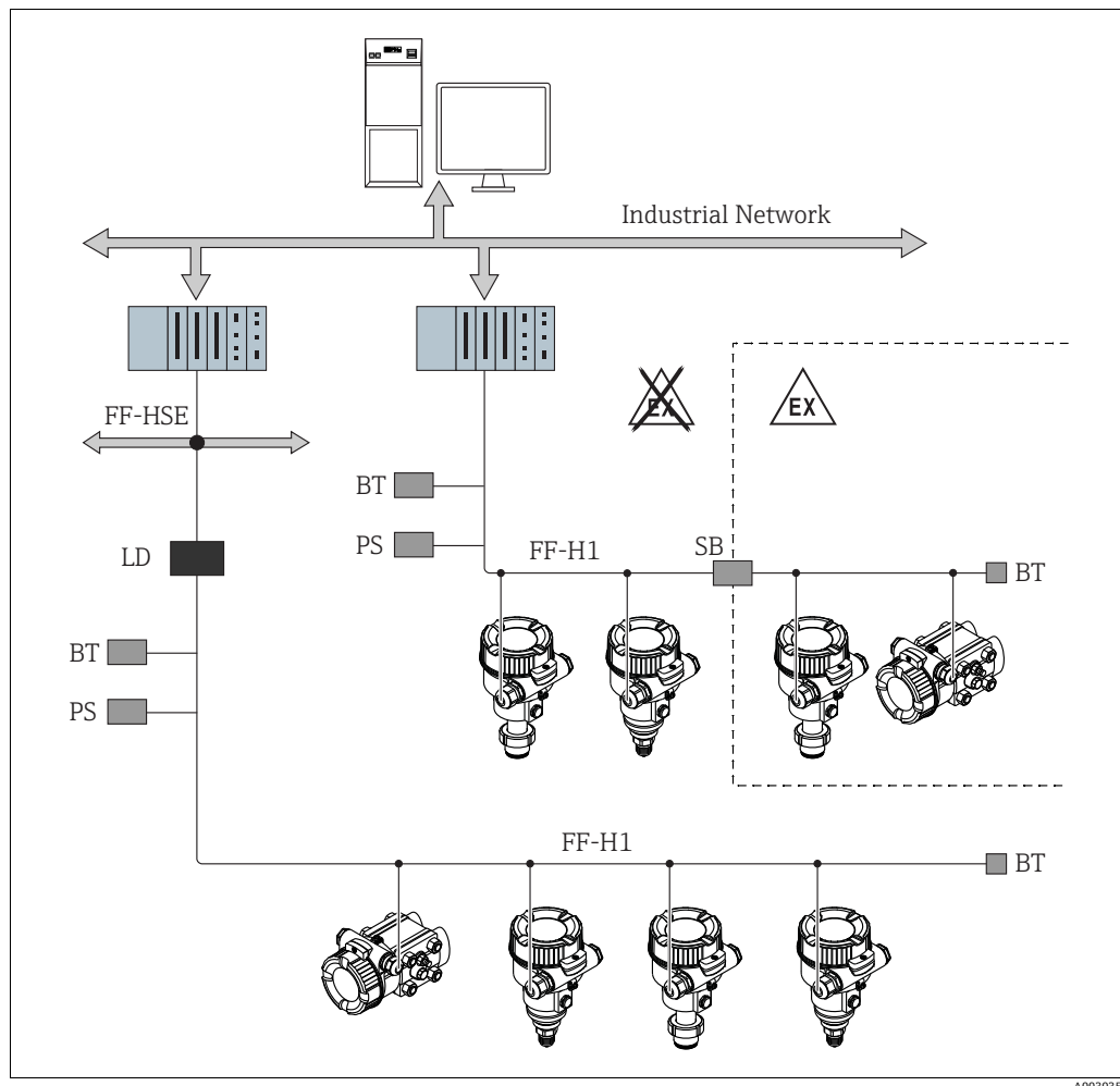
图 18: FOUNDATION Fieldbus 系统架构及组件
