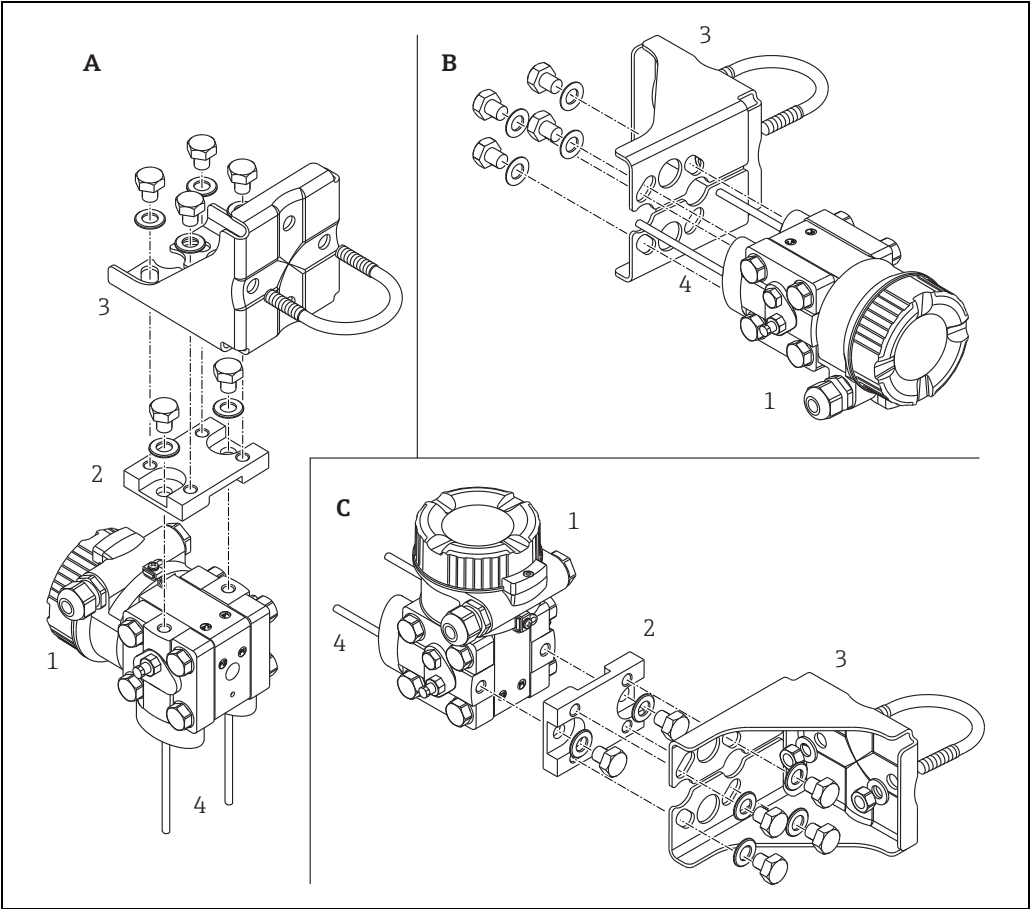
图 8: A 垂直引压管, V1 型, 对齐角度 90° B 水平引压管, H1 型, 对齐角度 180° C 水平引压管, H2 型, 对齐角度 90° 1 Deltabar M 2 转接板 3 安装支架 4 引压管
