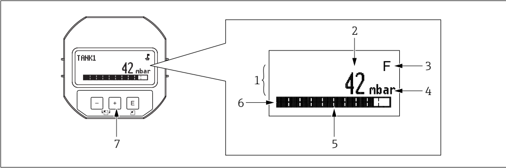
图 17: 显示单元
