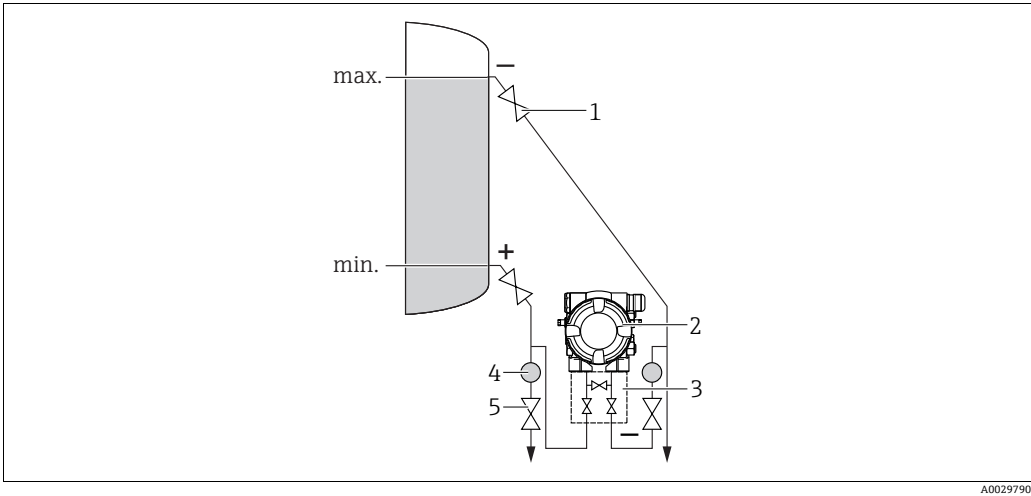
密闭式罐体中的液位测量示意图
