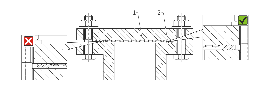
图 5: 1 过程膜片 2 密封圈
