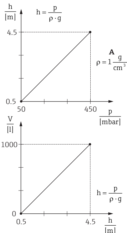
图 27: 带参考压力的标定 - 湿标
