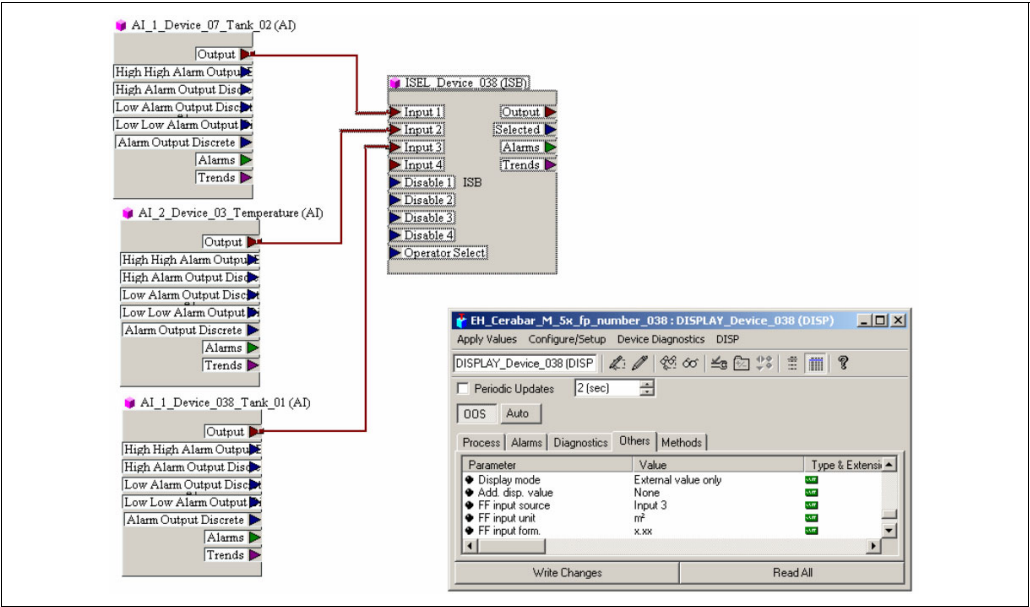
图 38: 连接实例
