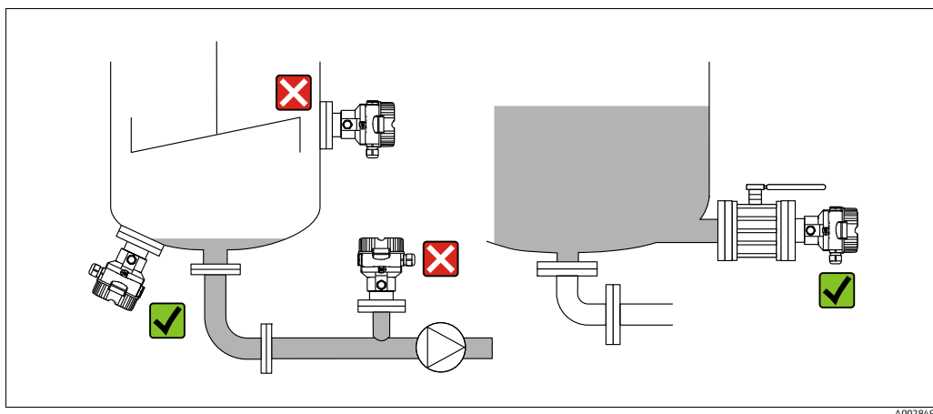
图 9: 液位测量布置
