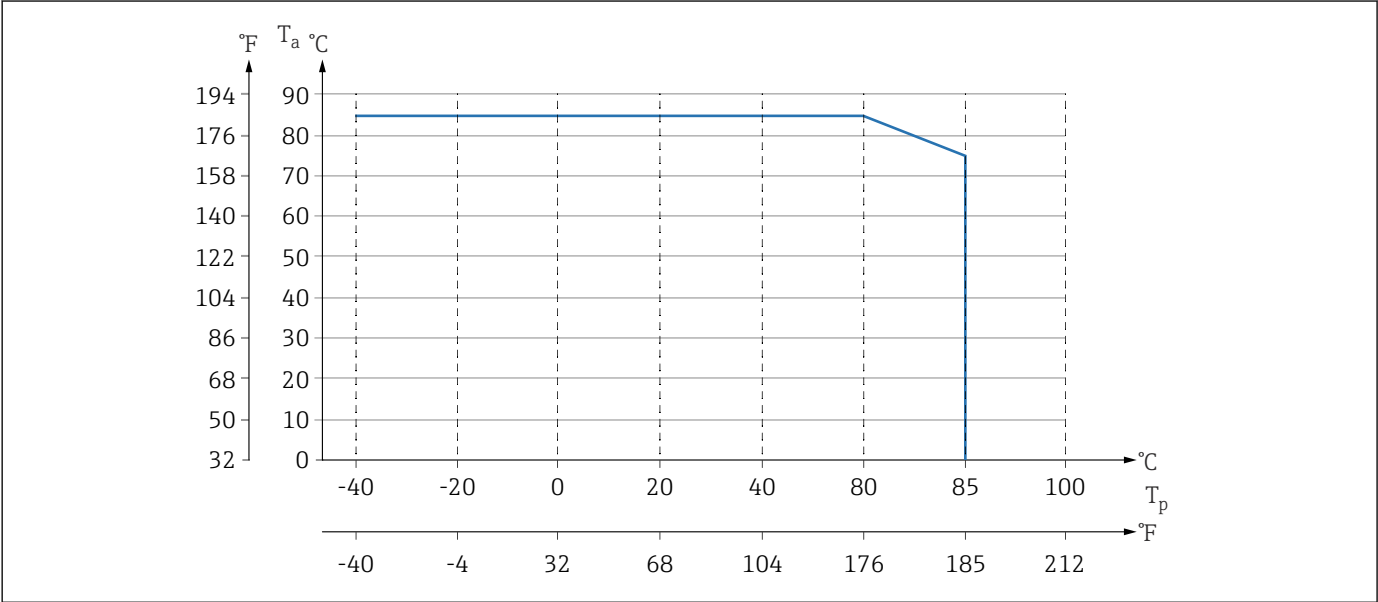
图 5 以上为无保温层竖直安装时的温度范围。 Tp 过程温度 Ta 环境温度
