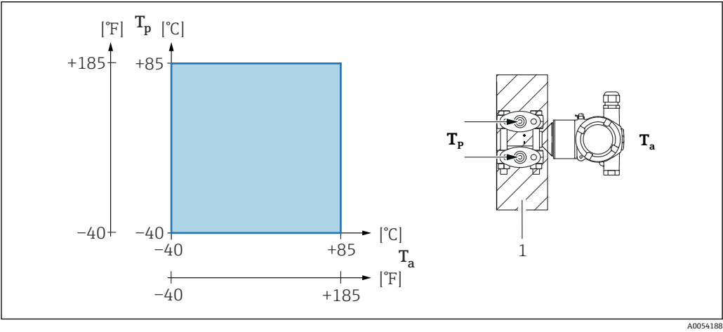
1 保温材料
