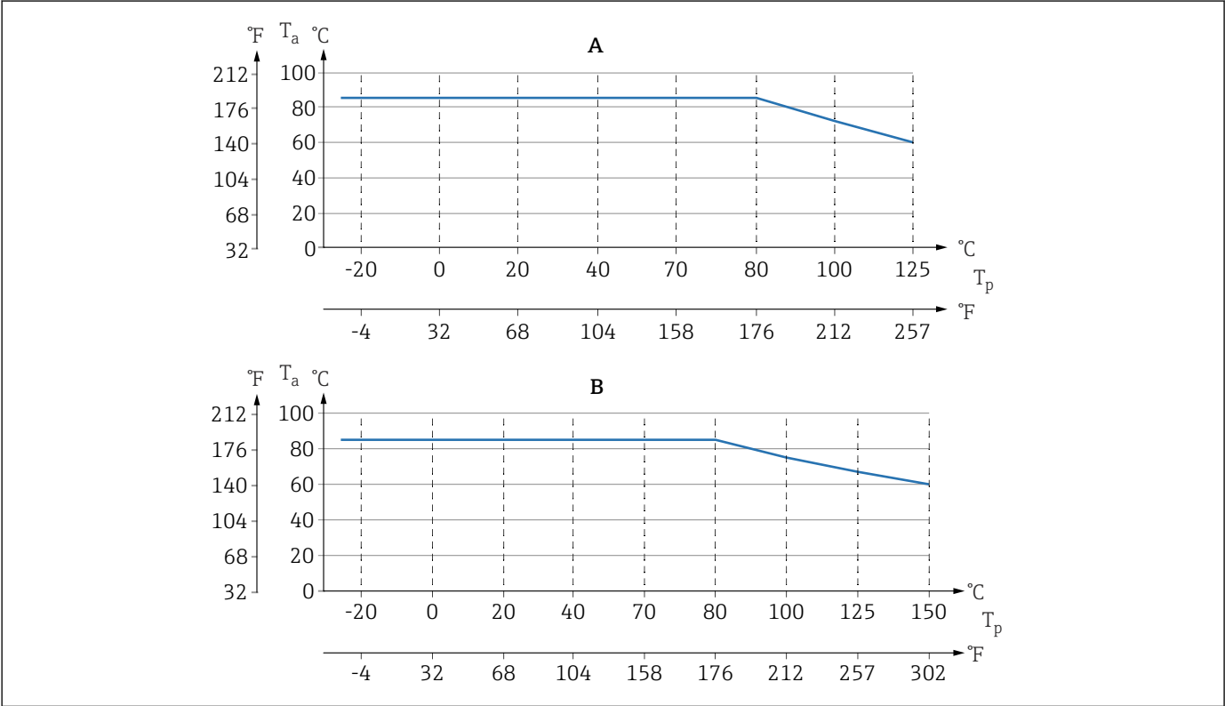
图 12 以上为无保温层竖直安装时的温度范围。
