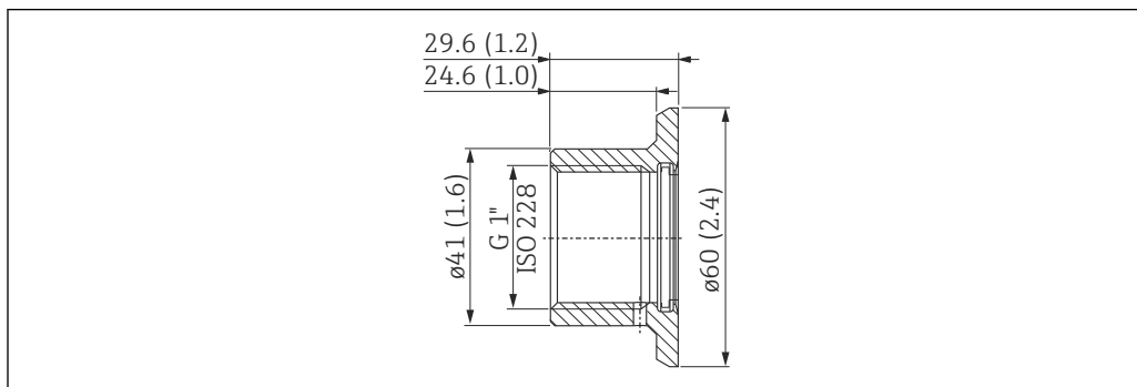
图 7 焊接接头 (G 1, d=60) 的外形尺寸示意图; 安装在罐体上。测量单位 mm (in)
