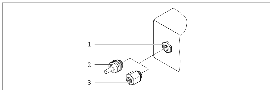
图 41 允许的电缆入口/缆塞
