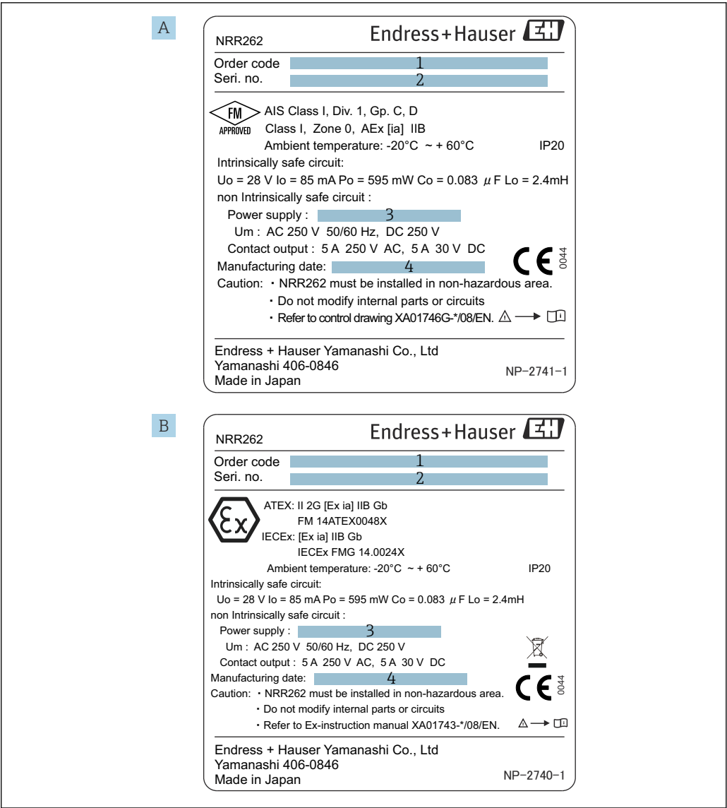
4 NRR262 铭牌
