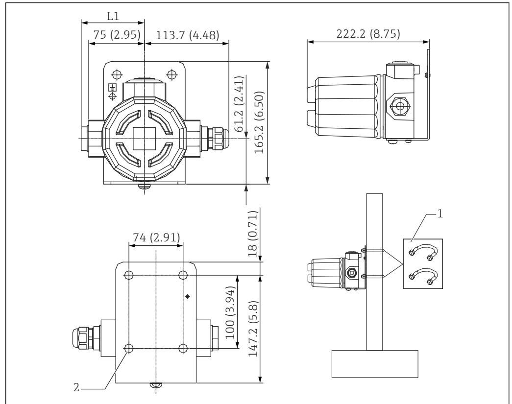
图 10 本安防爆型 (Ex [ia]) 传感器数据转换盒的外形尺寸示意图。测量单位 mm (in)
