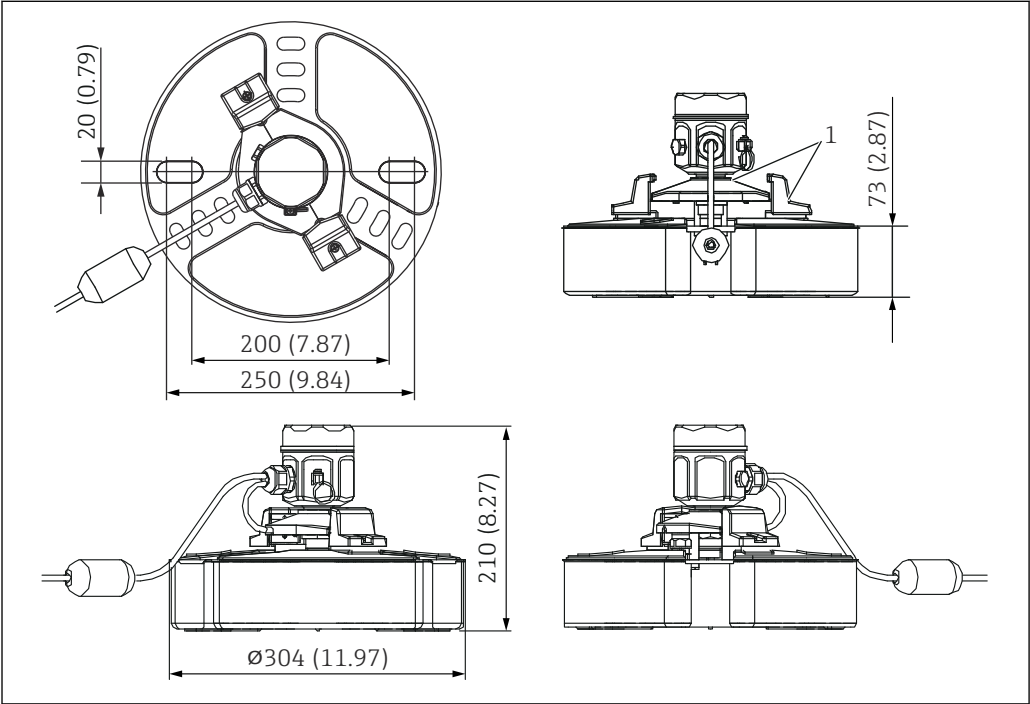
图 7 NAR300 浮子开关的外形尺寸示意图
