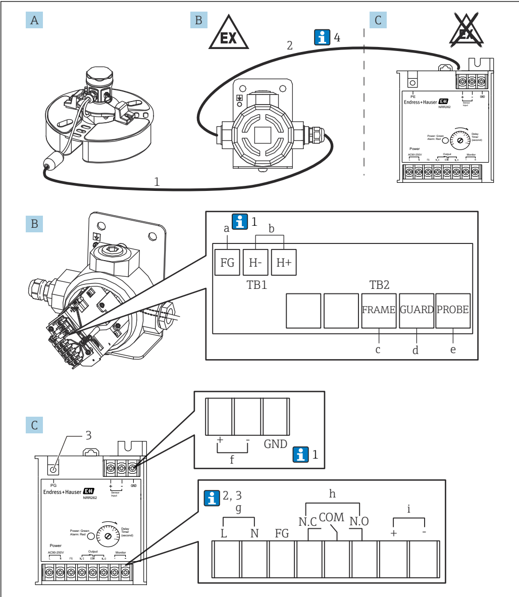
图 17 本安防爆型 (Ex ia) 转换器 NRR262-4/A/B/C 接线示意图
