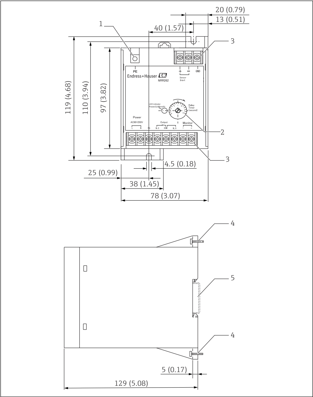
图 9 NRR262 的外形尺寸示意图。测量单位 mm (in)
