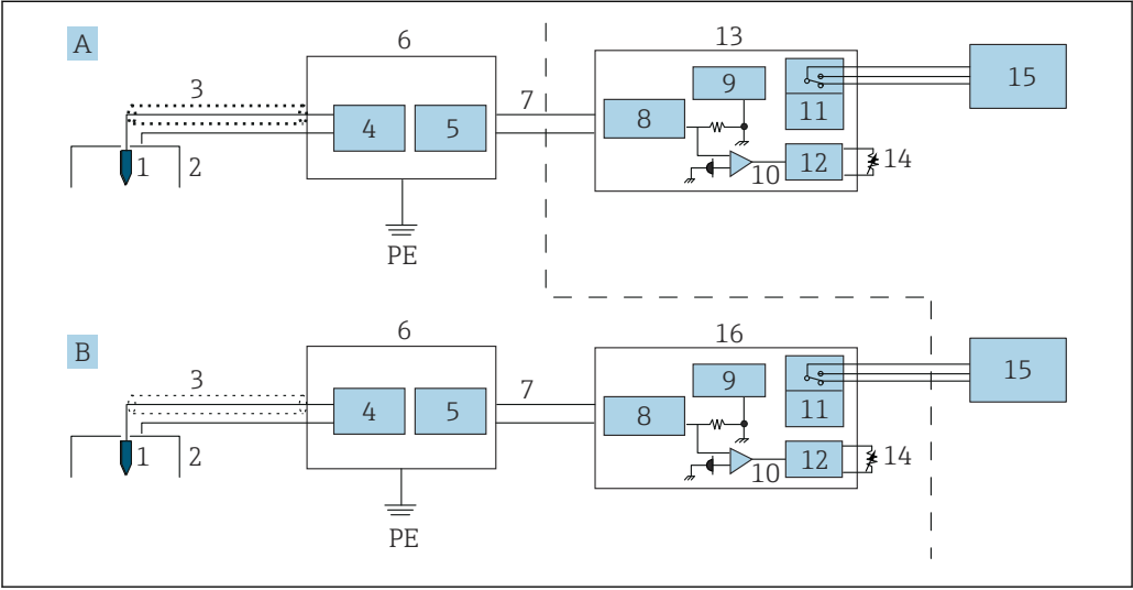
19 接线图
