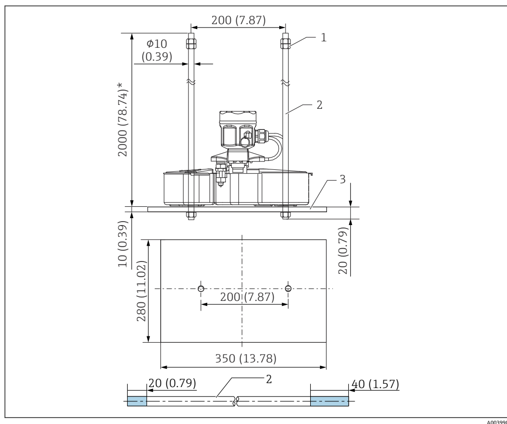
图 22 浮子导杆
