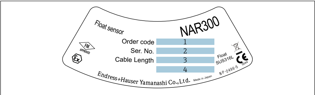
图 2 NAR300 铭牌
