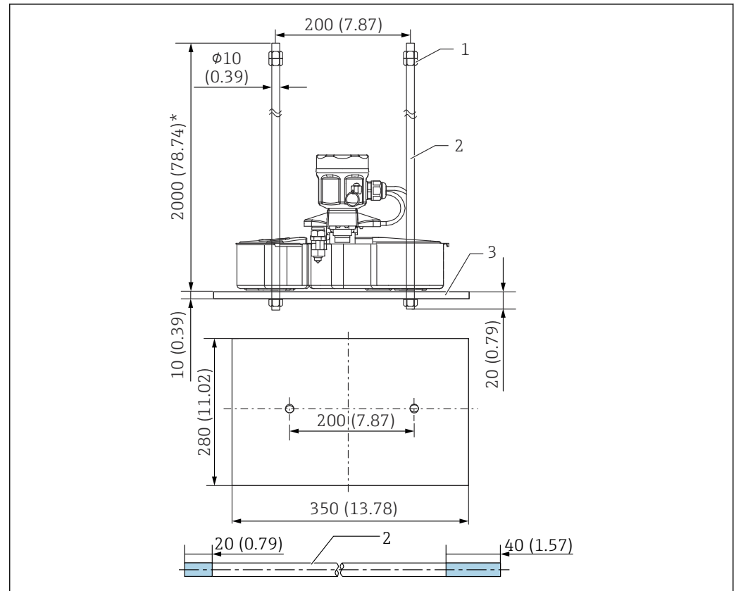
13 NAR300, 浮子导杆
