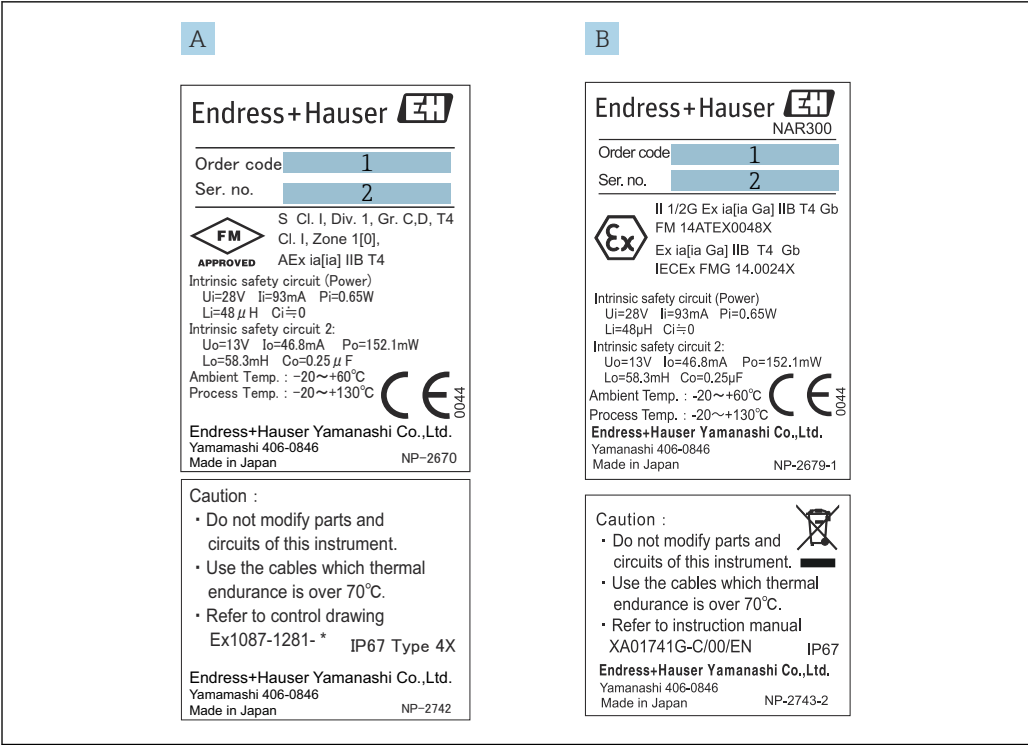
3 NAR300 铭牌 A NAR300, FM 认证型 B NAR300 ATEX / IECEx 认证铭牌 1 订货号 2 序列号
