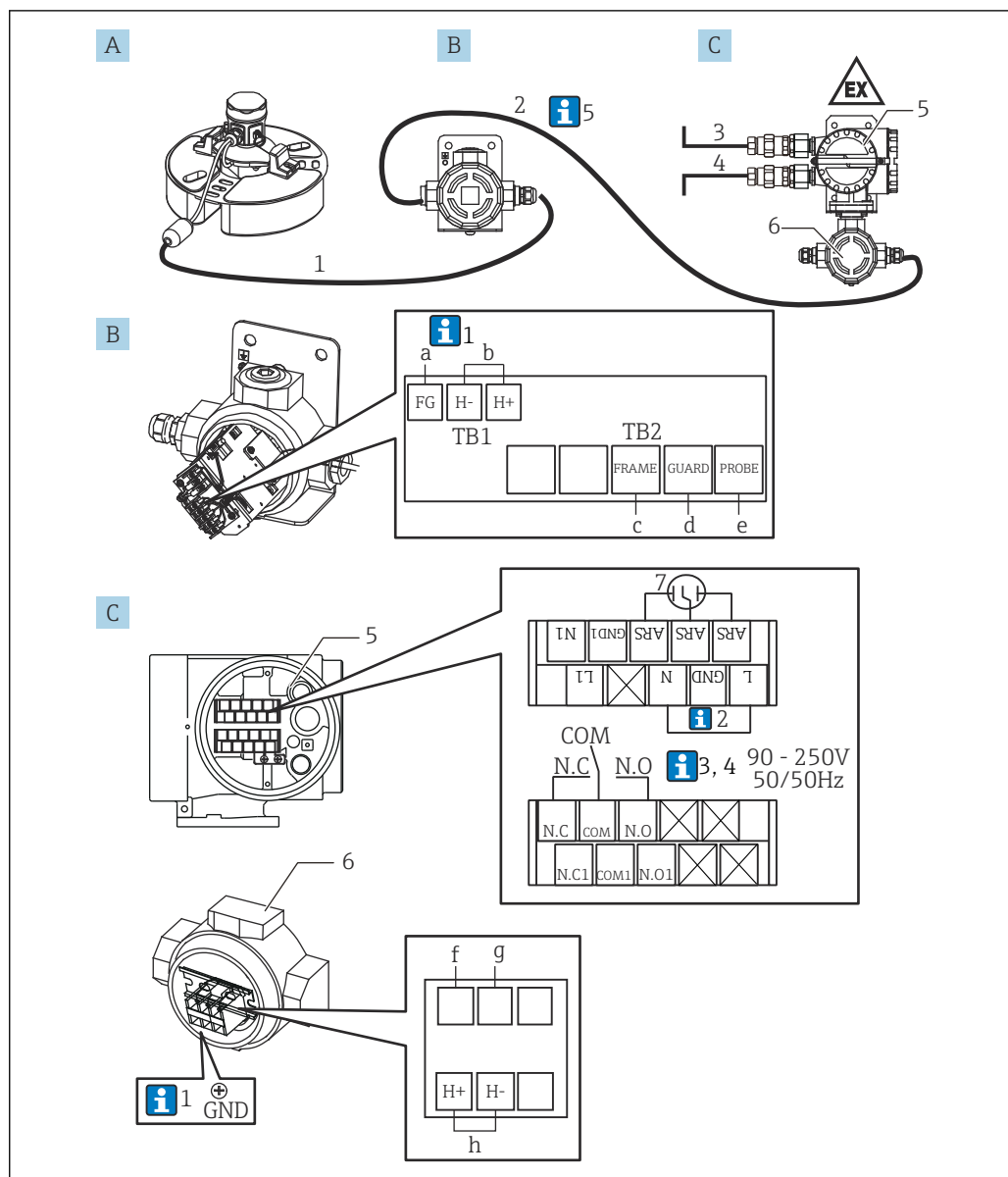
18 本安隔爆型 (Ex d [ia]) 转换器 NRR261-5 接线示意图
