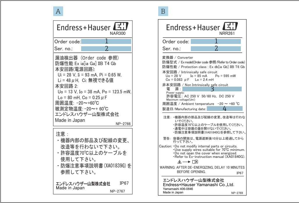
5 JPN 防爆认证铭牌 A NAR300 JPN 防爆认证铭牌 B NRR261 JPN 防爆认证铭牌 (NAR300 分体式) 1 订货号 2 序列号 3 供电电压 4 生产日期
