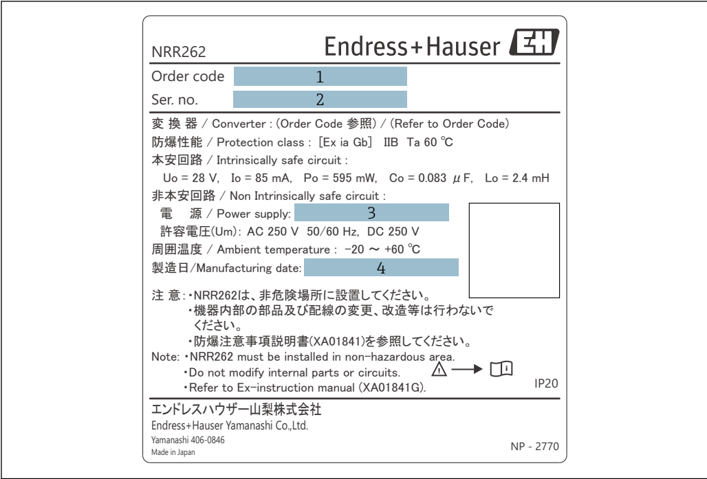
6 NRR262 JPN 防爆认证铭牌 1 订货号 2 序列号 3 供电电压 4 生产日期
