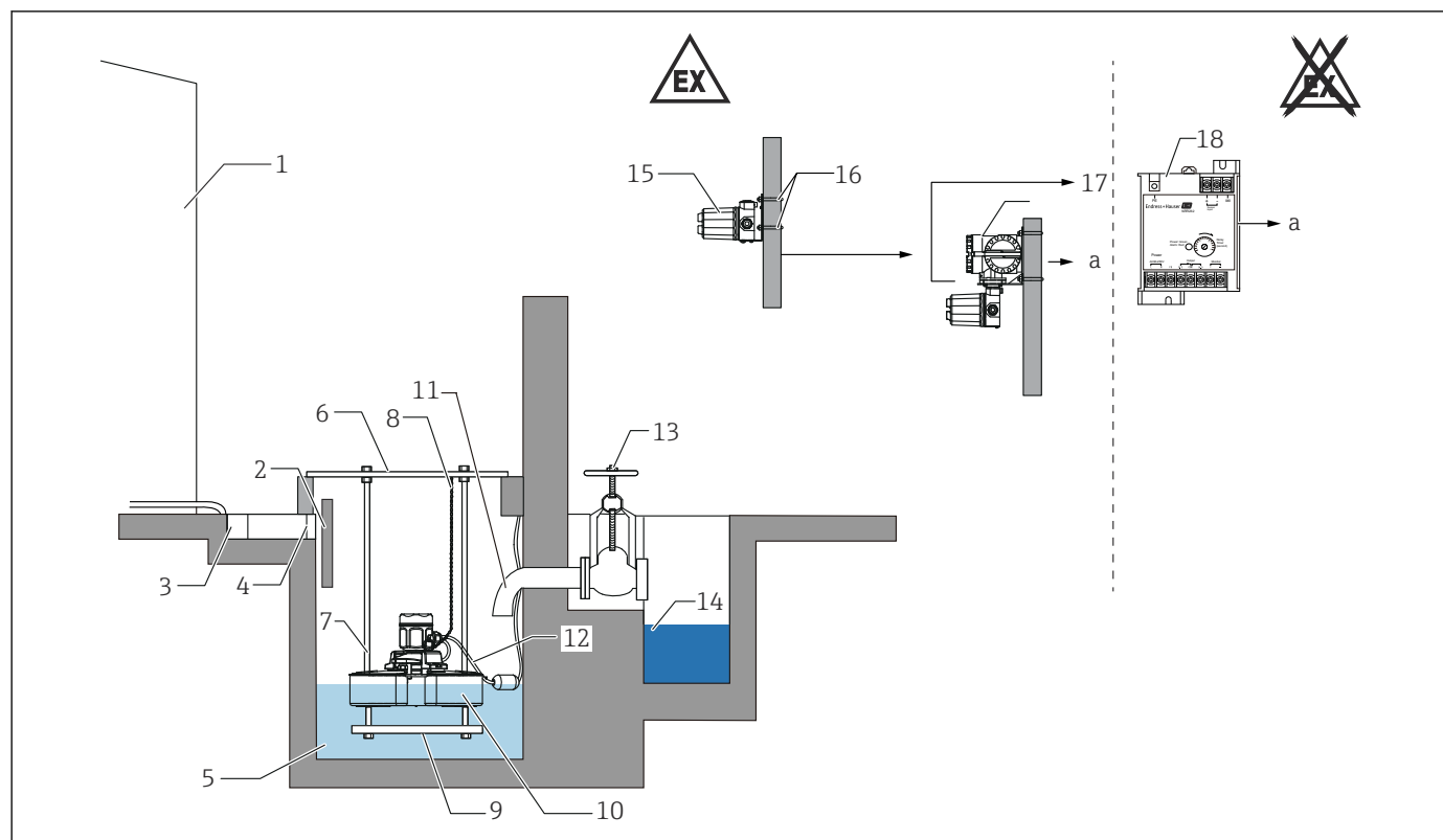
图 11 NAR300 + NRR26x
