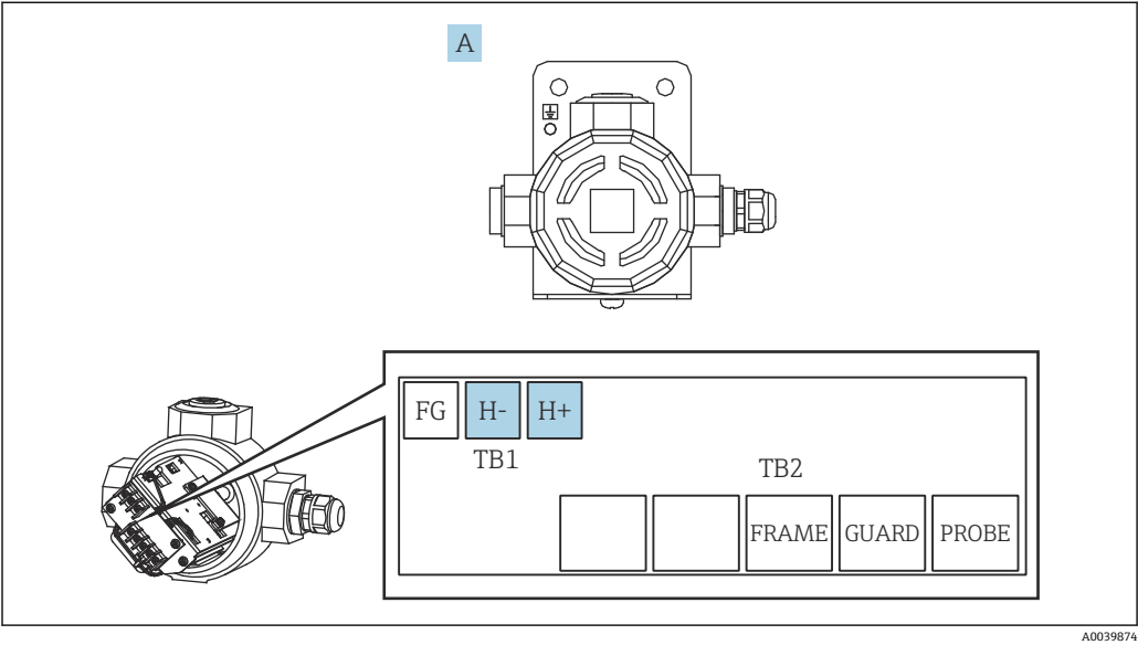
图 20 本安型接线盒 A 防爆型传感器数据转换盒 H- 蓝色 H+ 蓝色
