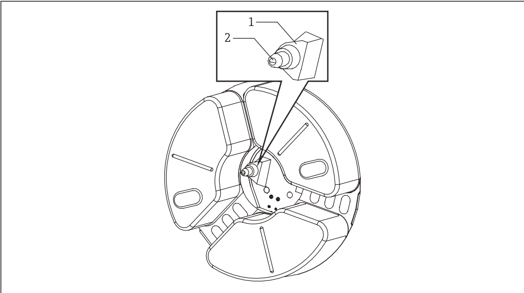
图 21 传感器清洁
