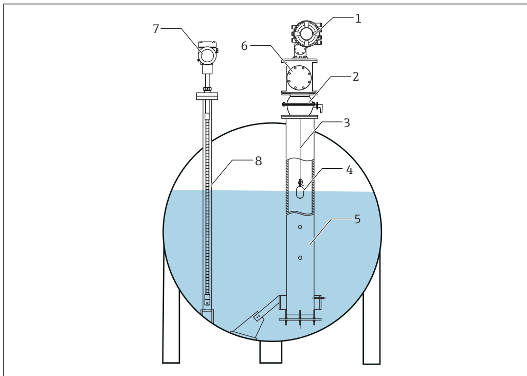
图 24 在高压罐中安装保护套管
