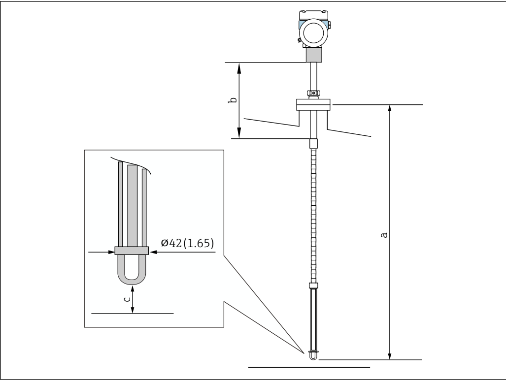
14 推荐安装高度。测量单位 mm (in) a 推荐安装高度 b 约± 180 mm (7.09 in)，总计 360 mm (14.17 in)（可调范围） c 取决于仪表配置
