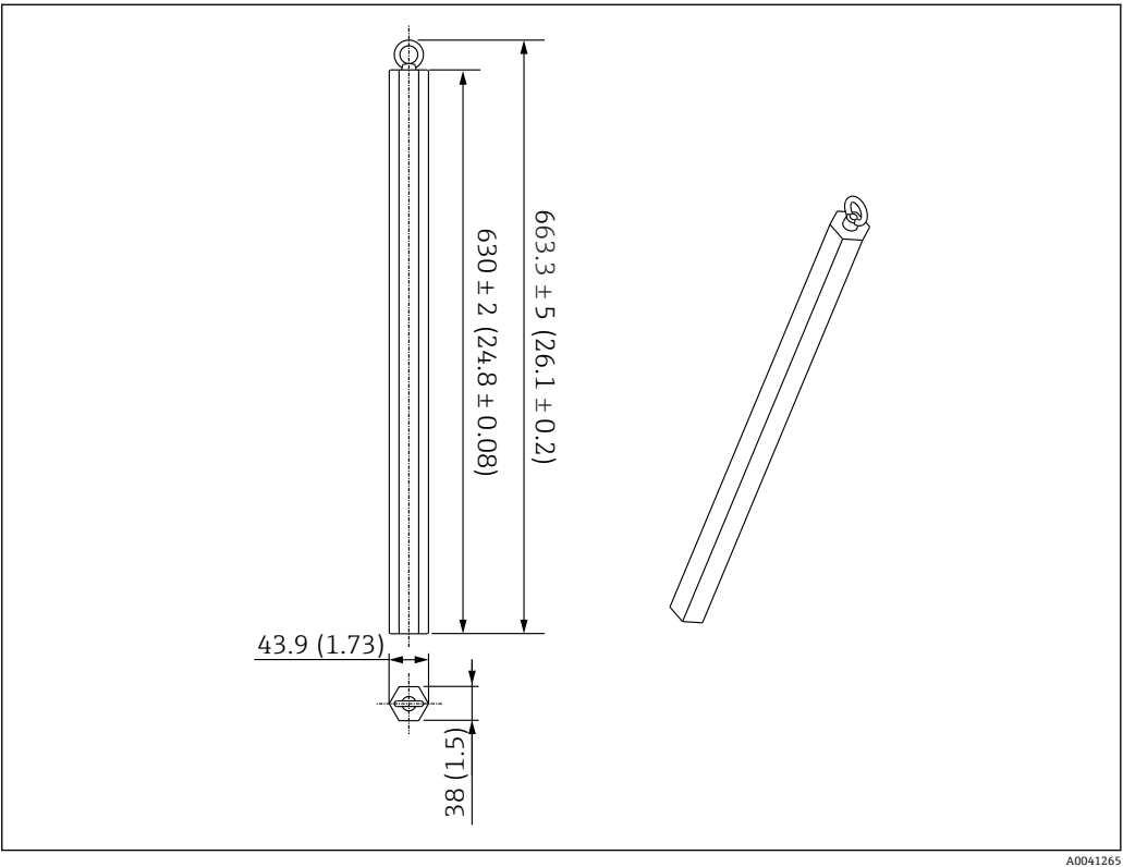
40 安装附件。测量单位 mm (in)
