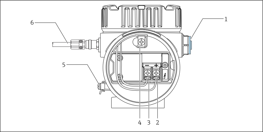
图 5 NMT81 的接线端子 (ATEX 本安防爆)
