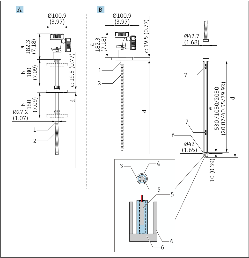
30 “转换器+平均温度探头+油水界面测量探头”型仪表。测量单位 mm (in)
