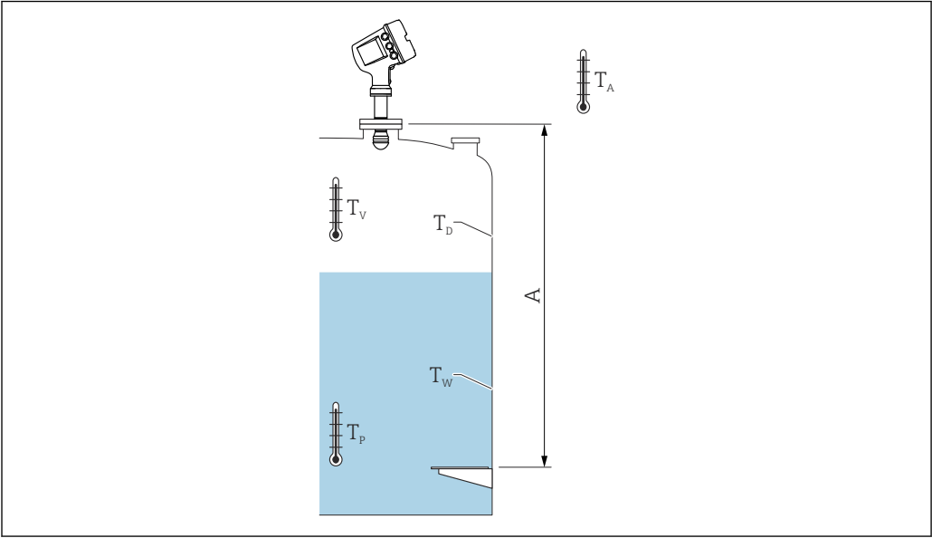
57 “CTSh calculation”参数
