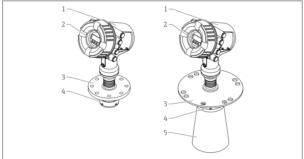
图 1 Micropilot NMR84 的结构示意图
