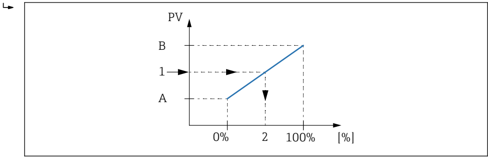
41 按百分比调整罐体参数
