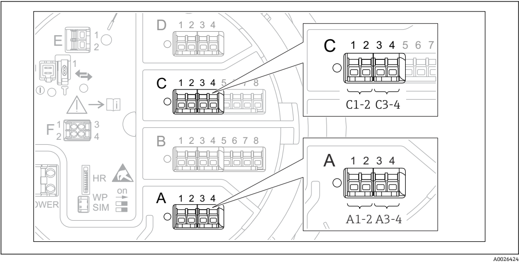
图 14 数字量输入或输出的名称（实例）
