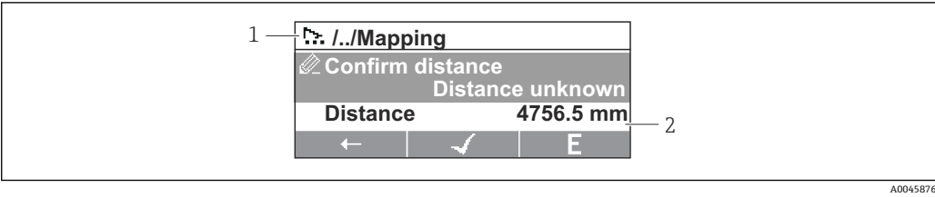
图 18 显示单元上的设置向导界面
