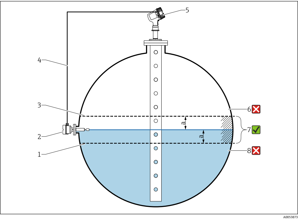
图 37 带液位开关的应用实例
