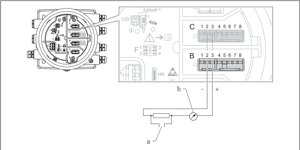
图 11 输出模式下的有源模拟量输入/输出模块
