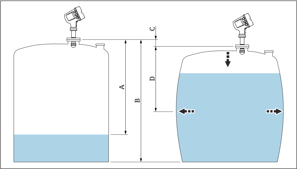
34 静压式储罐变形校正 (HyTD)
