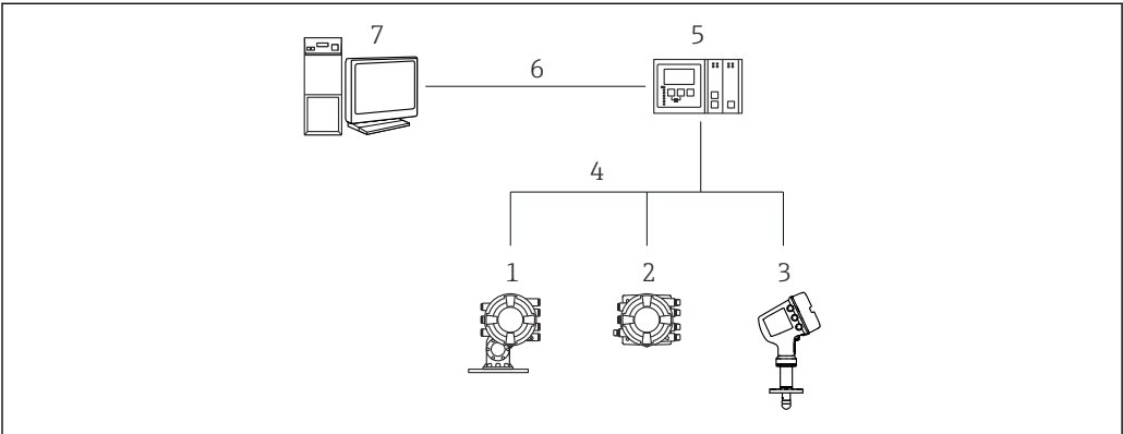
24 通过 Tankvision 储罐扫描仪 NXA820 连接伺服罐表设备至 FieldCare 1 Proservo NMS8x 2 罐旁指示仪 NRF81 3 Micropilot NMR8x 4 现场通信协议 (例如 Modbus、V1) 5 Tankvision 罐体扫描仪 NXA820 6 以太网 7 计算机, 安装有 FieldCare
