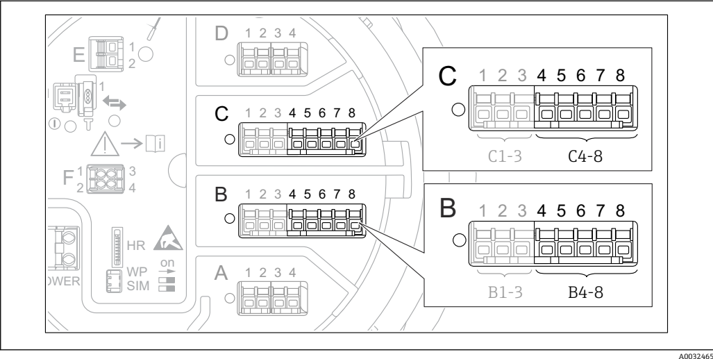
49 “Analog IP” 子菜单的接线端子（分别为“B4-8”或“C4-8”）
