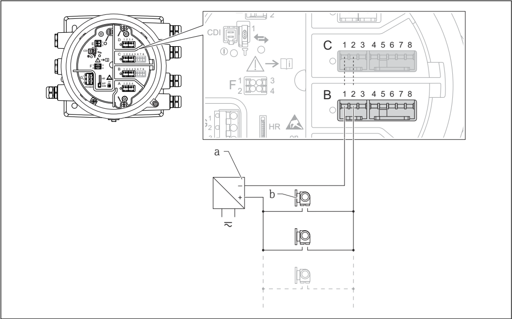
图 10 HART 主站模式下的无源模拟量输入/输出模块
