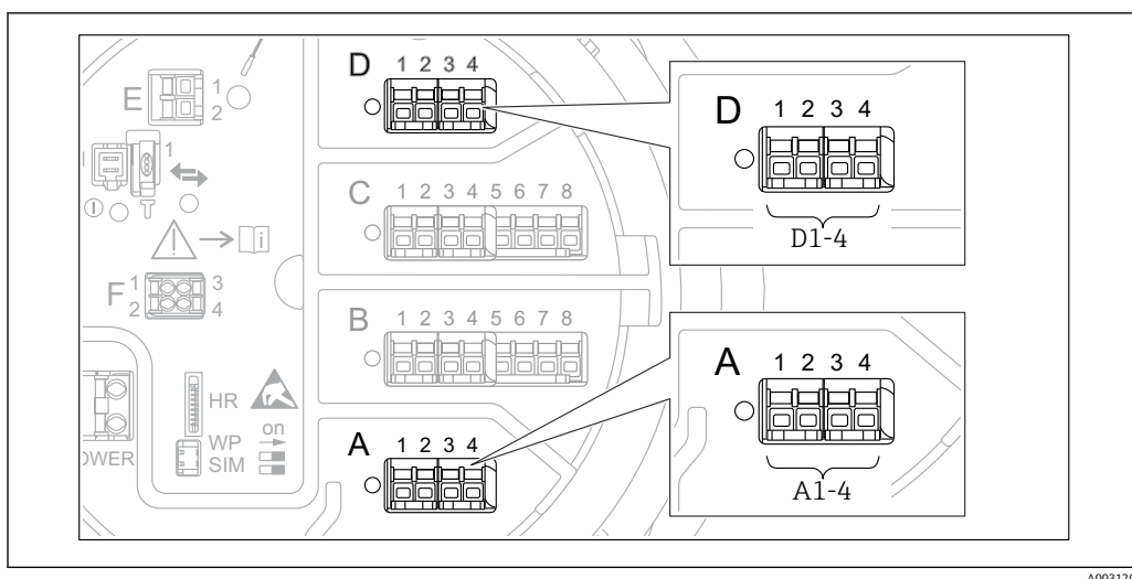
图 7 “Modbus”模块、“V1”模块或“WM550”模块的名称（实例）：这些模块可能位于插槽 B 或 C 中，与设备具体型号相关。
