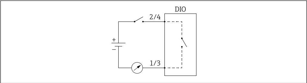
46 数字量输入输出模块用作数字量输出
