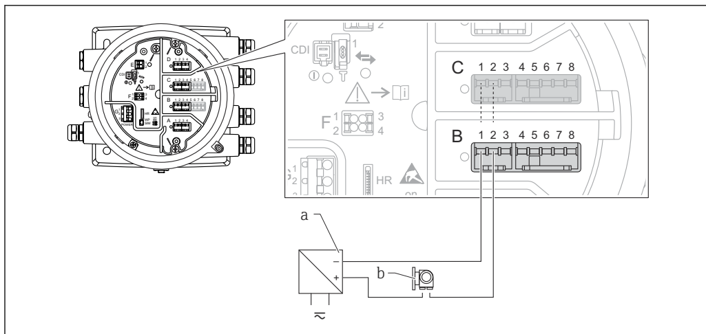
图 9 输入模式下的无源模拟量输入/输出模块
