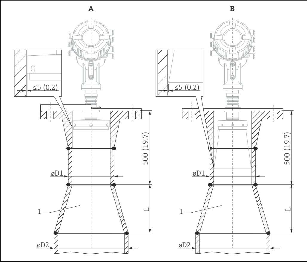
图 3 在较大管径的导波管中安装 NMR84
