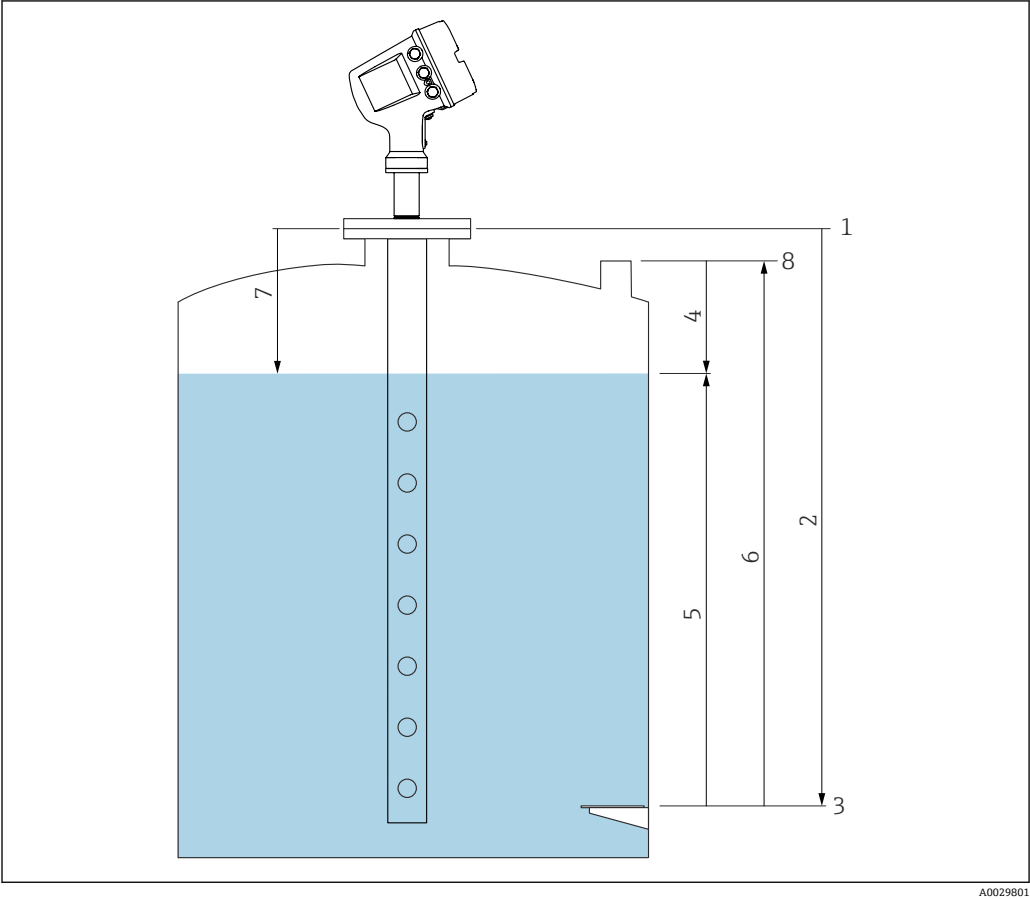
图 25 雷达罐体测量术语
