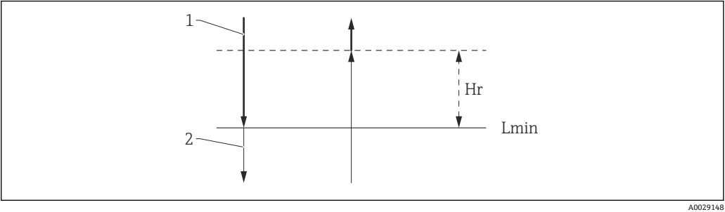
59 HTMS 单点回差控制范围
