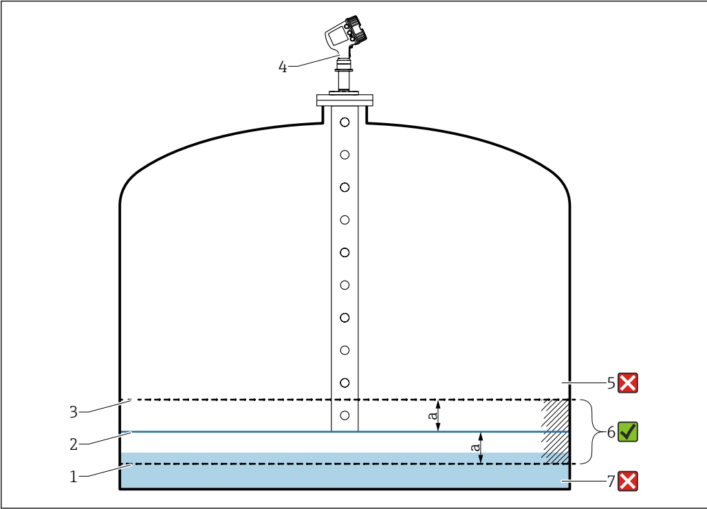
36 导波管末端固定参考点的应用实例
