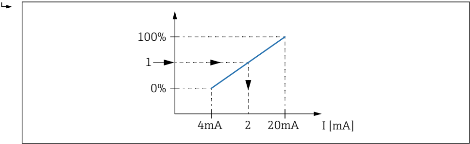
图 40 按输出电流调整罐体参数 1 罐体参数 2 输出电流
