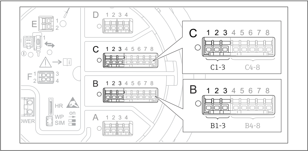
图 39 用作 4...20 mA 输出的模拟量输入/输出模块的可能安装位置。设备的订货号确定当前使用的模块 → 图 20。
