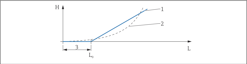
图 56 计算 HyTD 校正值
