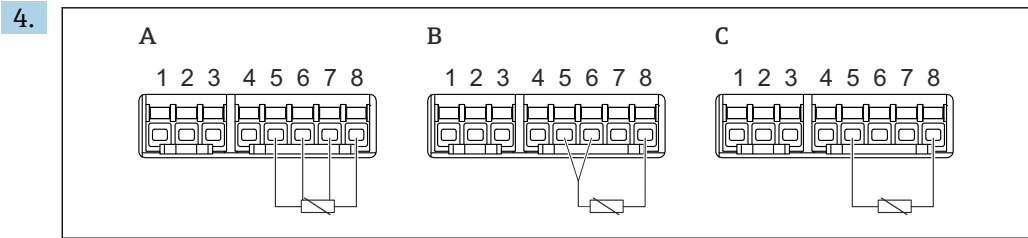
图 32 热电阻连接方式
