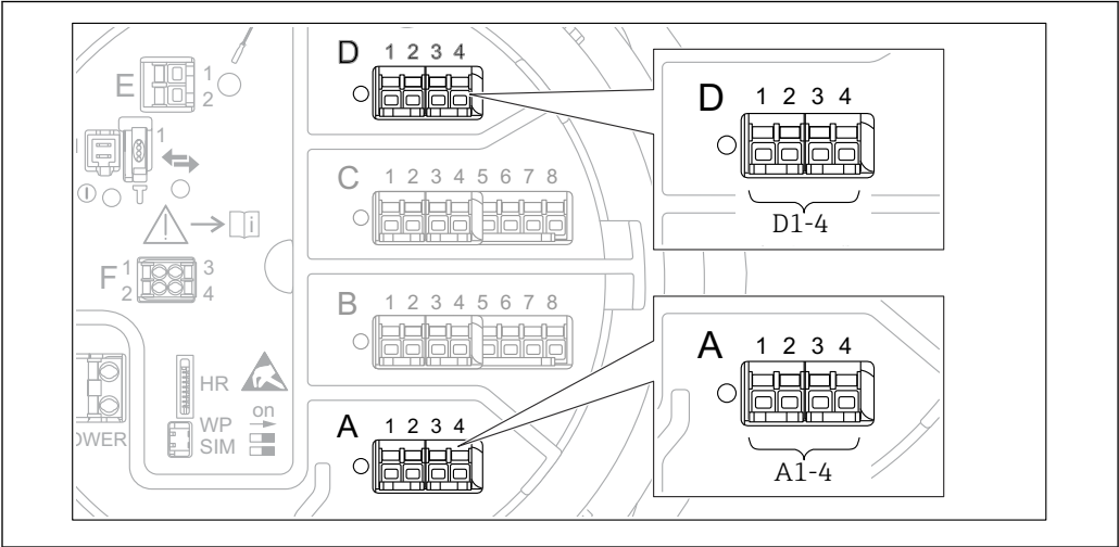
图 44 WM550 模块的可能安装位置（实例）；取决于设备型号，上述模块还可以安装在插槽 B 或 C 中→ 图 20。
