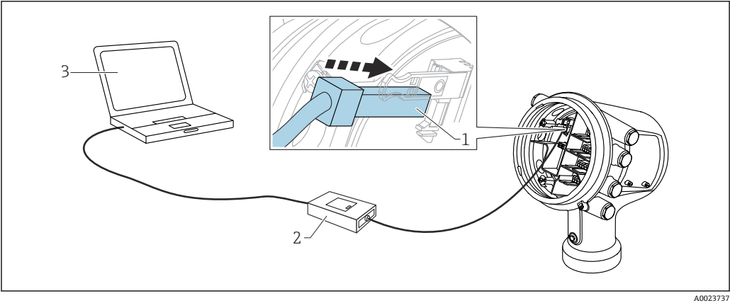
23 通过服务接口操作 1 服务接口 (CDI = Endress+Hauser 通用数据接口) 2 Commubox FXA291 3 计算机, 安装有“FieldCare”调试软件, 带“CDI Communication FXA291”COM DTM
