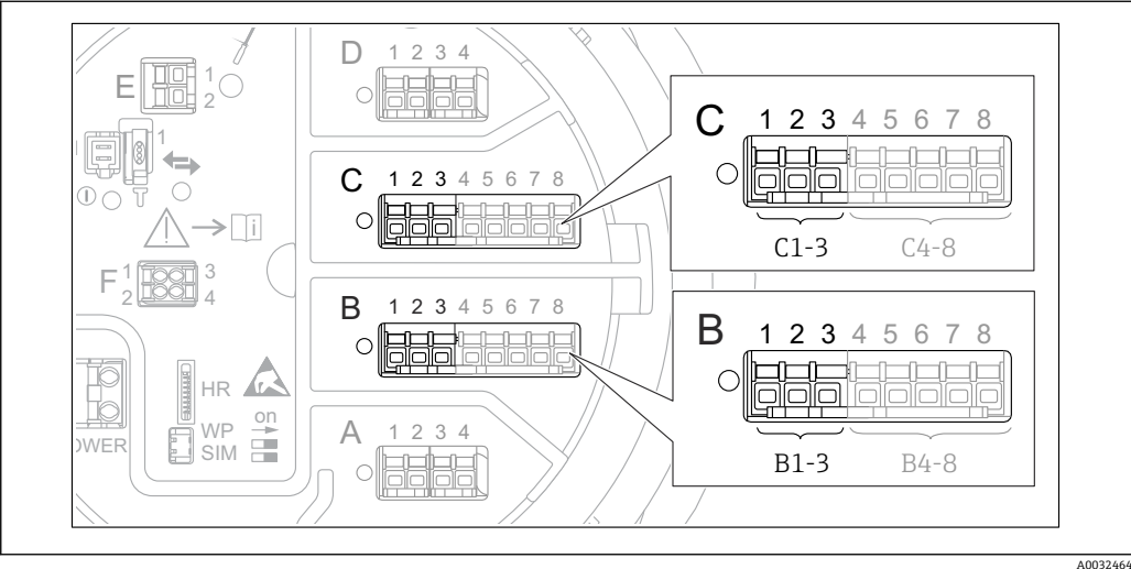
50 “Analog I/O” 子菜单的接线端子（分别为“B1-3”或“C1-3”）
