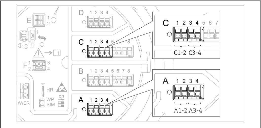
图 33 数字量输入/输出模块的可能安装位置（示例）；订货号确定数字量输入模块的数量和位置→ 图 20。
