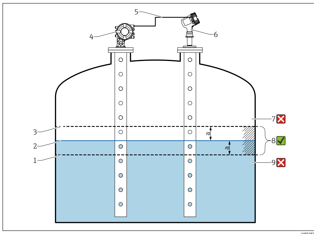
35 Proservo NMS8x 的应用实例
