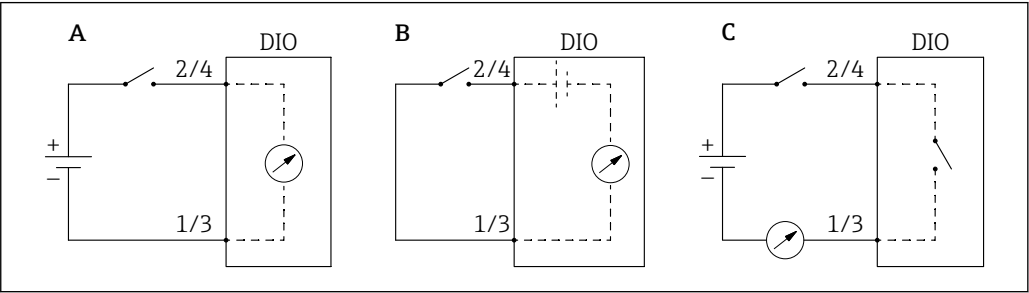
52 数字量输入/输出模块的工作模式
