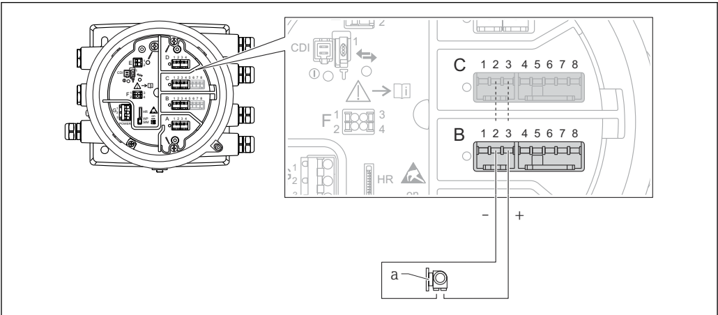
图 12 输入模式下的有源模拟量输入/输出模块
