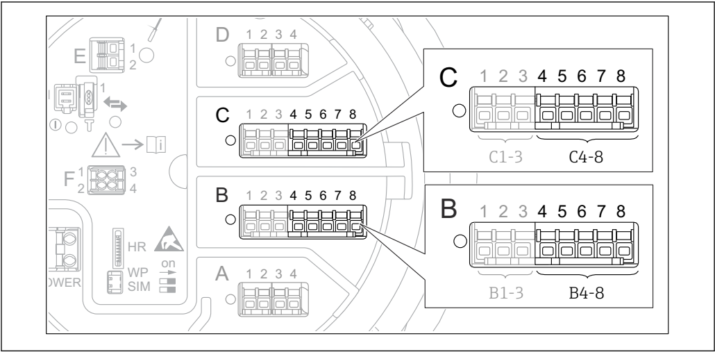
图 33 已连接 RTD 的模拟量输入/输出模块的可能安装位置。设备的订货号确定当前使用的模块 → 图 23。
