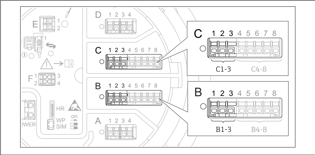
图 53 “Analog I/O” 子菜单的接线端子（分别为“B1-3”或“C1-3”）
