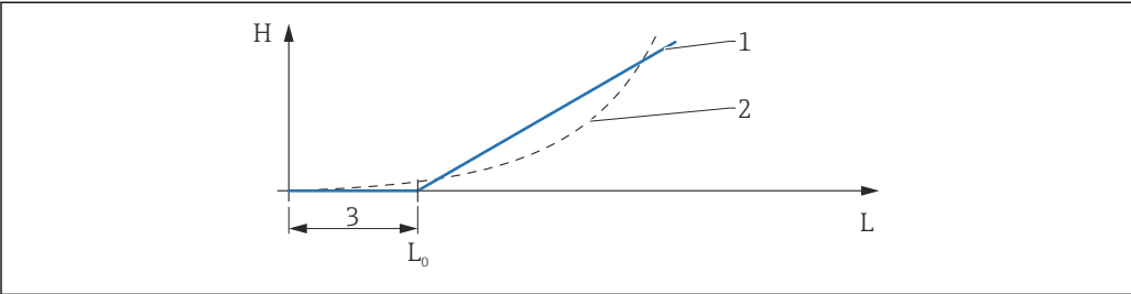
图 59 计算 HyTD 校正值
