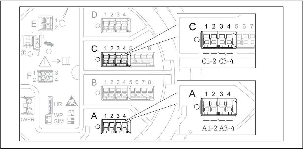
图 47 数字量输入/输出模块的可能安装位置 (实例)；订货号定义数字量输入/输出模块的数量和位置 → 图 23。
