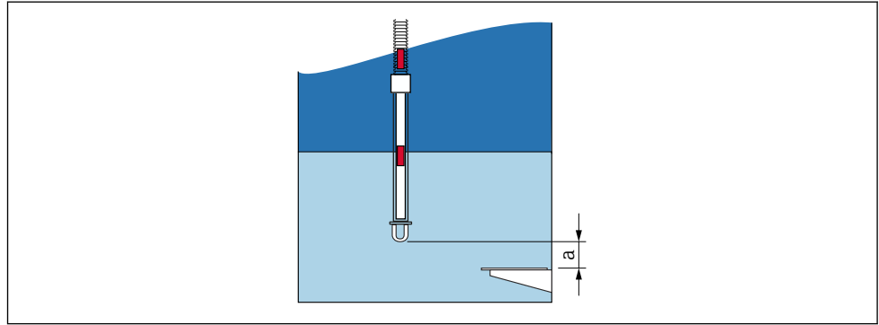
图 30 Prothermo NMT8x: 探头物理末端与零点位置之间的距离
