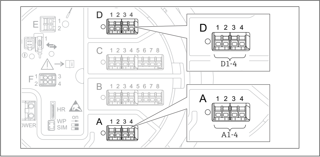
图 46 WM550 模块的可能安装位置 (实例)；取决于设备型号，上述模块还可以安装在插槽 B 或 C 中→ 图 23。
