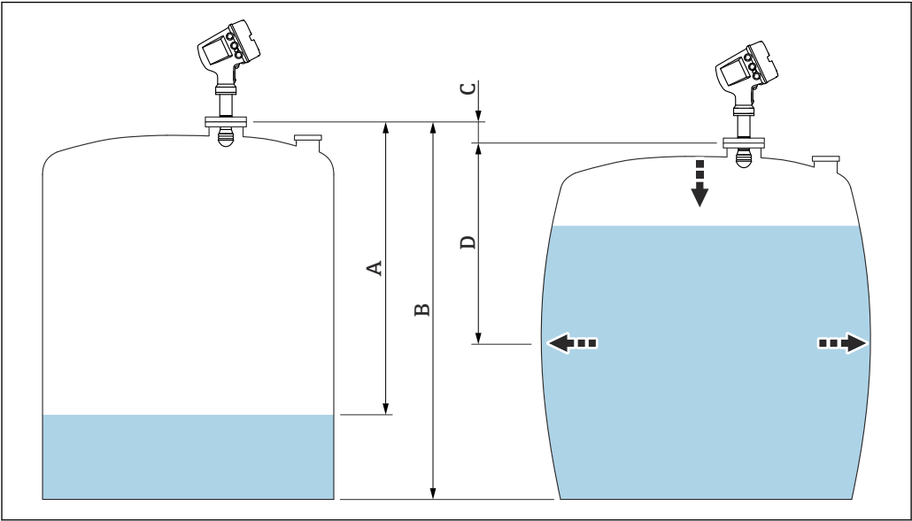
图 36 静压式储罐变形校正值（HyTD）
