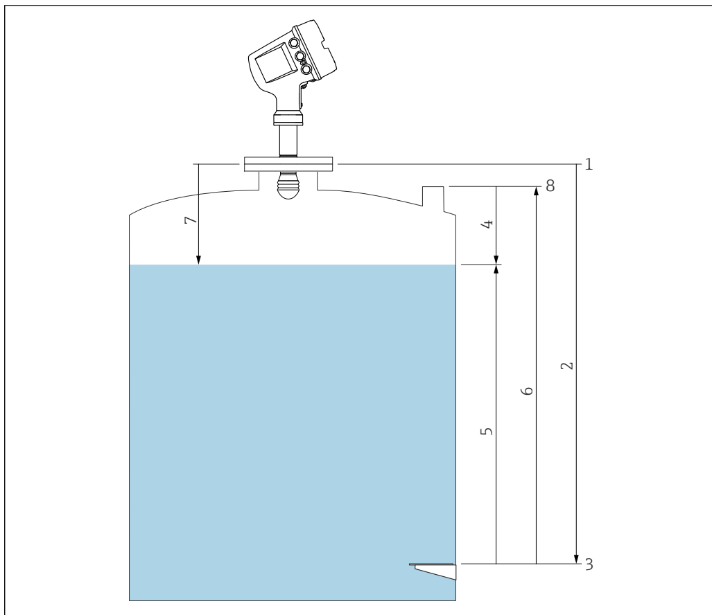
图 27 雷达罐体测量术语
