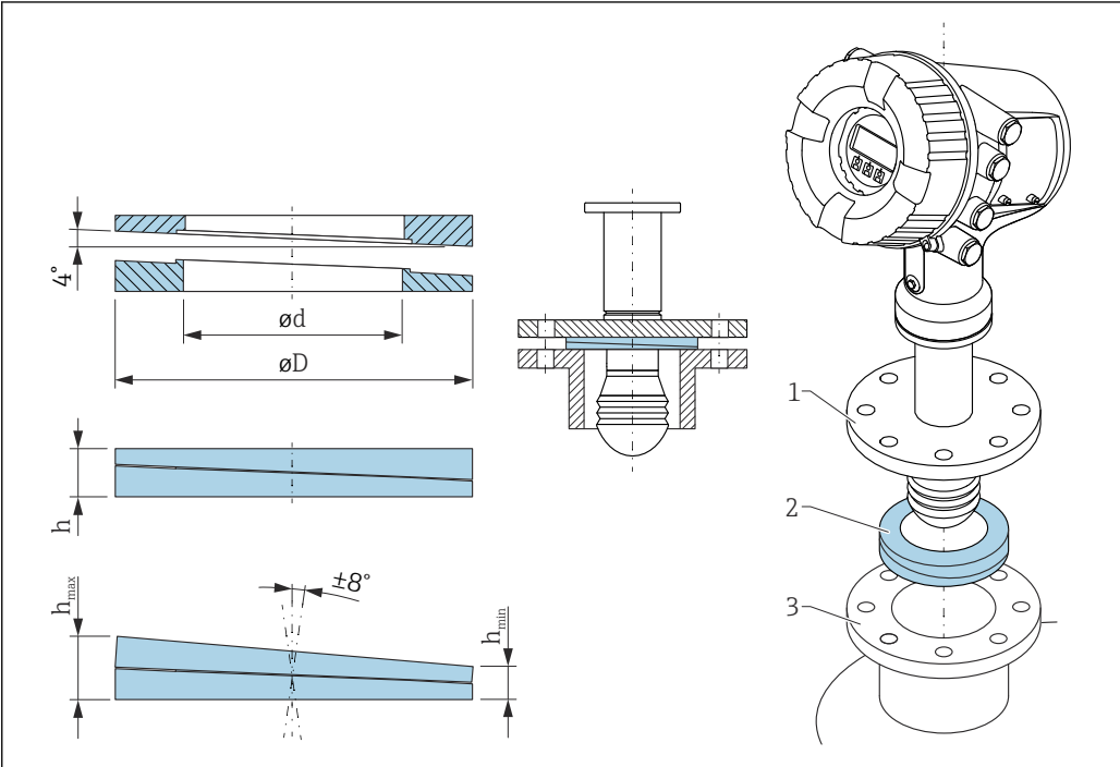
图 4 可调角度密封圈用于调节天线位置，角度调节范围为±8°
