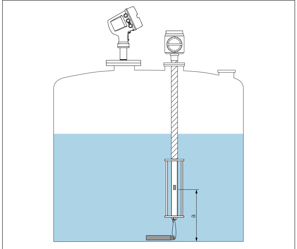
图 29 Prothermo NMT53x: 罐底测温元件位置
