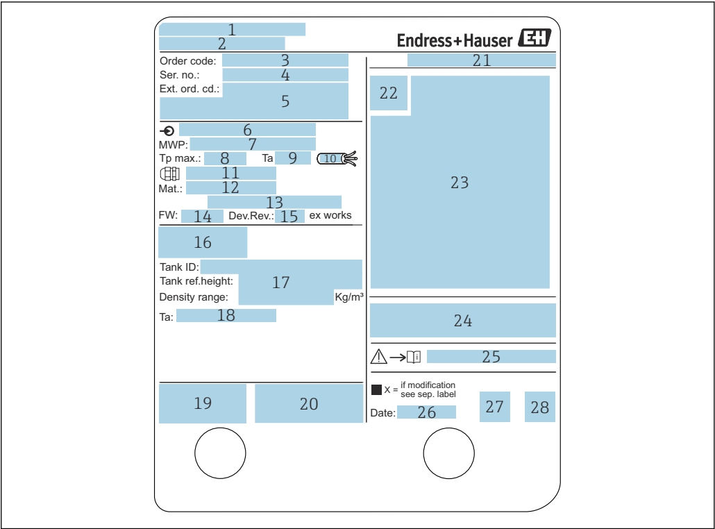
图 2 铭牌
