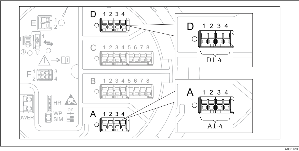
图 57 “Modbus”、“V1”或“WM550”模块名称实例; 取决于设备型号, 上述模块可以安装在插槽 B 或插槽 C 中。
