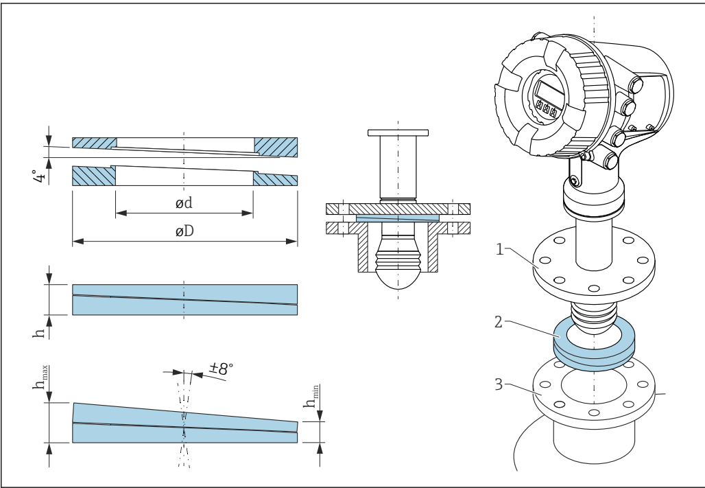
51 可调角度密封圈用于调节天线位置，角度调节范围为 \pm 8^\circ
