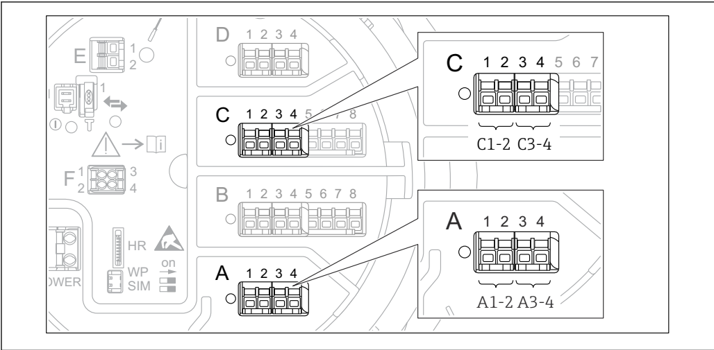
图 35 数字量输入/输出模块的可能安装位置 (示例) ; 订货号确定数字量输入模块的数量和位置→ 23。
