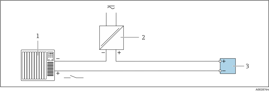
16 接线实例：状态输入 1 自动化系统，带状态输出（例如 PLC） 2 电源 3 变频器
