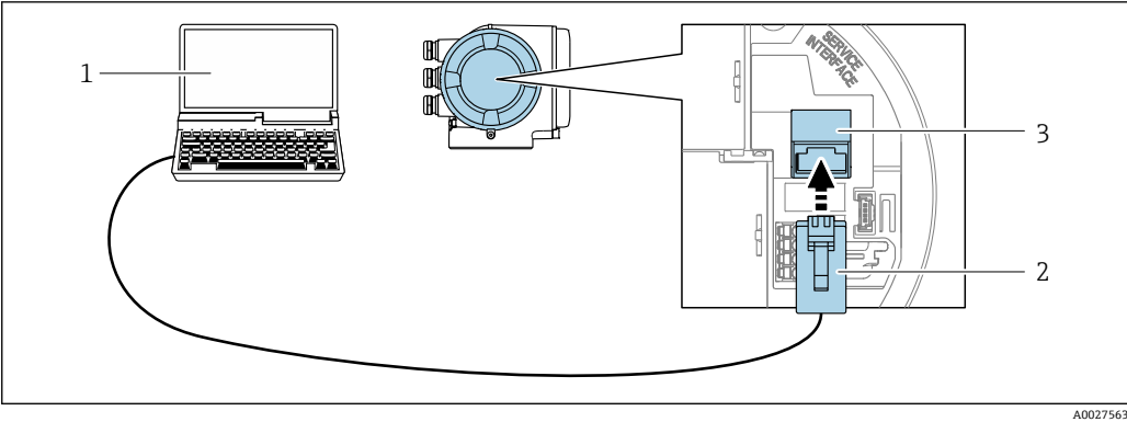
图 22 通过服务接口（CDI-RJ45）连接
