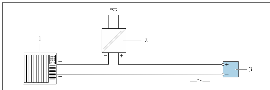
图 14 接线实例：继电器输出（无源信号）
