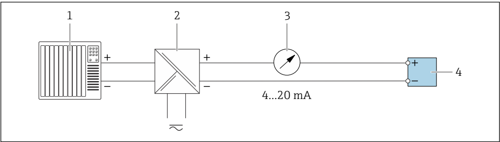
图 11 接线实例：4...20 mA 电流输出（无源信号）
