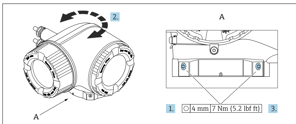
图 8 防爆型外壳
