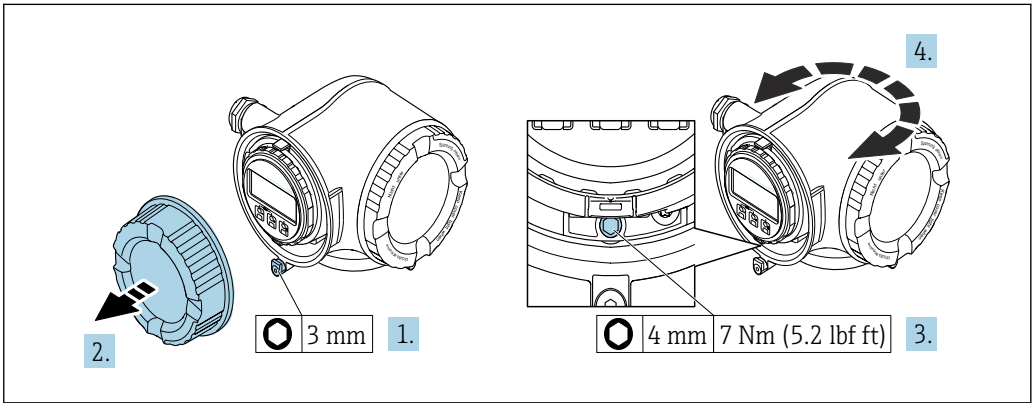
7 非防爆型外壳
