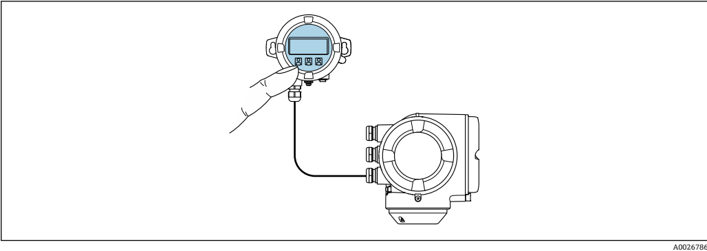
图 33 通过远传显示单元 DKX001 操作
