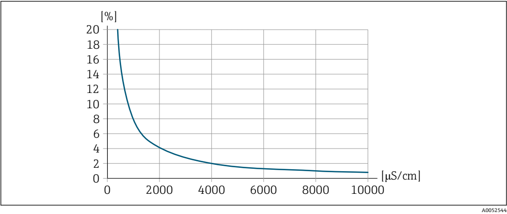
图 35 重复性 (测量值百分比) - 电导率 [µS/cm]
