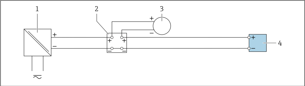
18 接线实例：4...20 mA 电流输入
