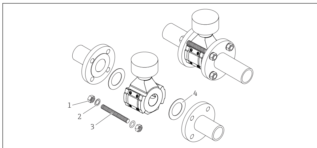
图 6 安装传感器
