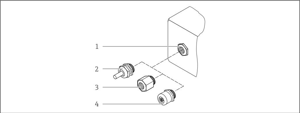
图 36 允许的电缆入口/缆塞 1 M20 × 1.5 内螺纹 2 M20 × 1.5 缆塞 3 转接头，适用于 G ½"或 NPT ½"内螺纹电缆入口 4 设备插头
