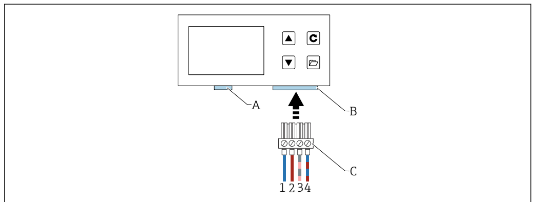
图 16 连接分离型显示单元
