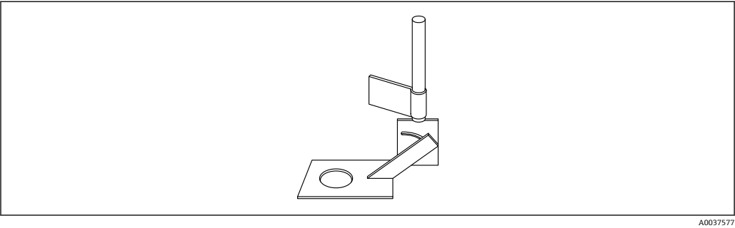
23 通用安装支座（1.4301 材质），配备倾转装置和固定头，传感器开孔直径 \varnothing 108 mm (4.25 in)
