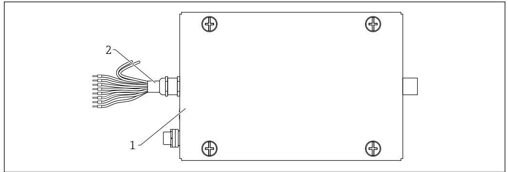
图 15 ATEX 防爆型电子部件腔：10 针电缆的接线端子分配
