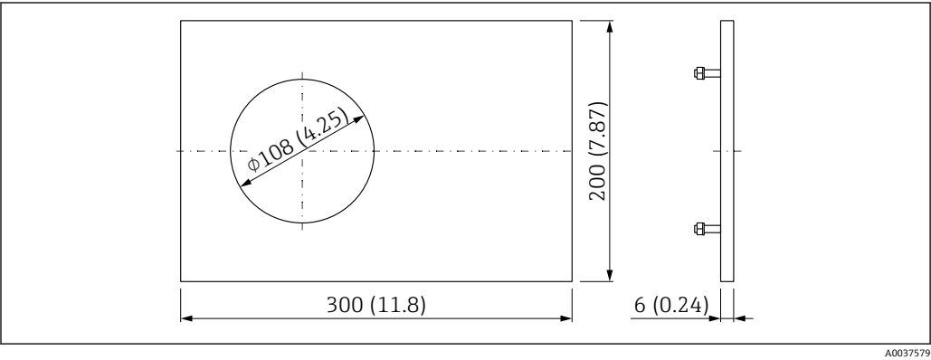
22 挡板，1.4301，传感器开孔 \varnothing 108 mm (4.25 in)。测量单位 mm (in)
