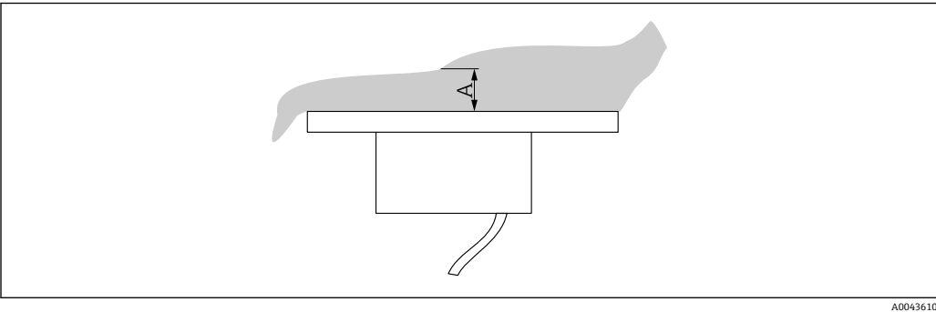
图 27 传感器顶部的物料高度
