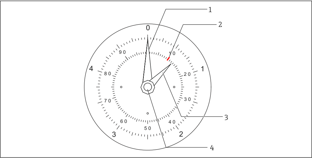
图 55 刻度盘显示 (5 m (16.4 ft) 刻度板)
