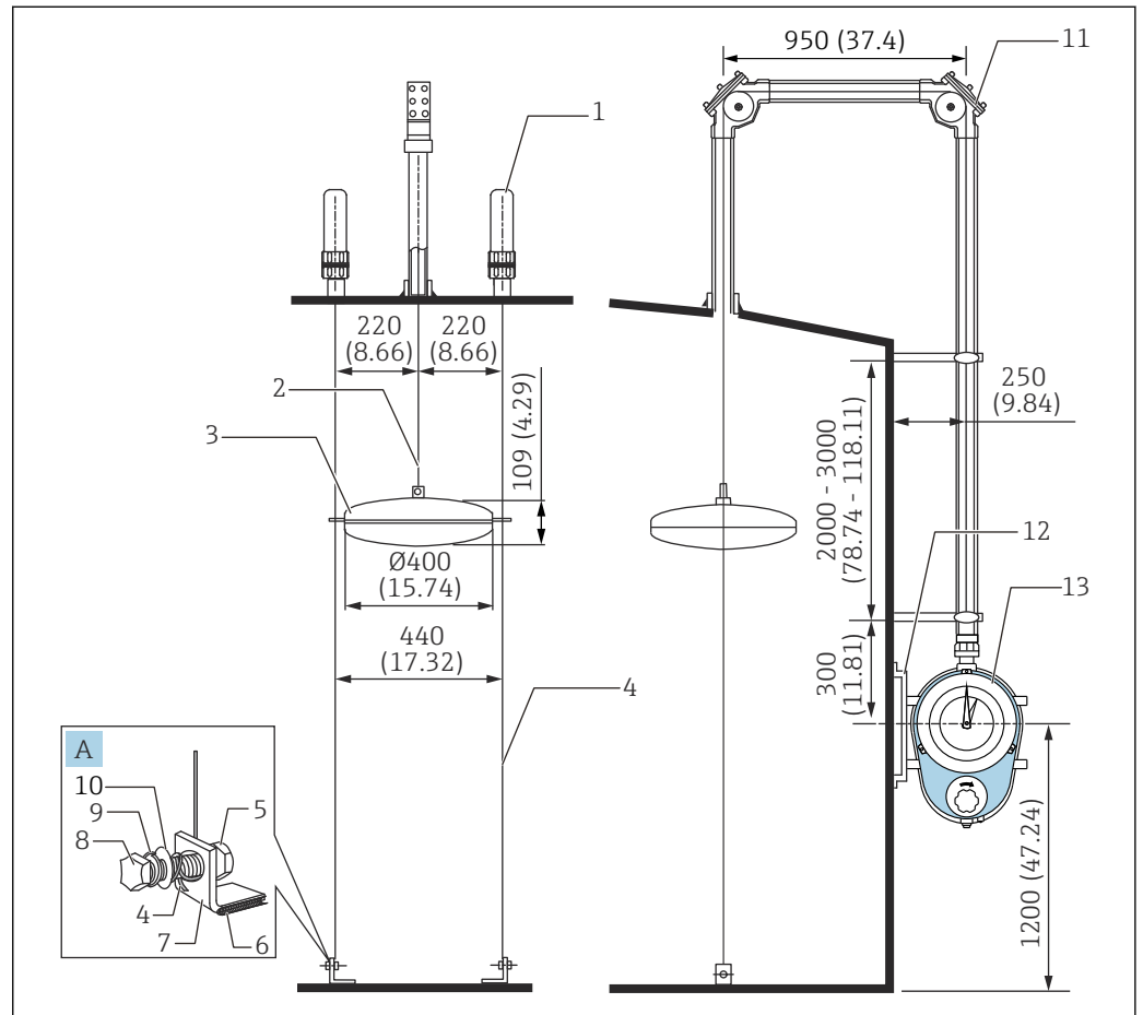
27 在锥顶罐体上安装。测量单位 mm (in)
