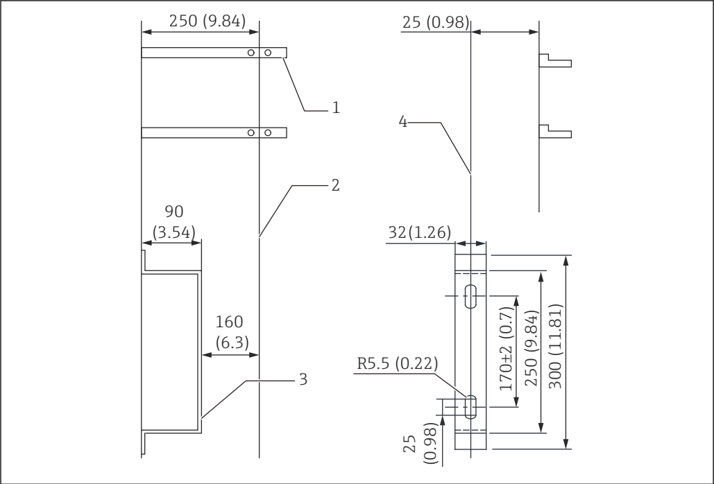
69 仪表支架（针对低压型/中压型）。测量单位 mm (in)
