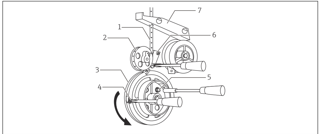
图 45 LT 部件
