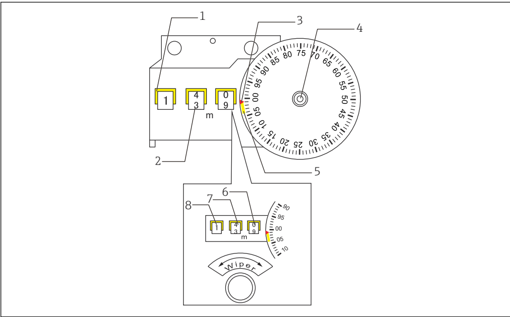
图 56 计数器显示
