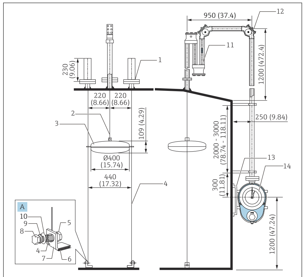
图 29 安装用于锥顶罐体的密封罐。测量单位 mm (in)
