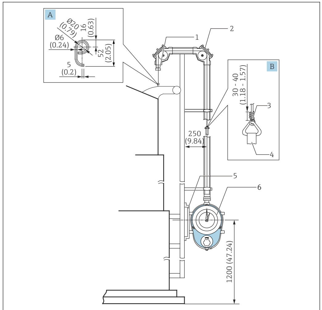
图 33 安装储气罐。测量单位 mm (in)
