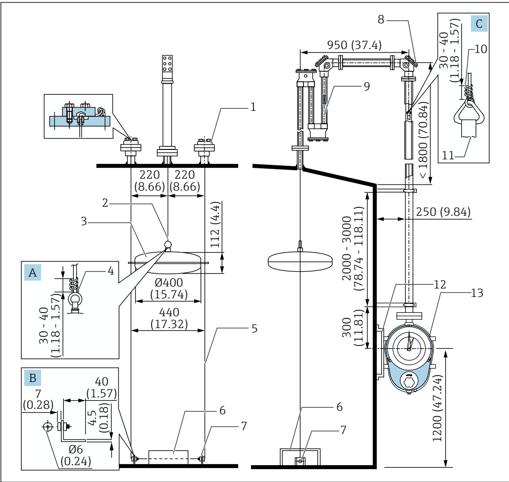
图 30 安装用于锥顶罐体的 PVC 密封罐。测量单位 mm (in)
