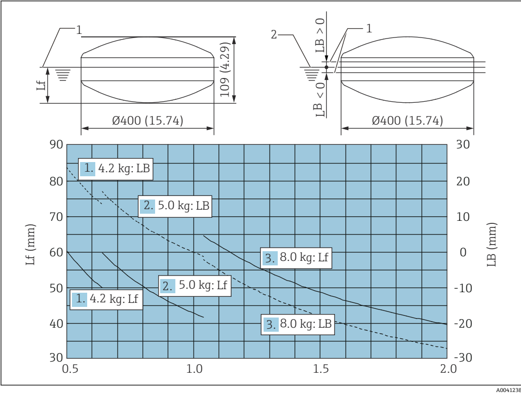
图 58 LT5-1 φ400 mm (15.75 in)浮子的图示：被测液体的密度 ρ (g/cm³)。测量单位：mm (英寸)
