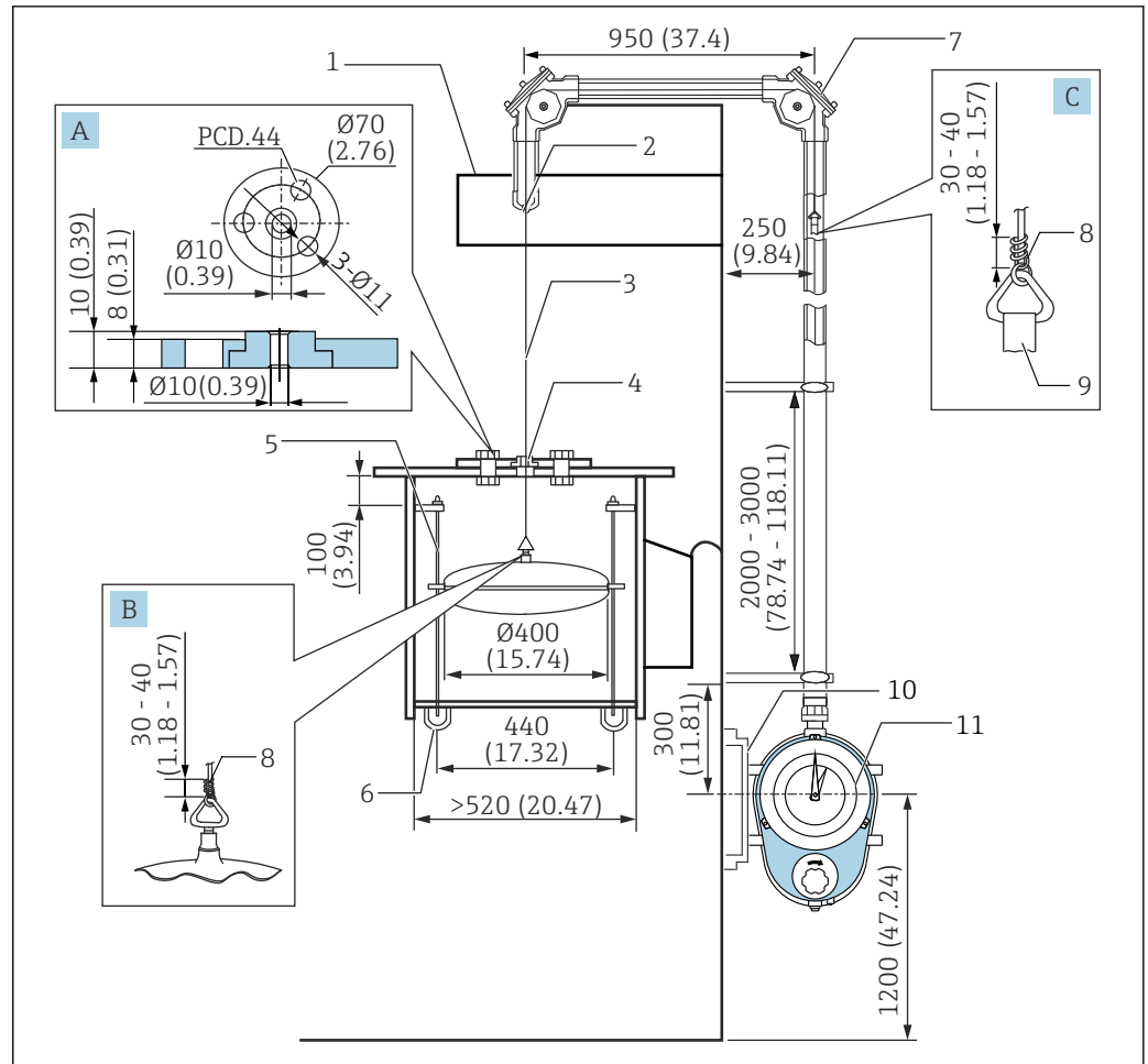
43 安装测量带。测量单位 mm (in)
