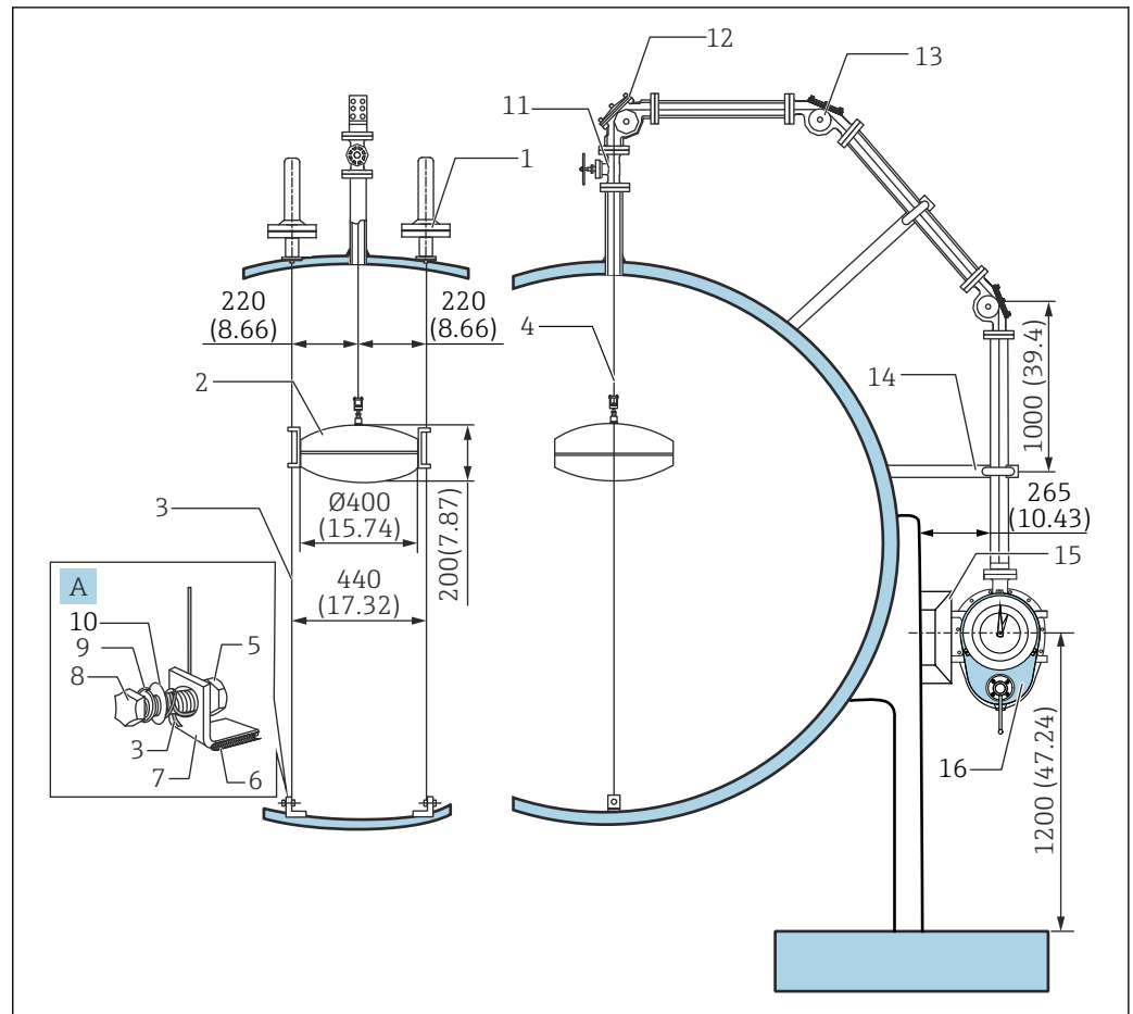
36 安装在高压球罐上。测量单位 mm (in)
