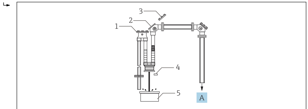
图 53 排放液体密封剂
