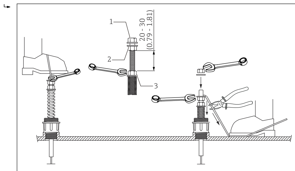
38 导丝安装 2。测量单位 mm (in)
