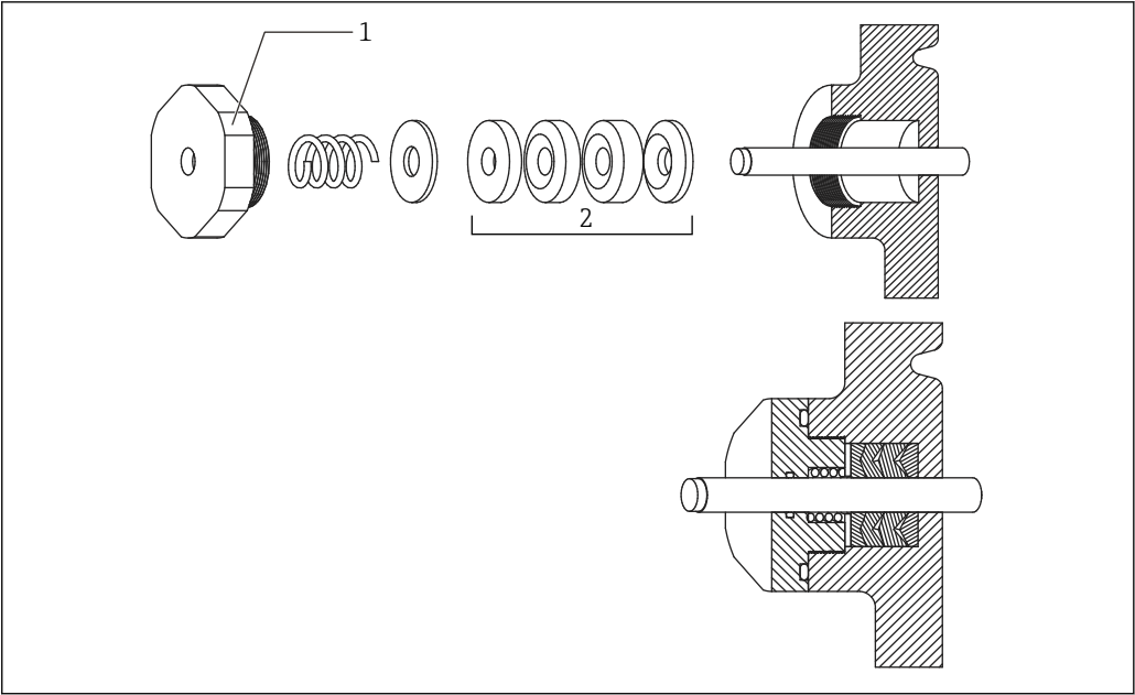
图 67 检查手柄装置
