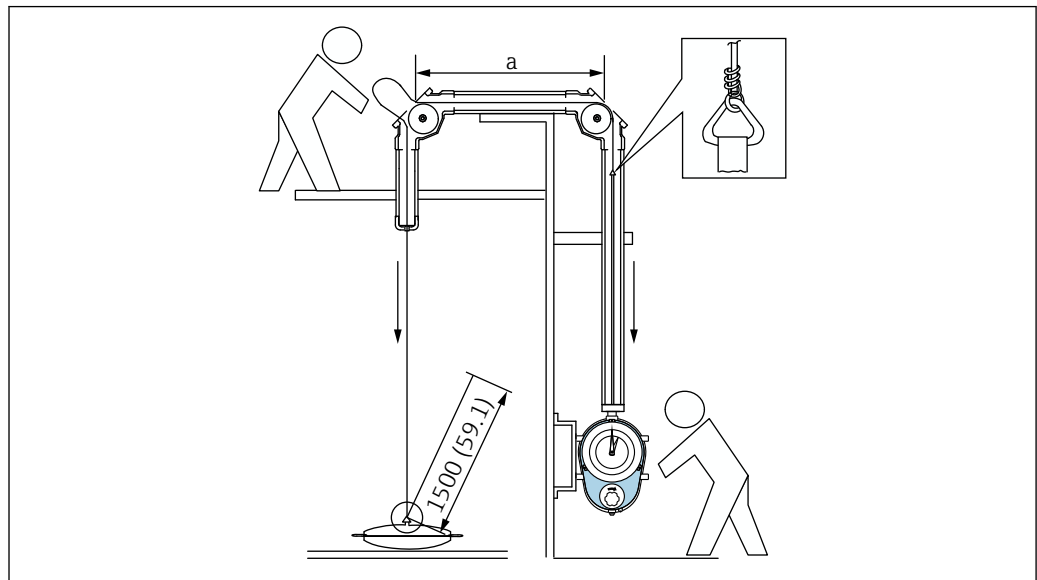
图 41 安装测量带和测量导丝：测量带 + 测量导丝。测量单位 mm (in)
