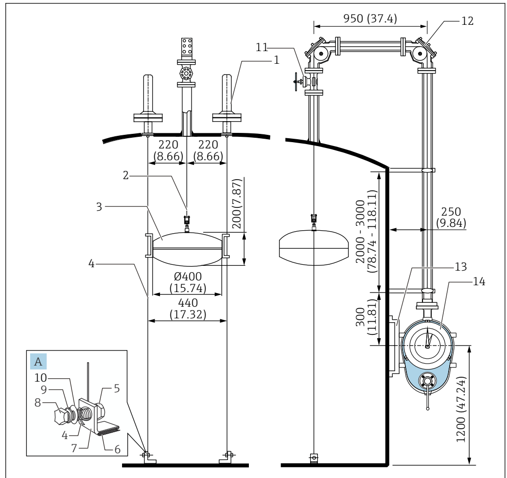
35 在中压拱顶罐体上安装。测量单位 mm (in)
