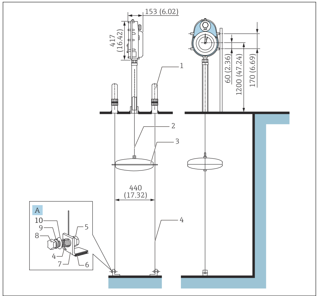
图 28 在地下罐上安装。测量单位 mm (in)
