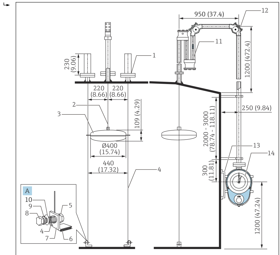
图 50 带密封罐的 LT。测量单位 mm (in)
