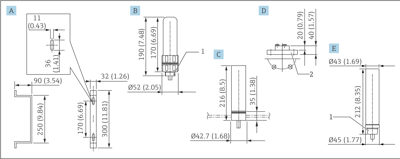
图 4 附件 1。测量单位 mm (in)
