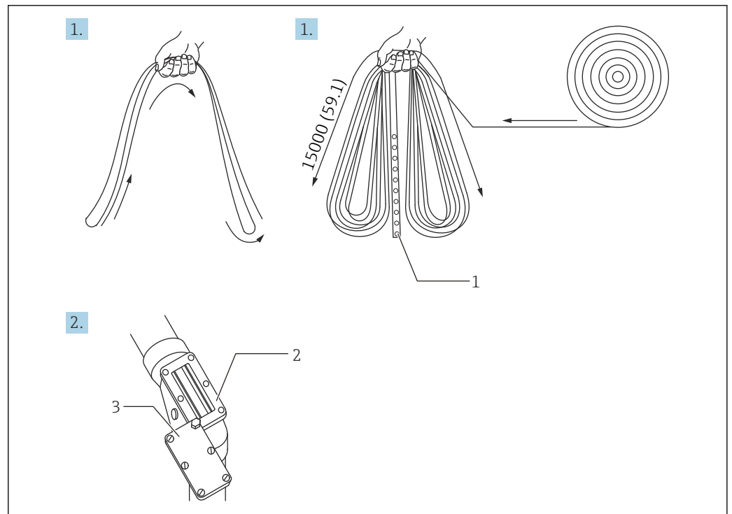
图 39 测量带准备。测量单位 mm (in)
