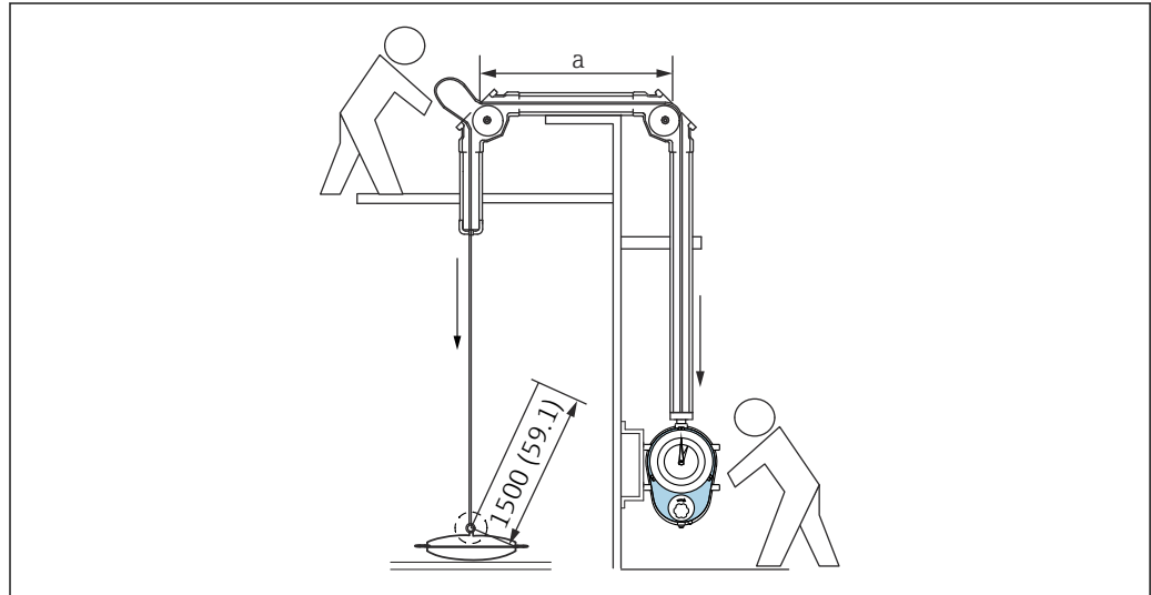
图 40 安装测量带：测量带。测量单位 mm (in)
