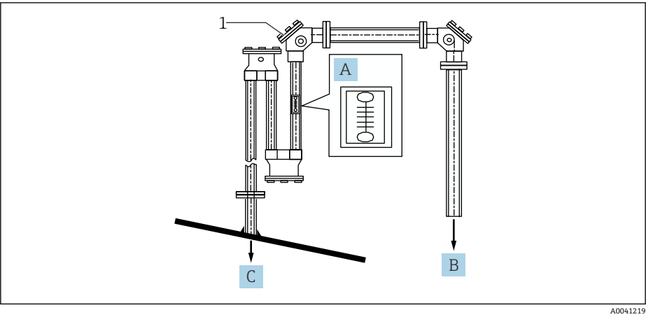
51 加注液体密封剂 A 液体密封剂的刻度 B 至 LT5 侧 C 至罐体内部 1 90°滑轮弯头
