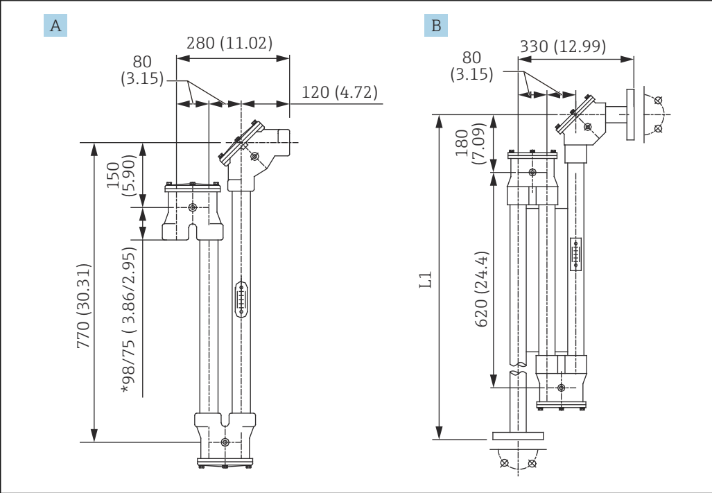
68 密封罐。测量单位 mm (in)
