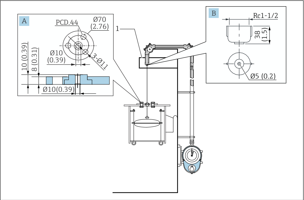
73 导丝金属导向装置、导丝导向装置插口。测量单位 mm (in)
