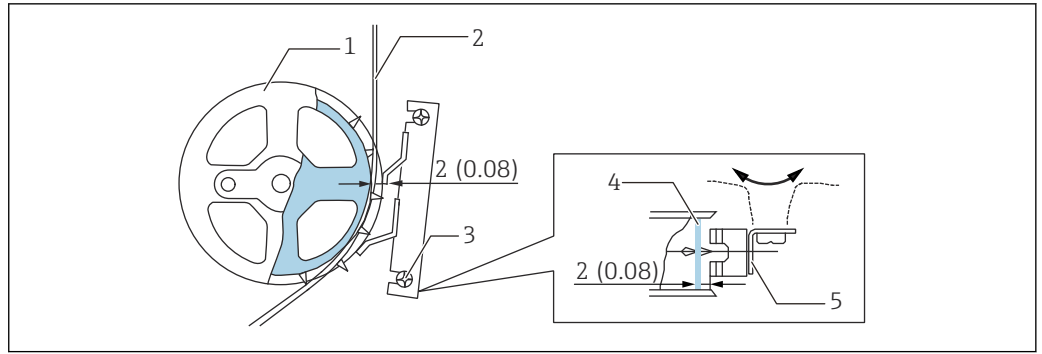
48 测量带导向装置调节。测量单位 mm (in)
