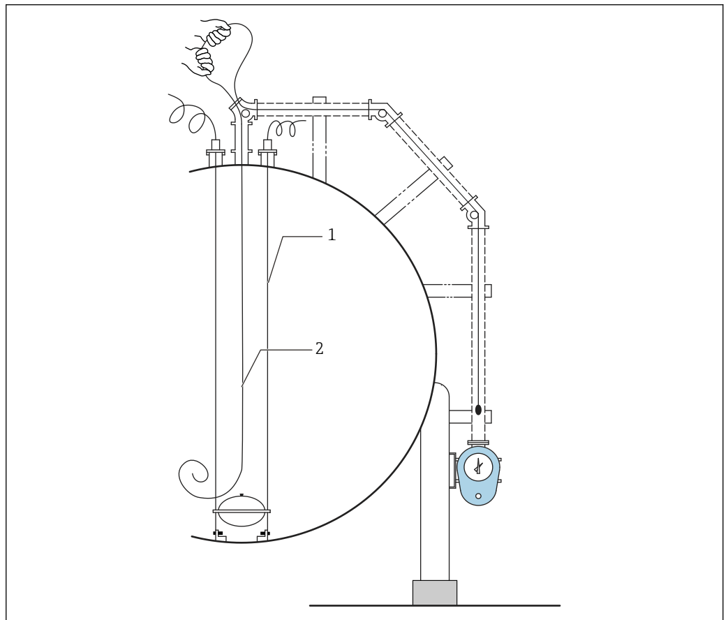
图 46 安装测量带
