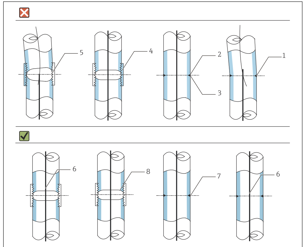
图 24 连接导管
