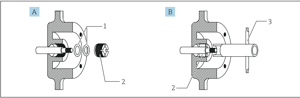
44 压盖固定工具
