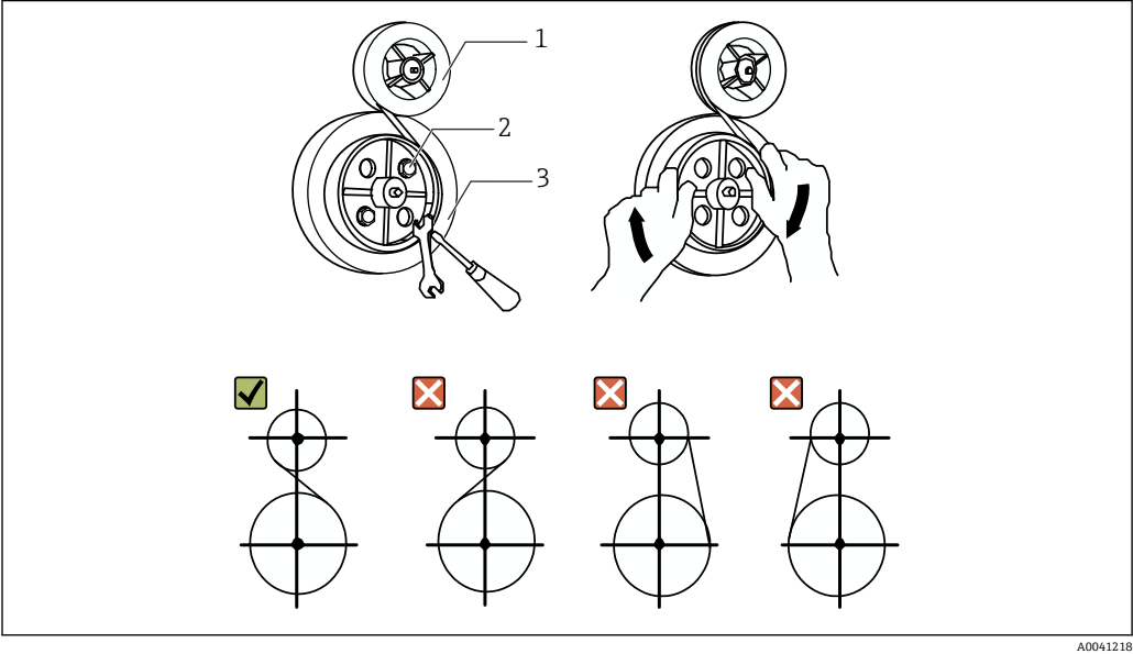
图 49 安装康斯特仪表
