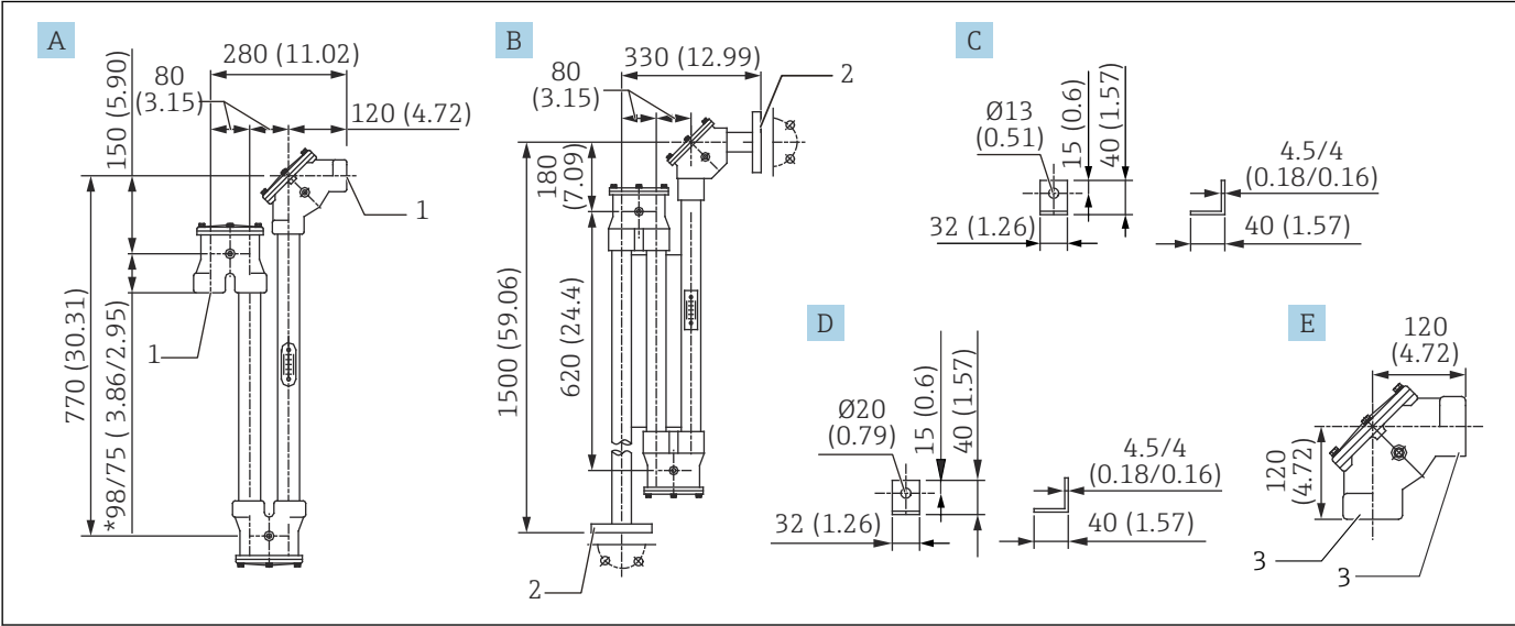
图 5 附件 2。测量单位 mm (in)
