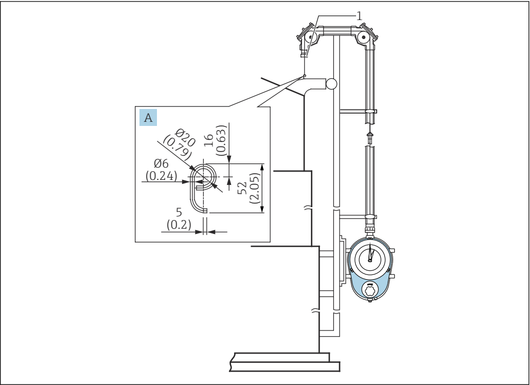
74 导丝钩和导丝导向装置插口。测量单位 mm (in)
