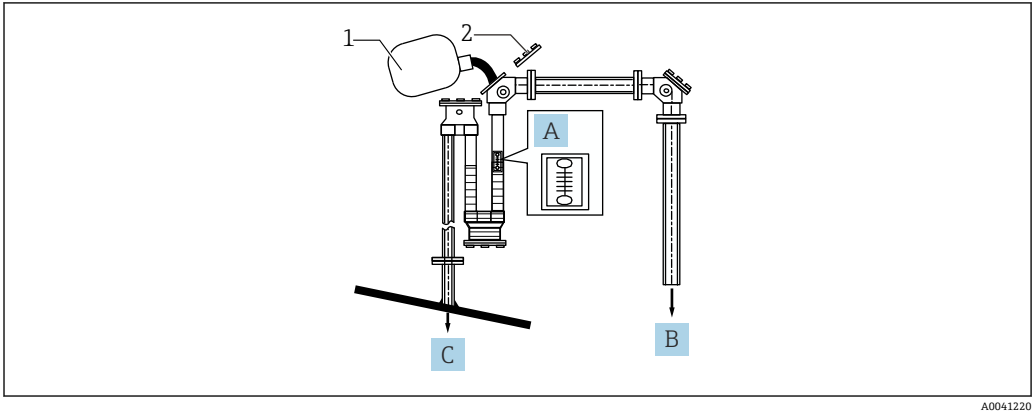
52 液体密封剂量 A 液体密封剂的刻度 B 至 LT5 侧 C 至罐体内部 1 液体密封剂 2 90°滑轮弯头盖板
