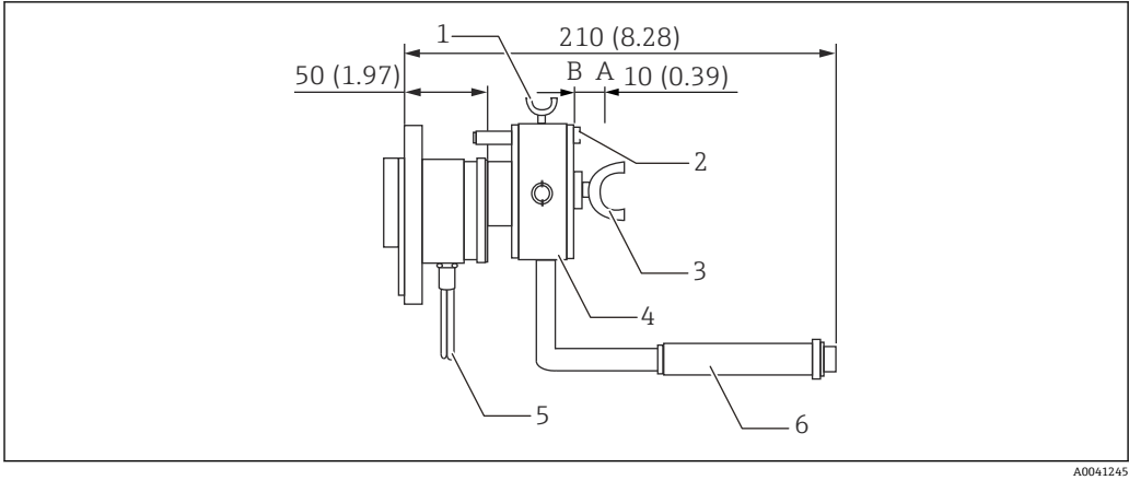
图 63 处理提升手柄 (LT5-1) 。 测量单位 mm (in)
