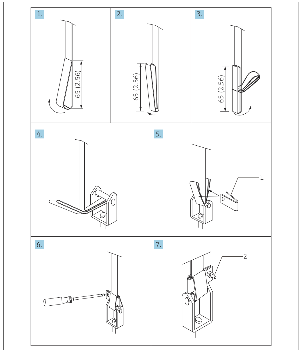
图 42 测量带和浮子的连接。测量单位 mm (in)
