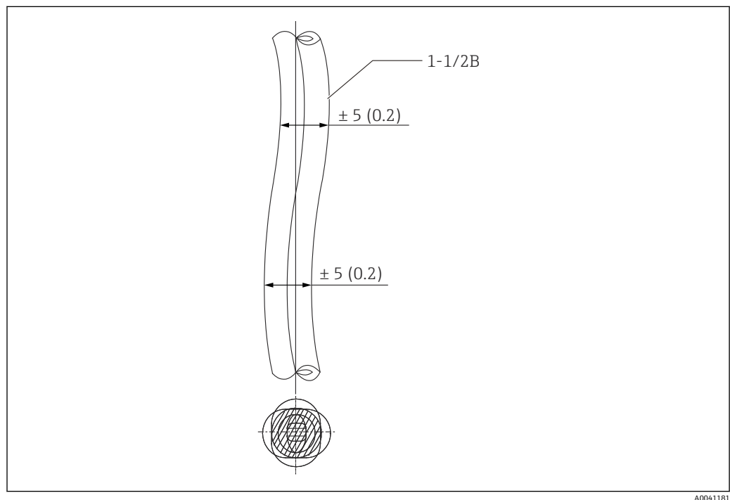
图 23 安装导管。测量单位 mm (in)
