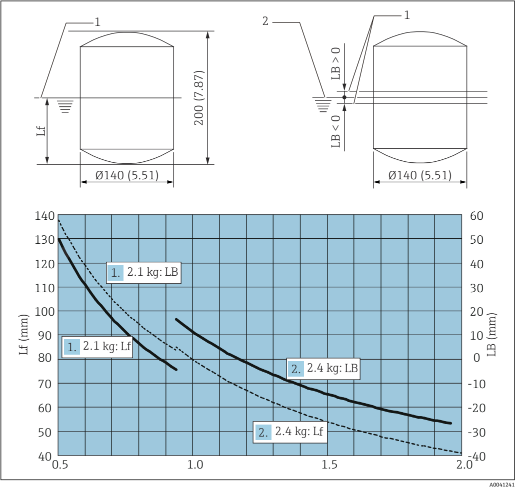
59 罐体中注满水时的指示仪数值。测量单位: mm (英寸)
