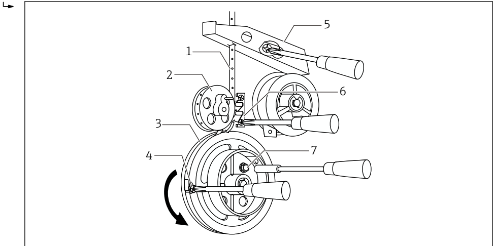
图 47 带轮
