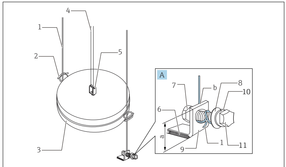
图 37 导丝安装 1
