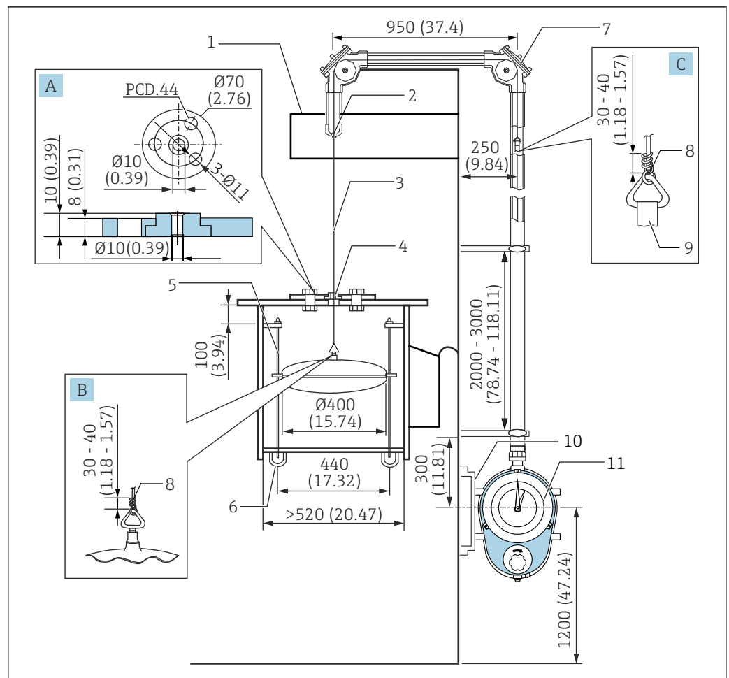
图 34 在浮顶罐体上安装。测量单位 mm (in)
