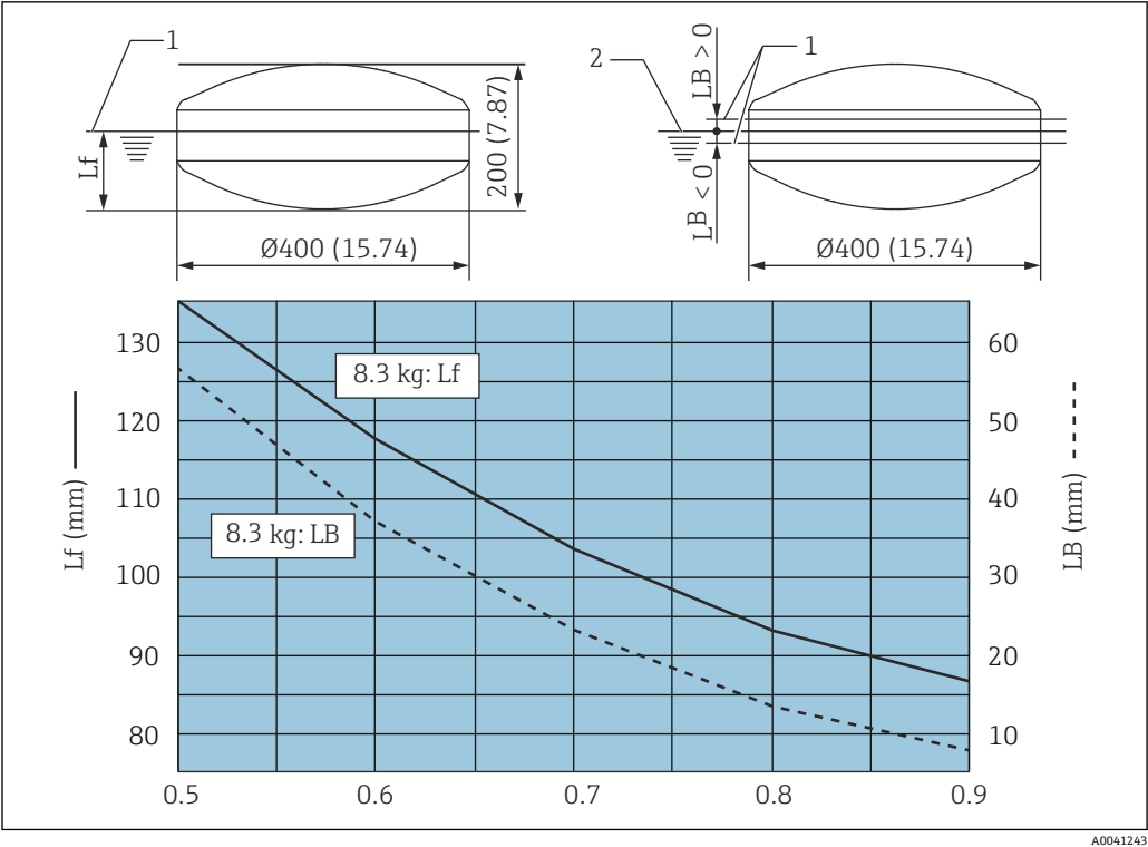
图 60 LT5-4/LT5-6 \text{Ø}400 \text{ mm} (15.75 in)浮子的图示: 被测液体的密度 \rho ( \text{g/cm}^3 )。测量单位: mm (英寸)
