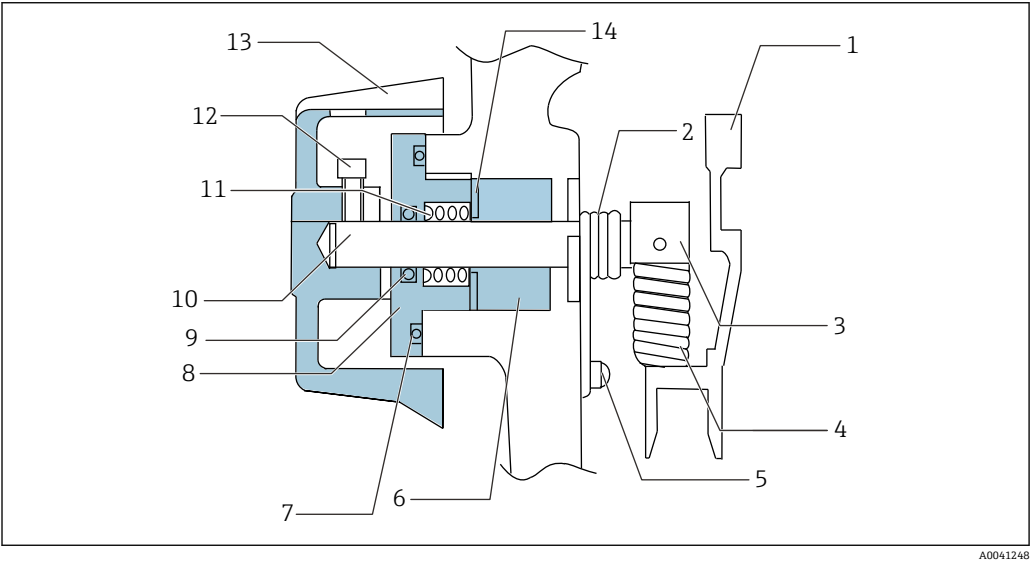
图 66 检查手柄装置各部分名称
