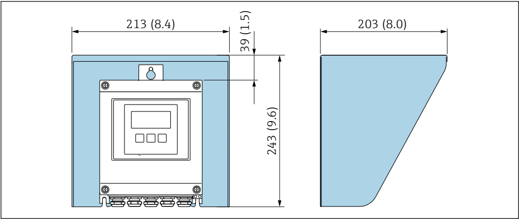
18 Proline 500（数字）变送器的防护罩；单位：mm (in)
