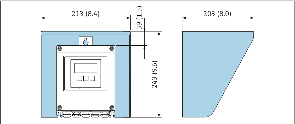
图 37 Proline 500（数字）变送器的防护罩；单位：mm (in)
