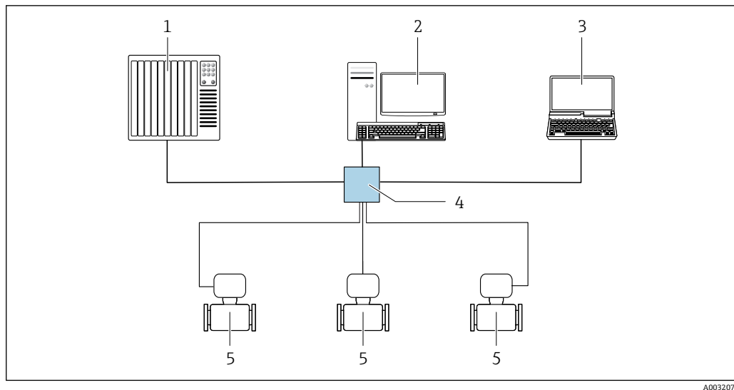
图 51 通过 EtherNet/IP 网络进行远程操作：星形拓扑结构
