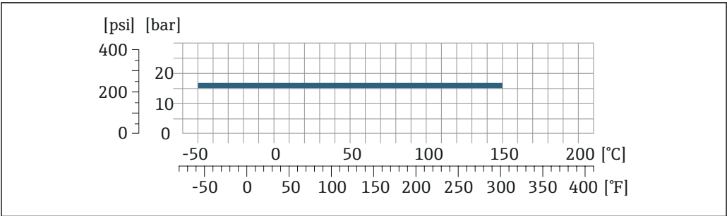
图 27 连接部件材质：二级钛材
