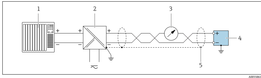
图 10 接线实例：4 ... 20 mA HART 电流输出（无源）
