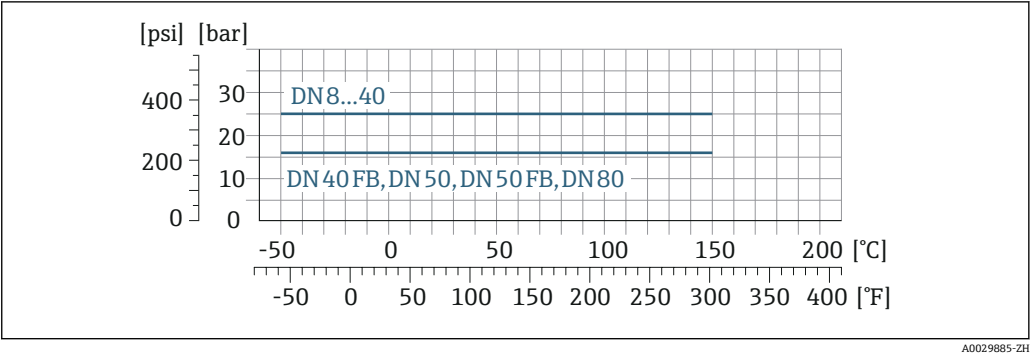
24 法兰材质：二级钛材
