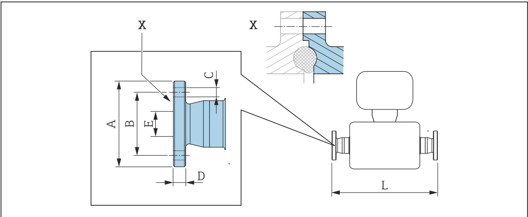
图 30 部件 X: 非对称过程连接; 灰色部分由供应商提供。
