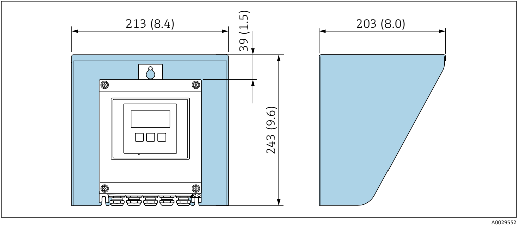
图 31 Proline 500 (数字) 变送器的防护罩; 单位: mm (in)
