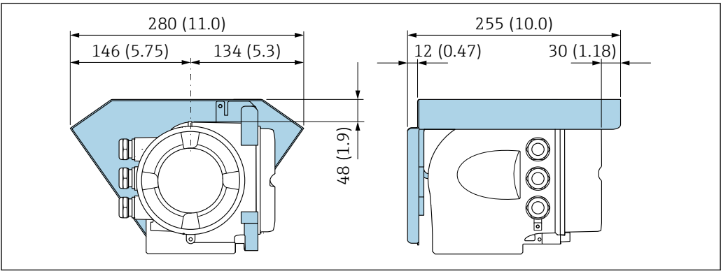
19 Proline 500 变送器的防护罩；单位：mm (in)
