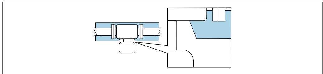
图 29 延长颈上无保温层覆盖
