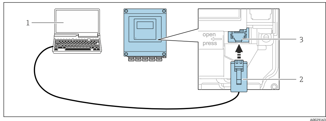
图 57 通过服务接口 (CDI-RJ45) 连接
