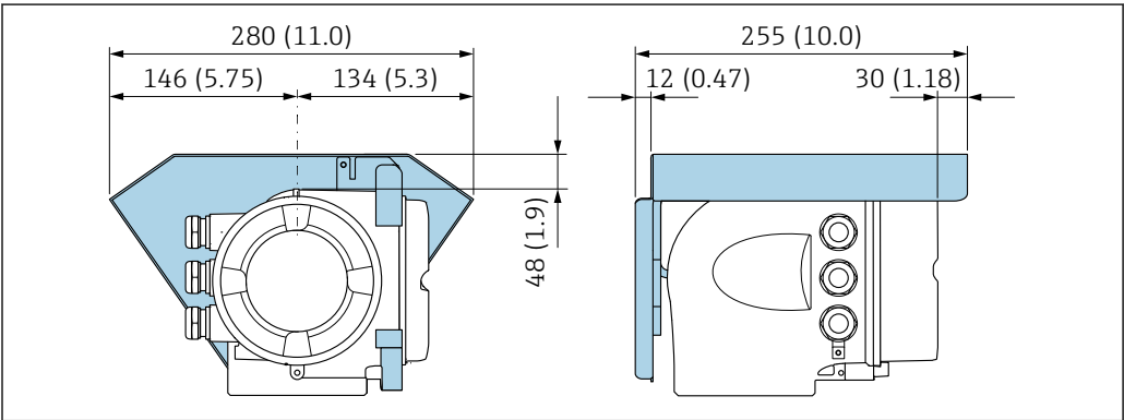
图 38 Proline 500 变送器的防护罩；单位：mm (in)
