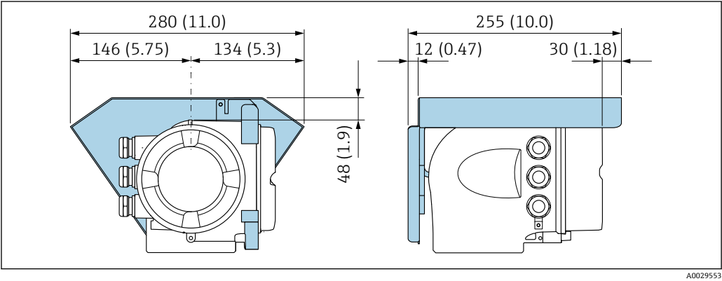
图 32 Proline 500 变送器的防护罩; 单位: mm (in)
