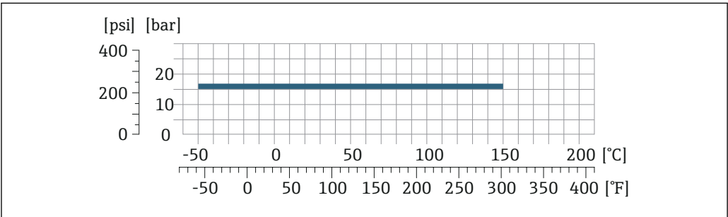
图 28 连接部件材质：二级钛材
