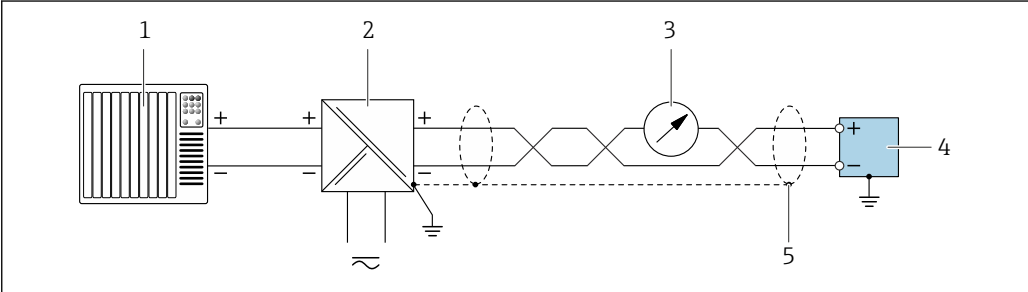
图 25 接线实例：4 ... 20 mA HART 电流输出（无源）
