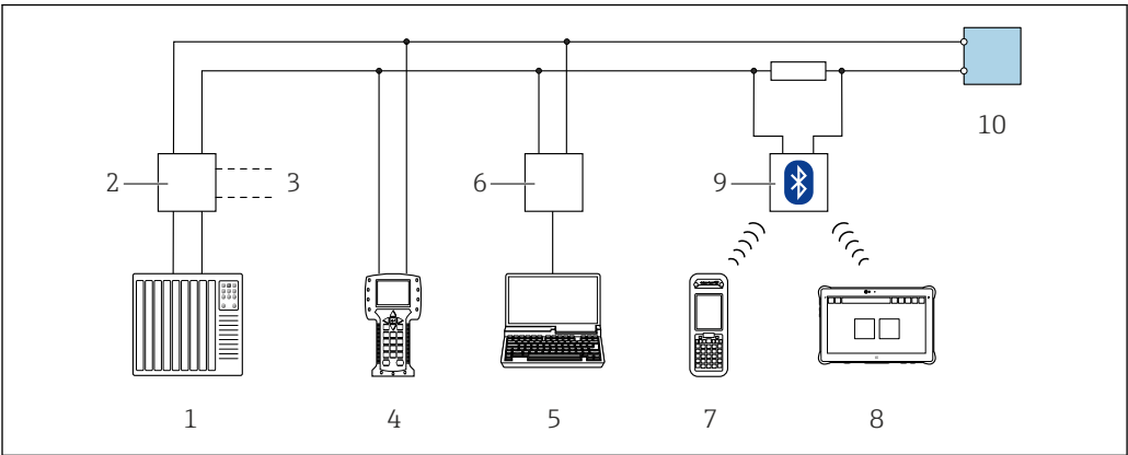
32 通过 HART 通信进行远程操作（无源信号）
