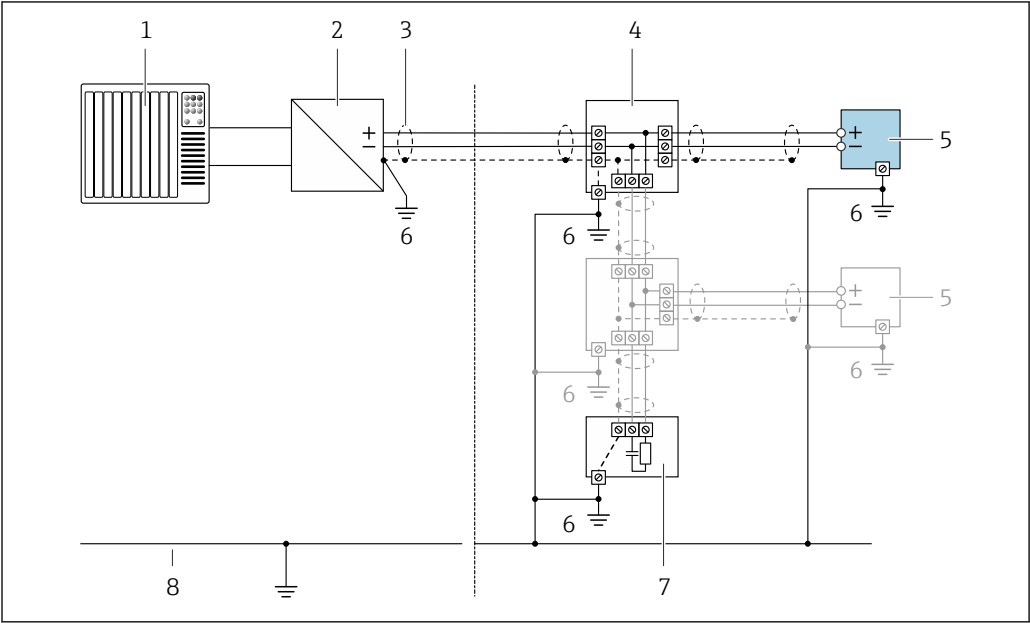
19 接线实例：PROFIBUS PA
