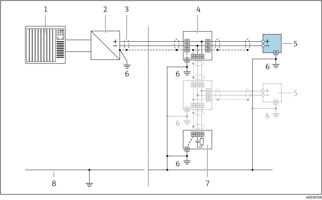
图 16 PROFIBUS PA 的接线实例
