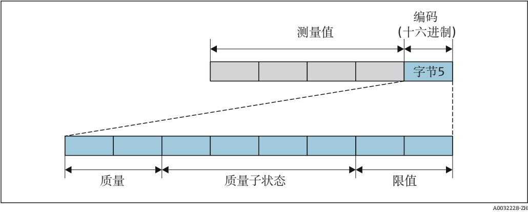
图 38 编码字节结构
