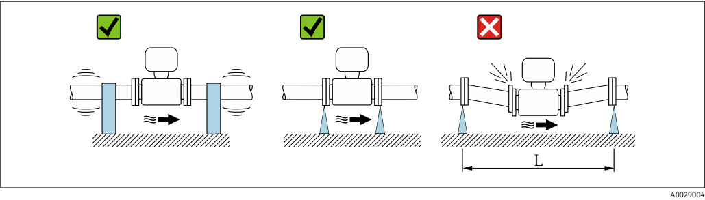
7 避免仪表振动的措施 ( L > 10\text{ m} (33 ft))
