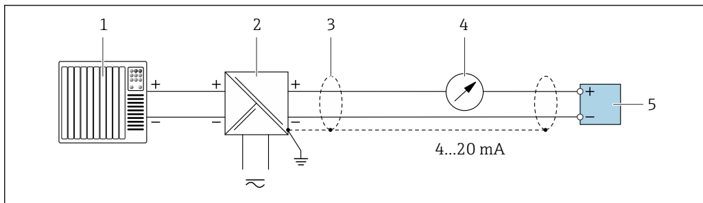
图 13 接线实例：4...20 mA HART 电流输出（无源信号）
