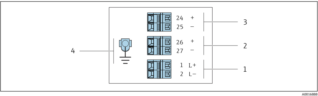
图 8 接线端子分配: 4...20 mA HART 或脉冲/频率/开关量输出
