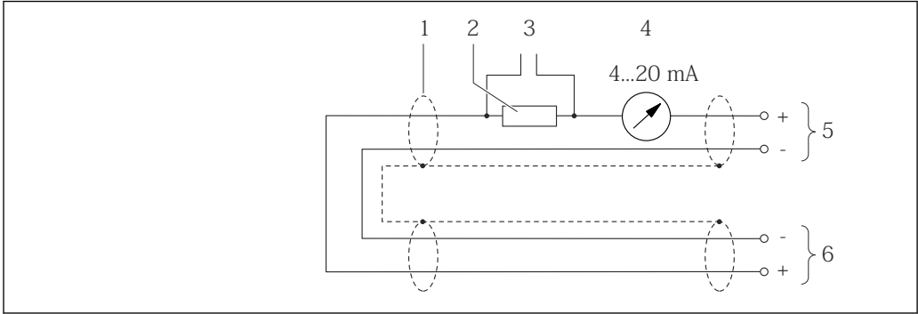
图 16 接线示例：HART 电流输入（burst 模式），HART 电流输出（有源信号）
