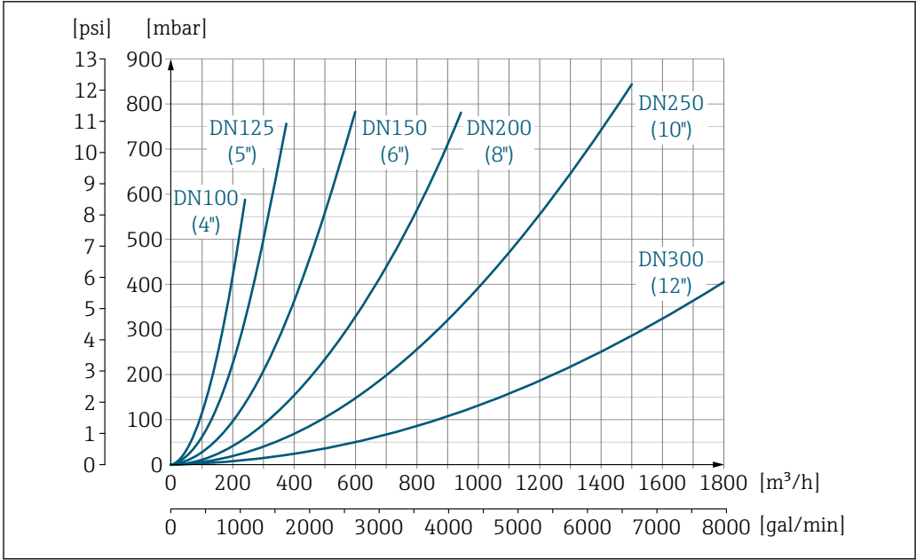
图 23 DN 100...300 (4...12")的压损 (订购选项“设计”，选项代号 C “短插入深度，符合 ISO/DVGW 标准 (最大适用口径为 DN 300)，测量管不带前后直管段”)
