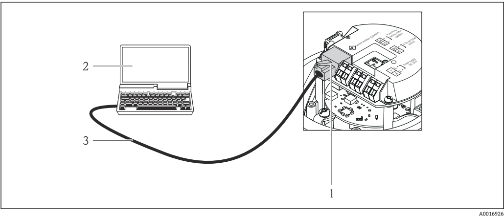
图 20 订购选项“输出”，选型代号 B: 4...20 mA HART，脉冲/频率/开关量输出
