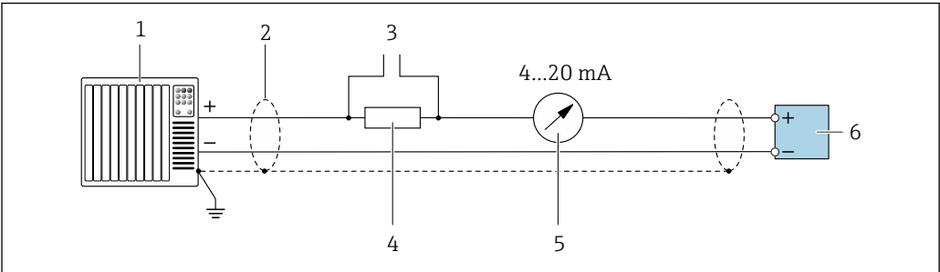
图 12 4...20 mA HART 电流输出（有源）的接线图
