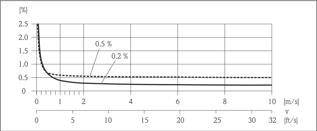
图 21 最大测量误差 (% o.r.)
