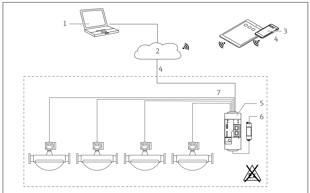
图 4 Fieldgate FXA42 的系统架构 (连接脉冲计数器)
