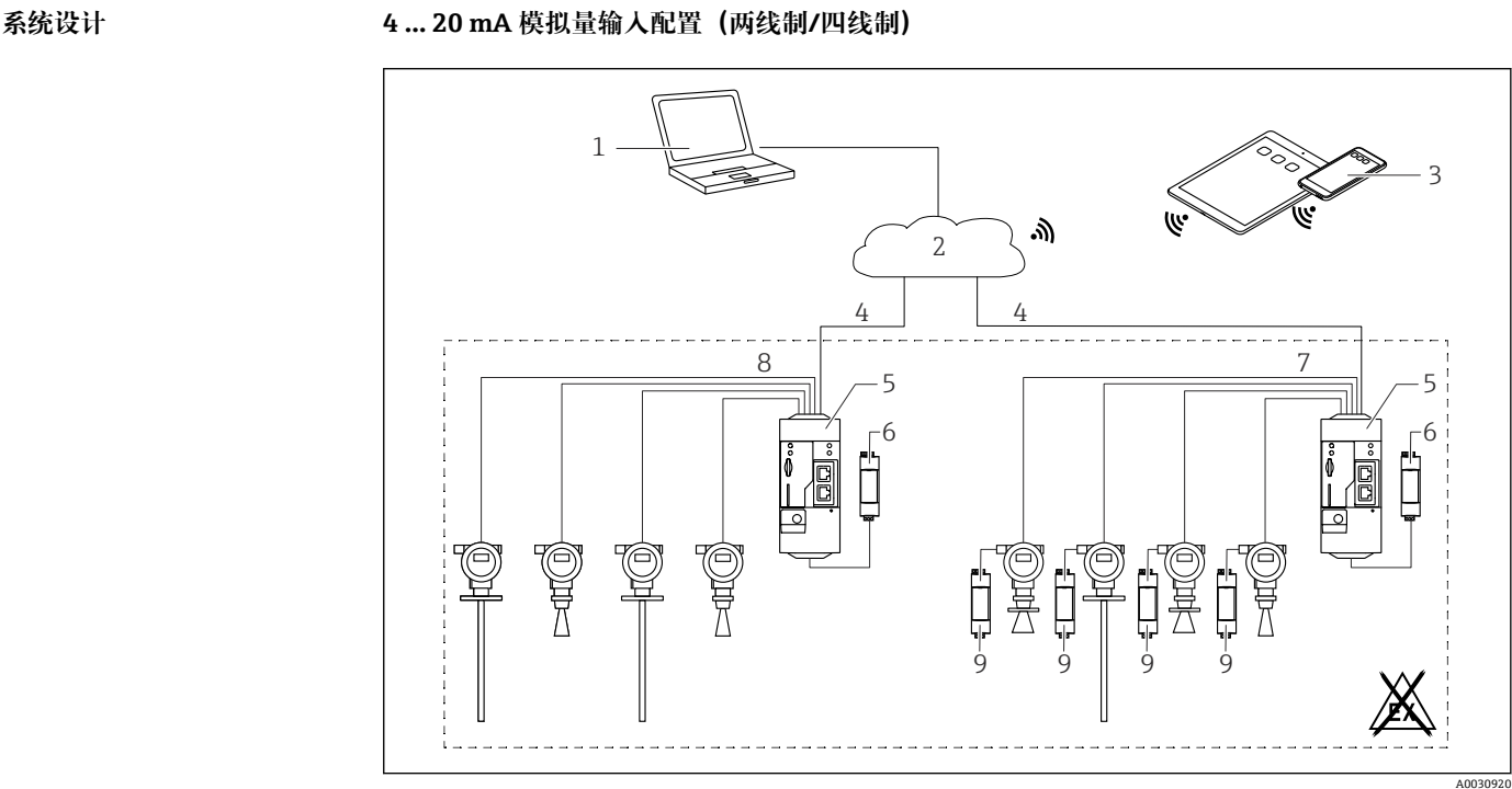
图 2 Fieldgate FXA42 系统架构 (带 4 ... 20 mA 模拟量输入)
