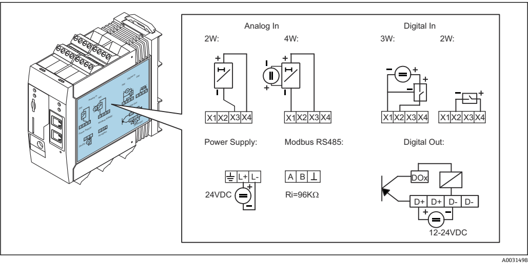
图 9 外壳上的接线端子分配标识
