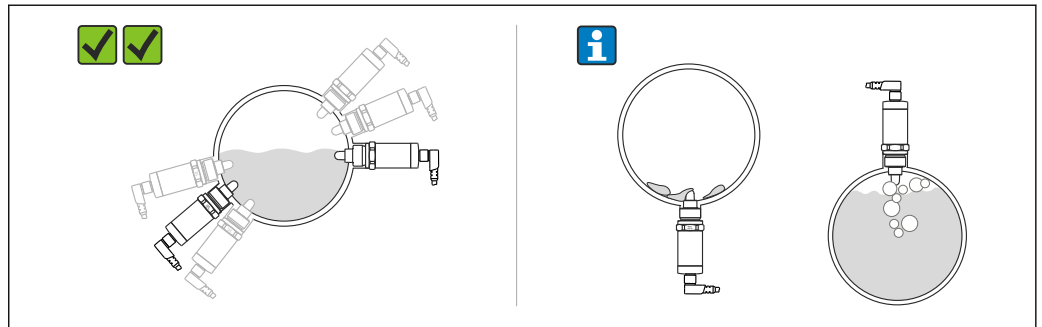
图 3 在水平管道中的安装位置
