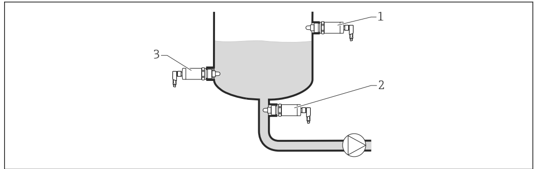
图 2 安装示意图
