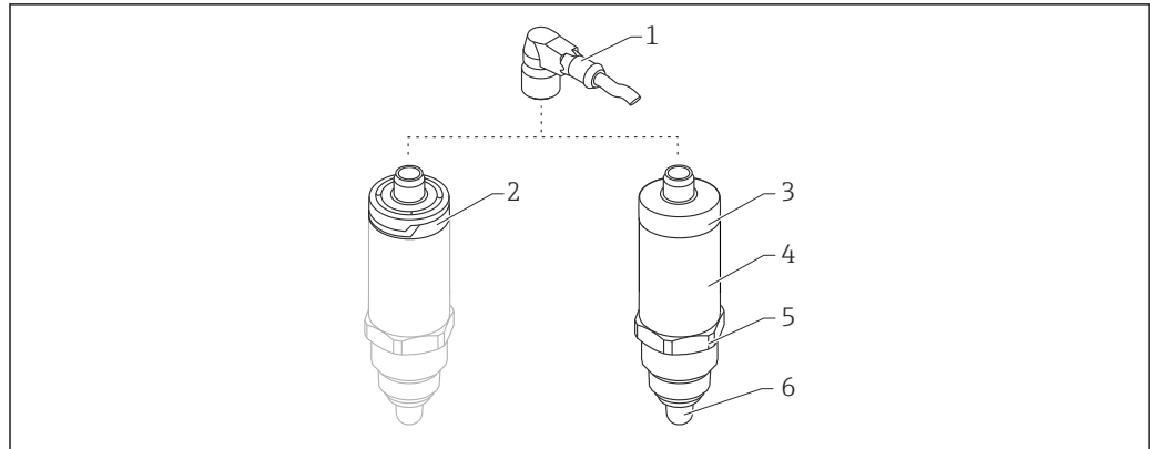
图 1 Liquipoint FTW23 的产品设计
